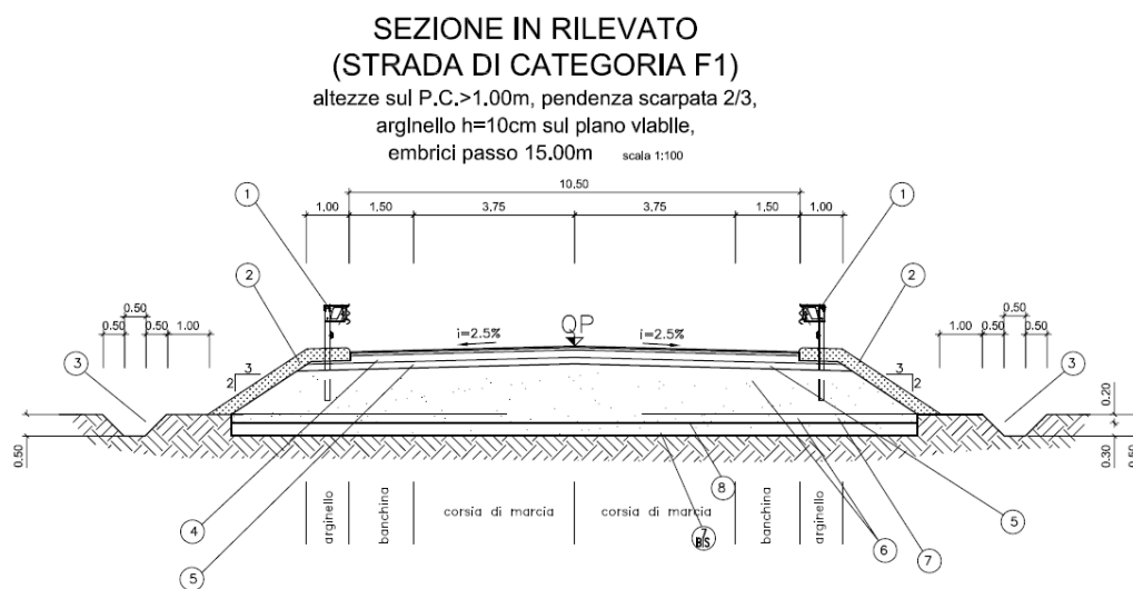
Figura 3 – sezione tipo in rilevato
