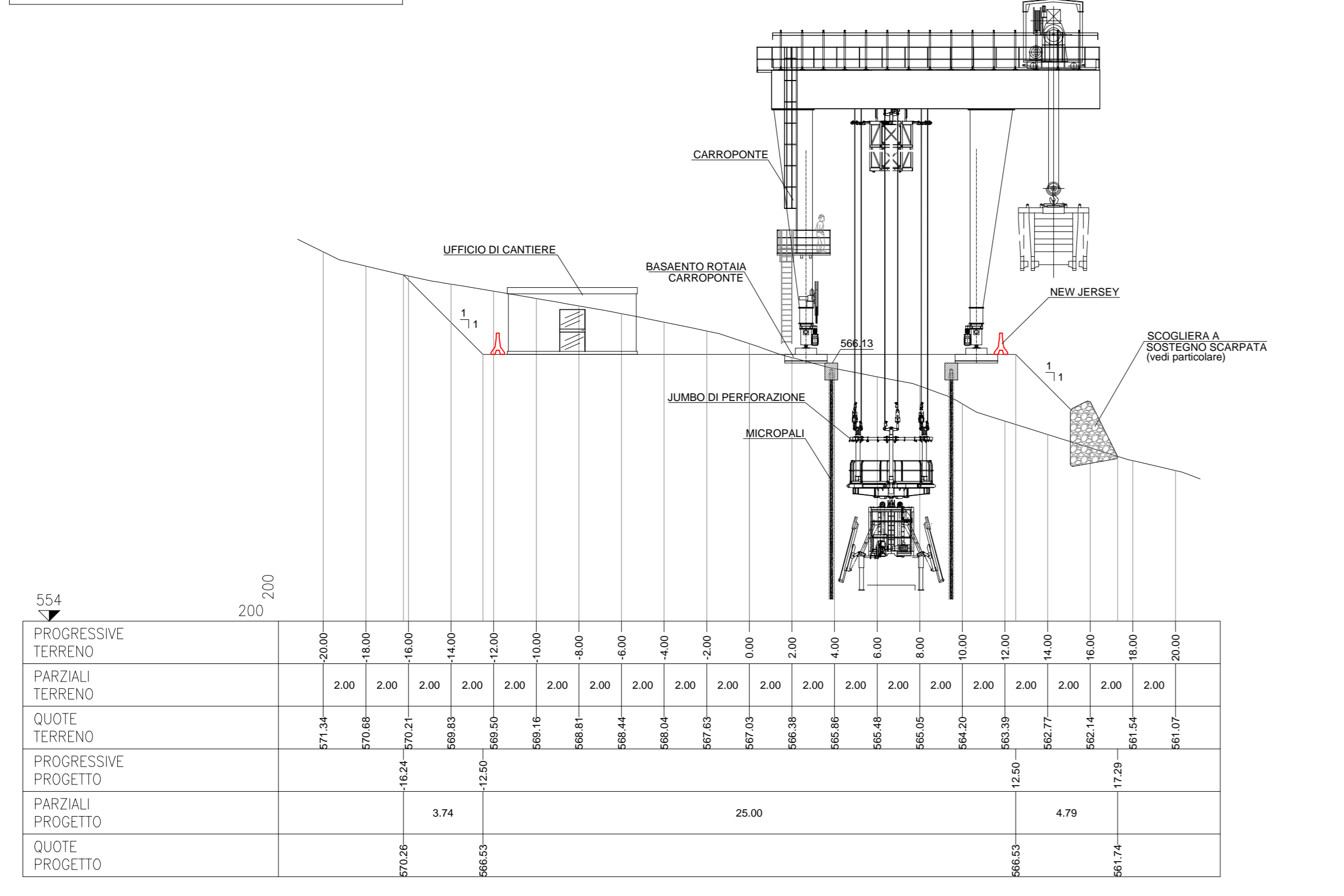
SEZIONE TRSVERSALE 1-1 SCALA 1:200
