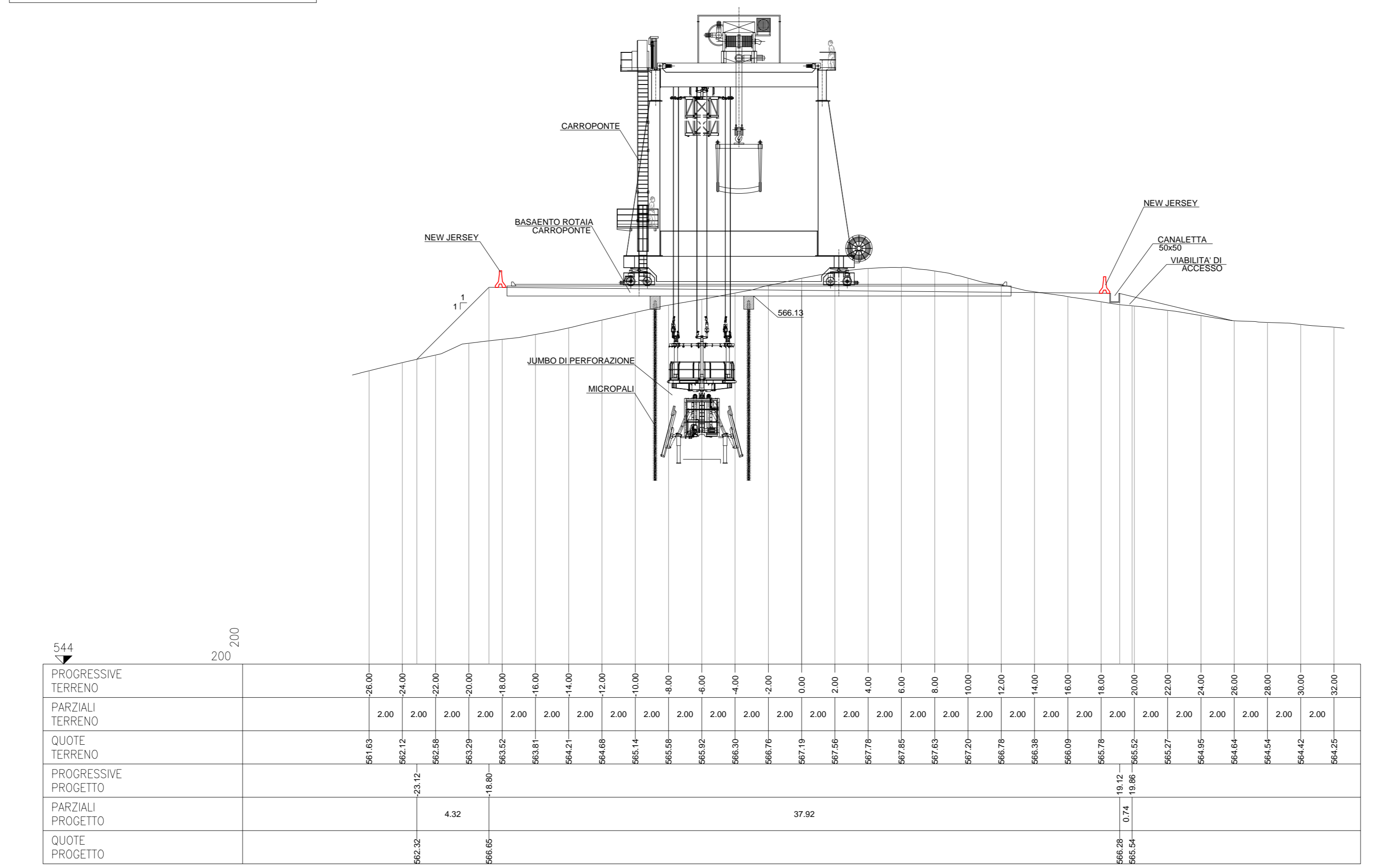
SEZIONE LONGITUDINALE 2-2 SCALA 1:200
