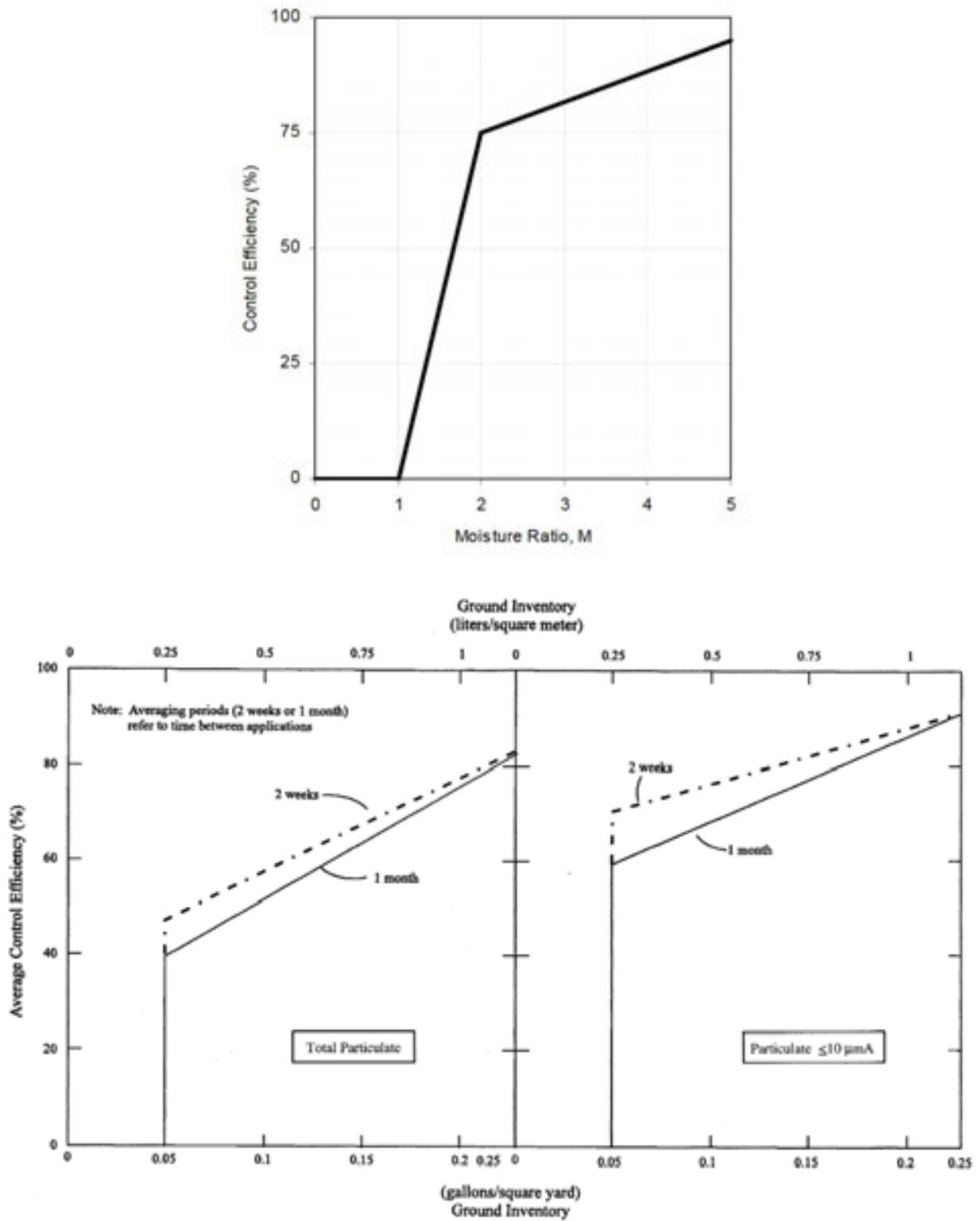
Figura 3-11 – Efficacia degli interventi di bagnatura sulle piste/aree non asfaltate (EPA - Emissions Factors & AP 42, Compilation of Air Pollutant Emission Factors, capitolo 13)
