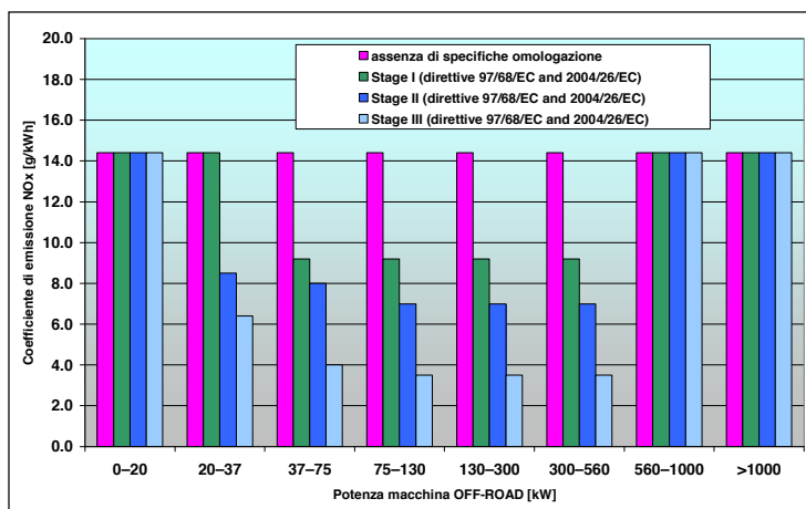
Figura 3-5 - Coefficienti di emissione NOx veicoli OFF-ROAD (fonte EMEP/EEA)
