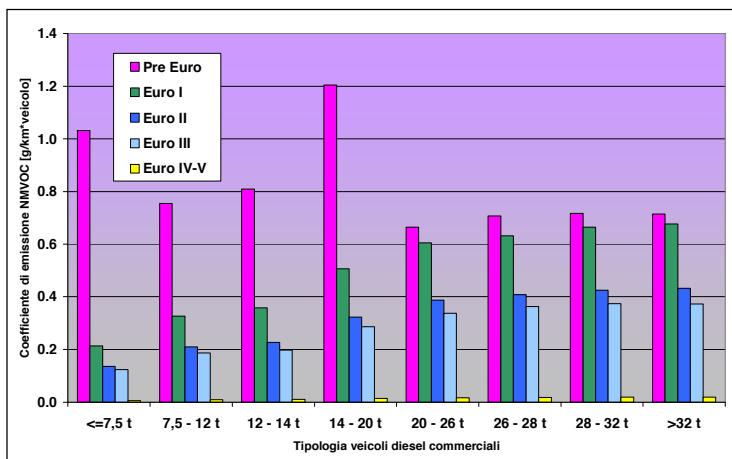
Figura 3-3 - Coefficienti di emissione NMVOC veicoli diesel comm. pesanti (Copert IV)
