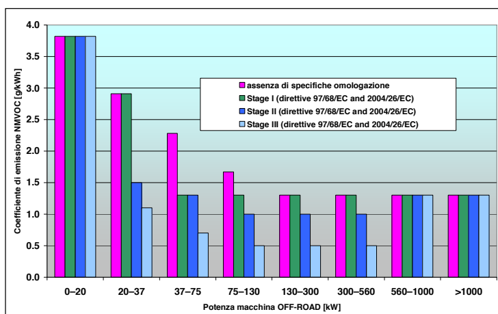
Figura 3-6 - Coefficienti di emissione NMVOC veicoli OFF-ROAD (fonte EMEP/EEA)
