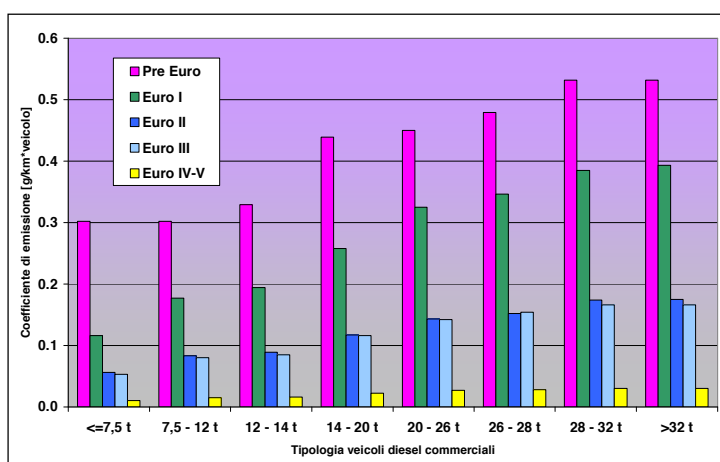
Figura 3-1 - Coefficienti di emissione Pm10 veicoli diesel commerciali pesanti (Copert IV)
