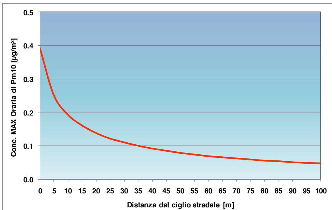
Figura 3-14 – Andamento delle concentrazioni massime di Pm10
