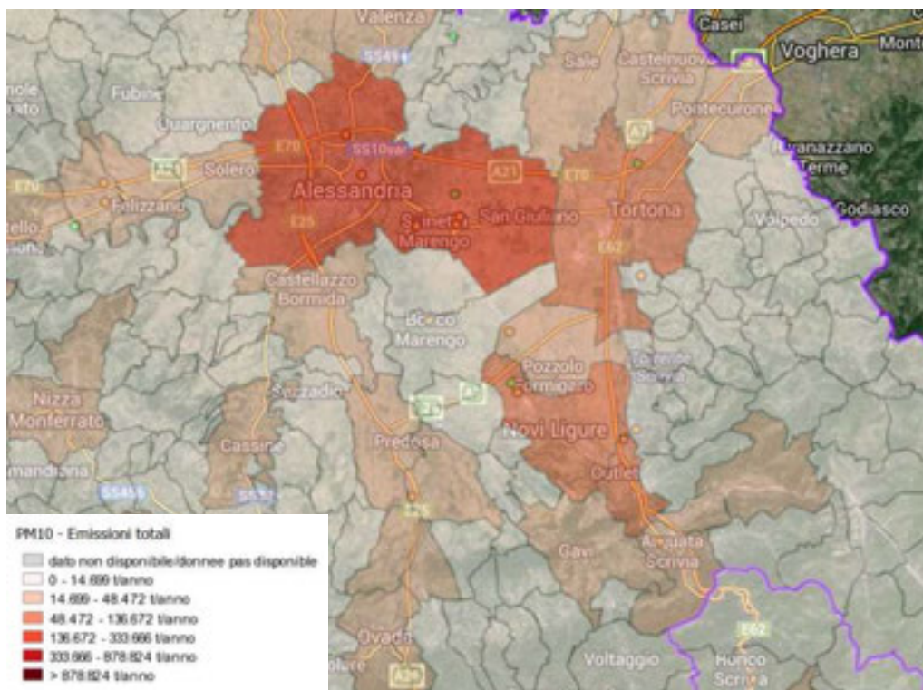
Figura 2.32 – Emissioni Totali Pm10 Provincia di Alessandria – IREA 2008
