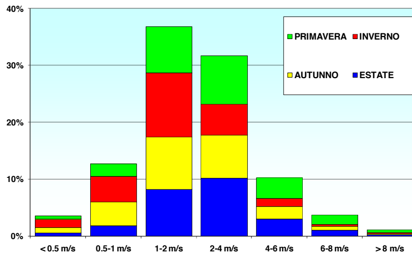
Figura 2.17 – Velocità del vento: Punto 22680
