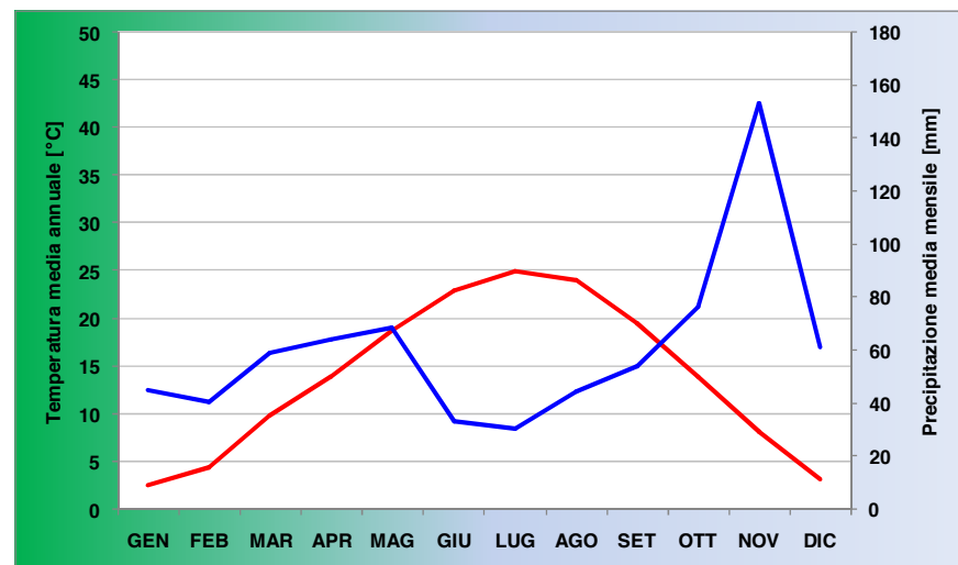
Figura 2.9 – Diagramma di Walter e Lieth – Stazione di Novi Ligure
