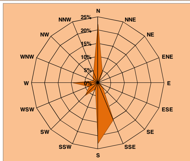
Figura 2.10 – Caratteristiche Anemologiche - Stazione di Novi Ligure
