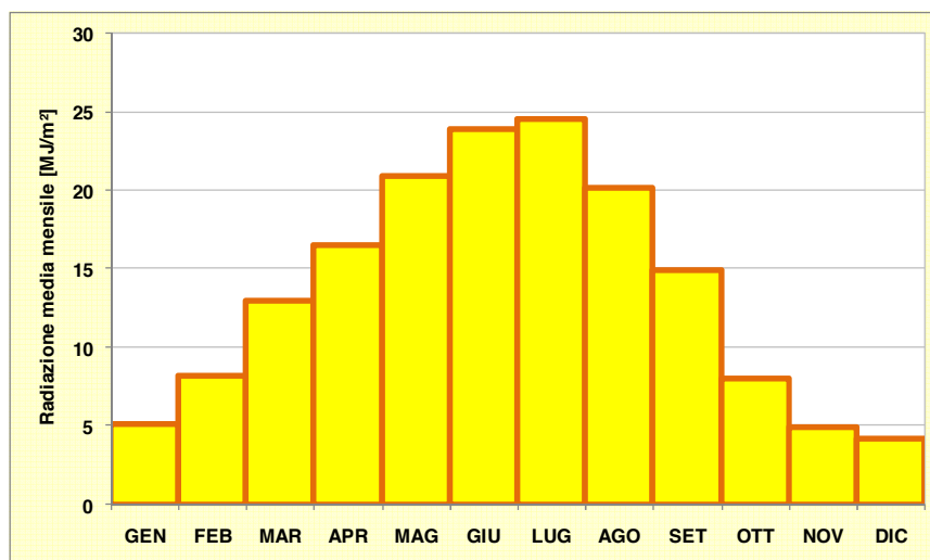
Figura 2.11 – Radiazione solare - Stazione di Novi Ligure
