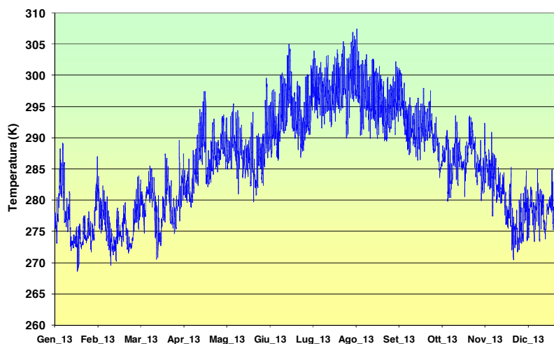
Figura 2.13 – Andamento delle temperature orarie: Punto 22680
