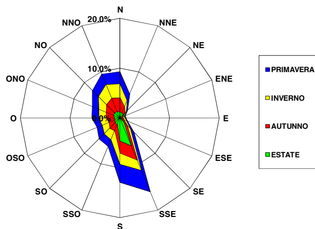
Figura 2.16 – Direzione del vento: Punto 22680
