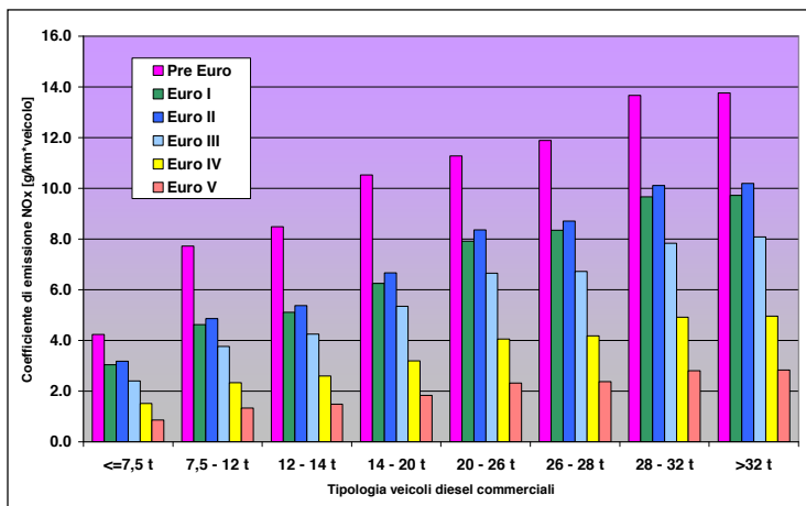
Figura 3-2 - Coefficienti di emissione NOx veicoli diesel commerciali pesanti (Copert IV)
