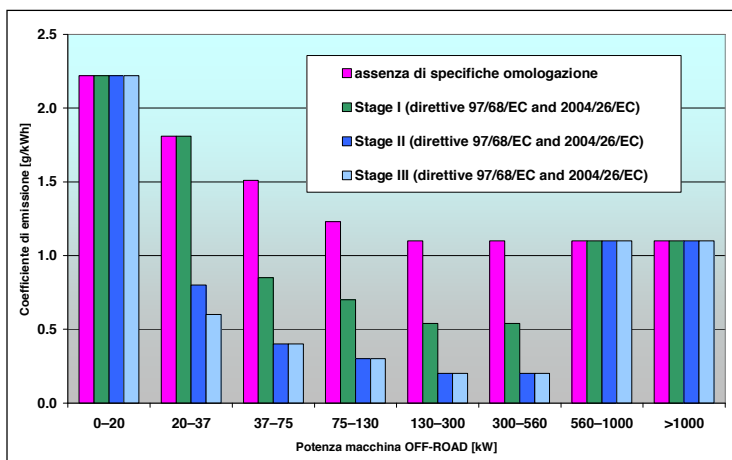
Figura 3-4 - Coefficienti di emissione Pm10 veicoli OFF-ROAD (fonte EMEP/EEA)
