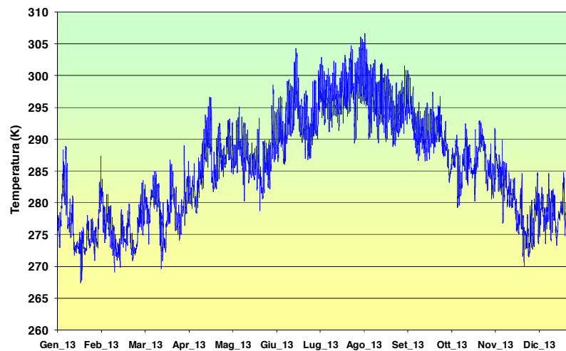
Figura 2.18 – Andamento delle temperature orarie: Punto 22681
