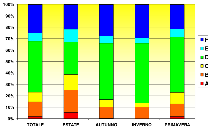
Figura 2.19 – Classi di stabilità: Punto 22681
