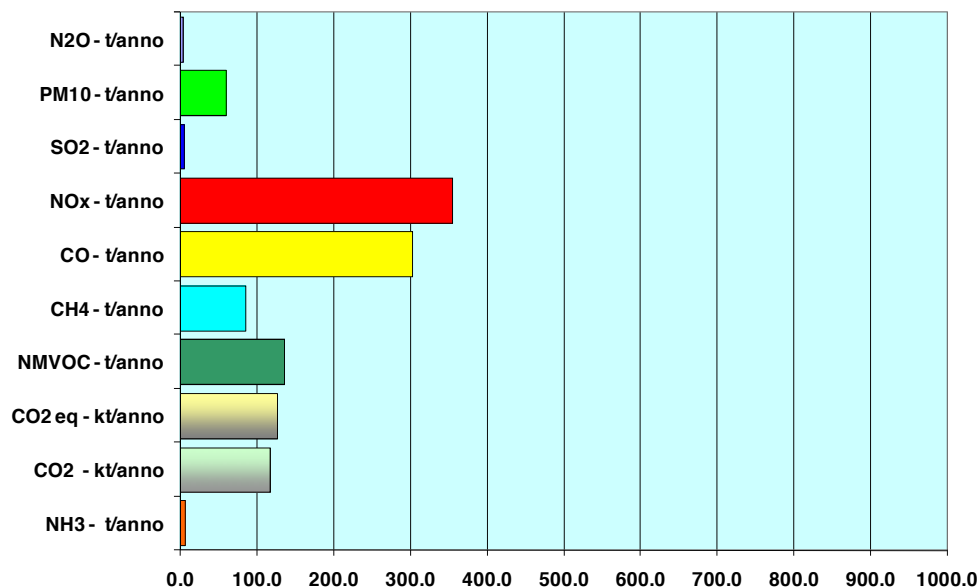
Figura 2.29 – Emissioni Comune di Serravalle Scrivia – IREA 2008
