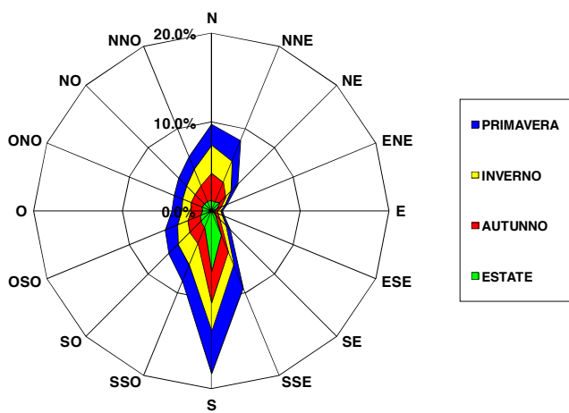
Figura 2.26 – Direzione del vento: Punto 22849
