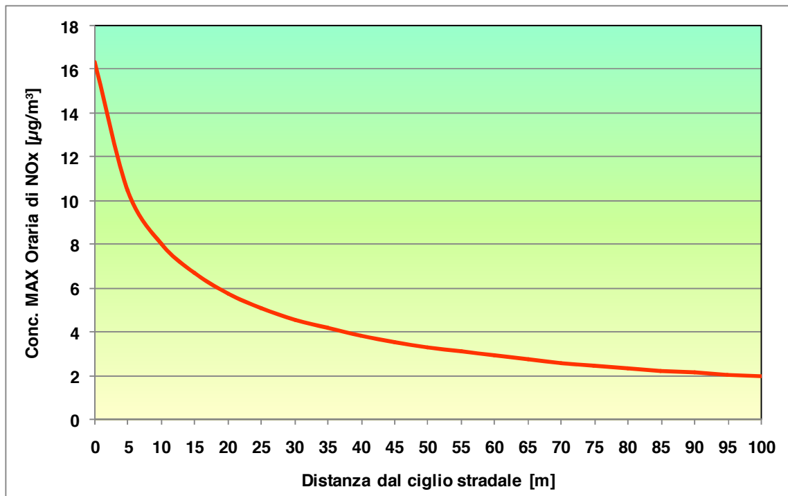
Figura 3-13 – Andamento delle concentrazioni massime di NOx
