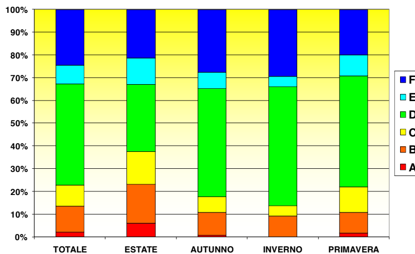
Figura 2.24 – Classi di stabilità: Punto 22849
