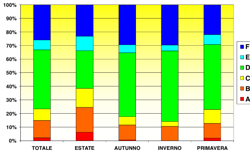
Figura 2.14 – Classi di stabilità: Punto 22680
