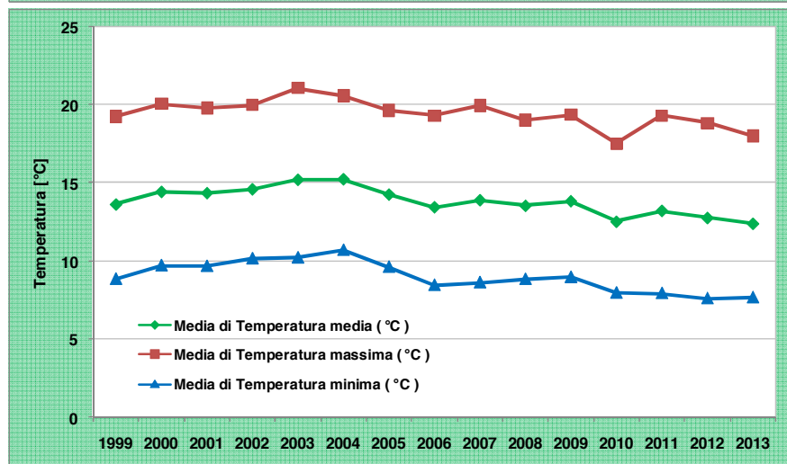
Figura 2.7 – Caratteristiche Termiche - Stazione di Novi Ligure
