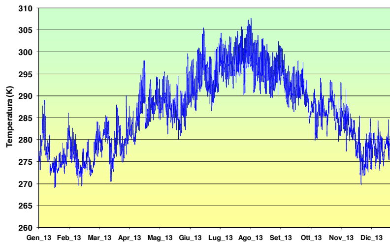
Figura 2.23 – Andamento delle temperature orarie Punto 22849
