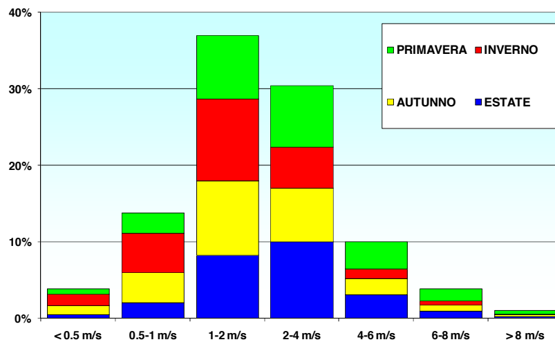
Figura 2.22 – Velocità del vento: Punto 22681
