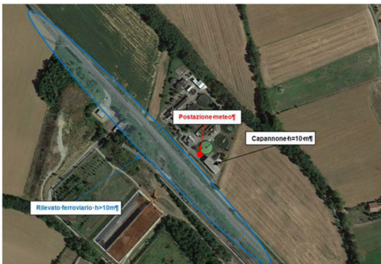
Figura 2.4 – Ubicazione stazione meteo di Novi Ligure
