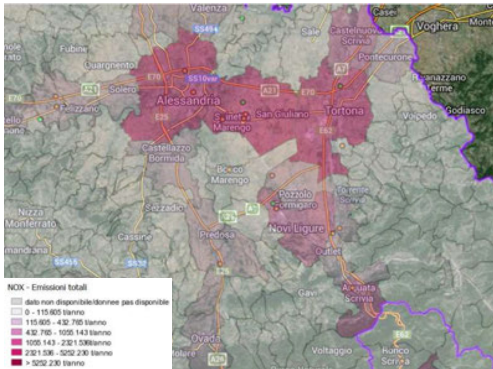
Figura 2.31 – Emissioni Totali NOx Provincia di Alessandria – IREA 2008
