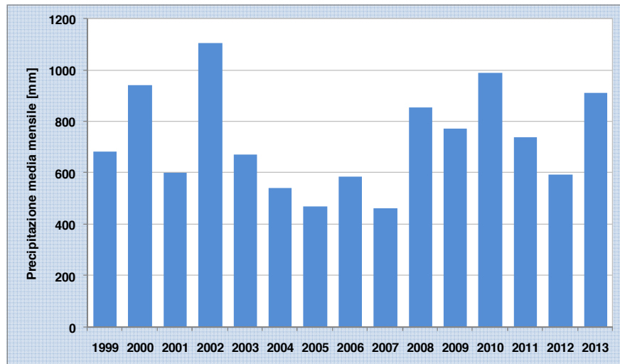
Figura 2.8 – Caratteristiche Pluviometriche - Stazione di Novi Ligure
