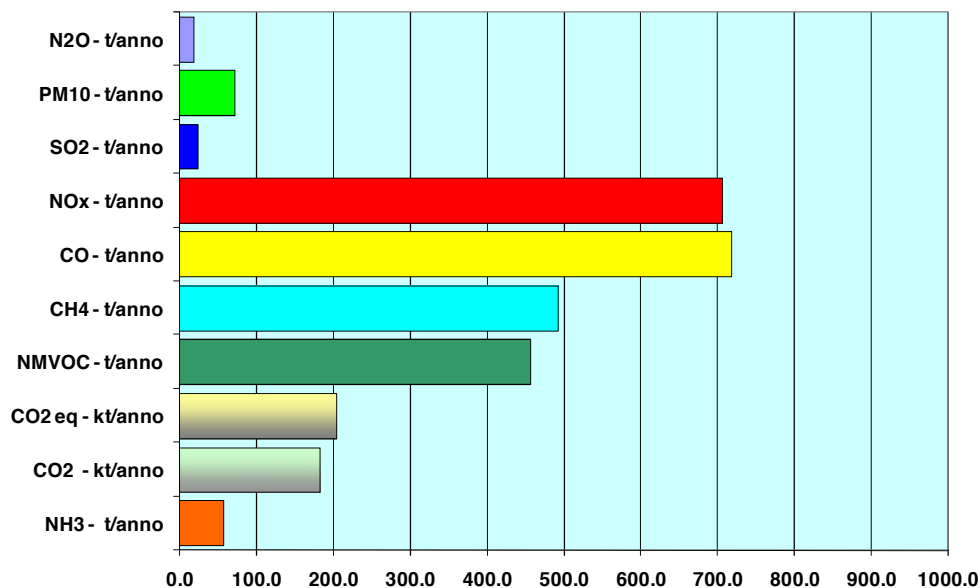
Figura 2.28 – Emissioni Comune di Novi Ligure – IREA 2008
