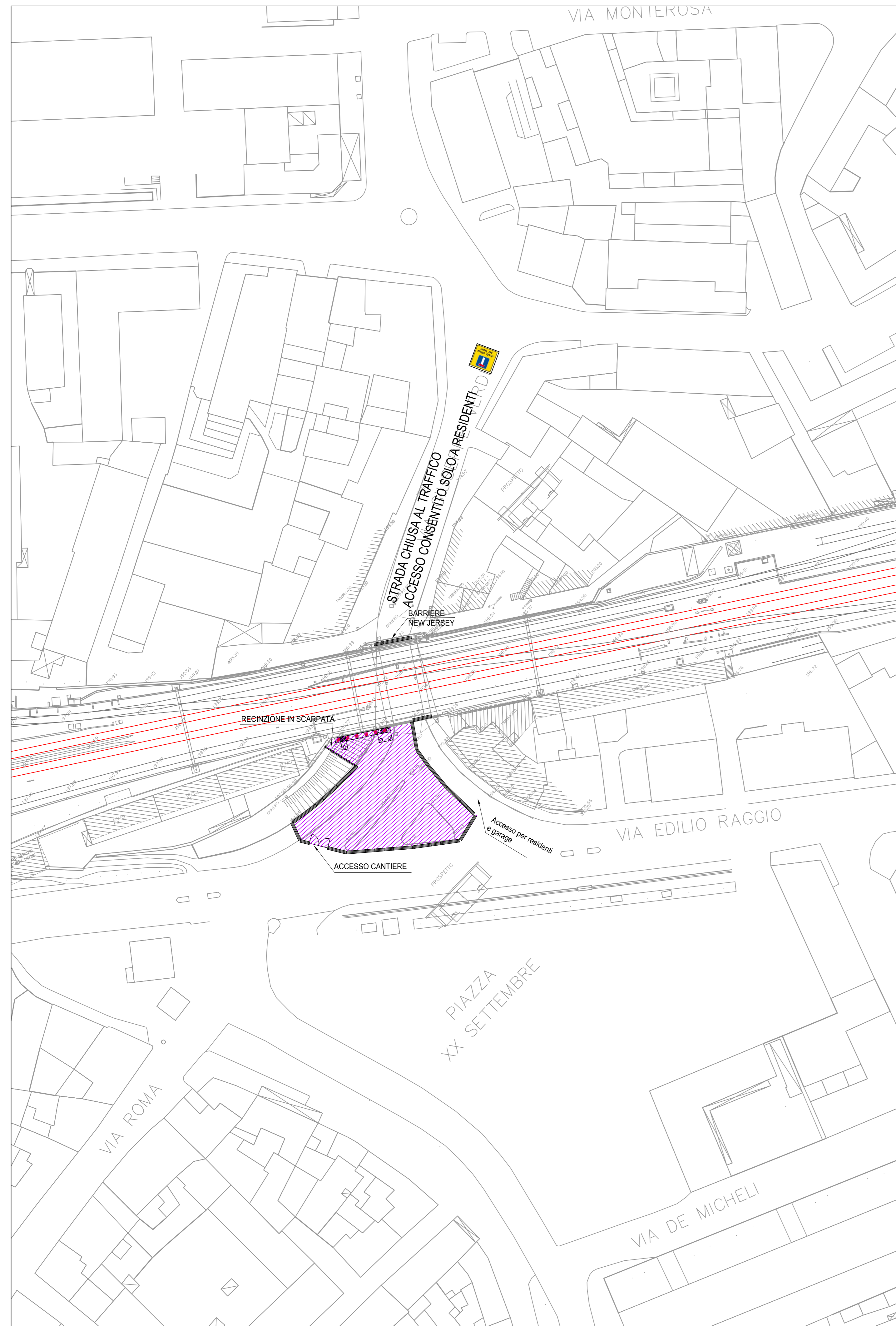
AREA DI CANTIERIZZAZIONE 5: 1° FASE Scala: 1:500
