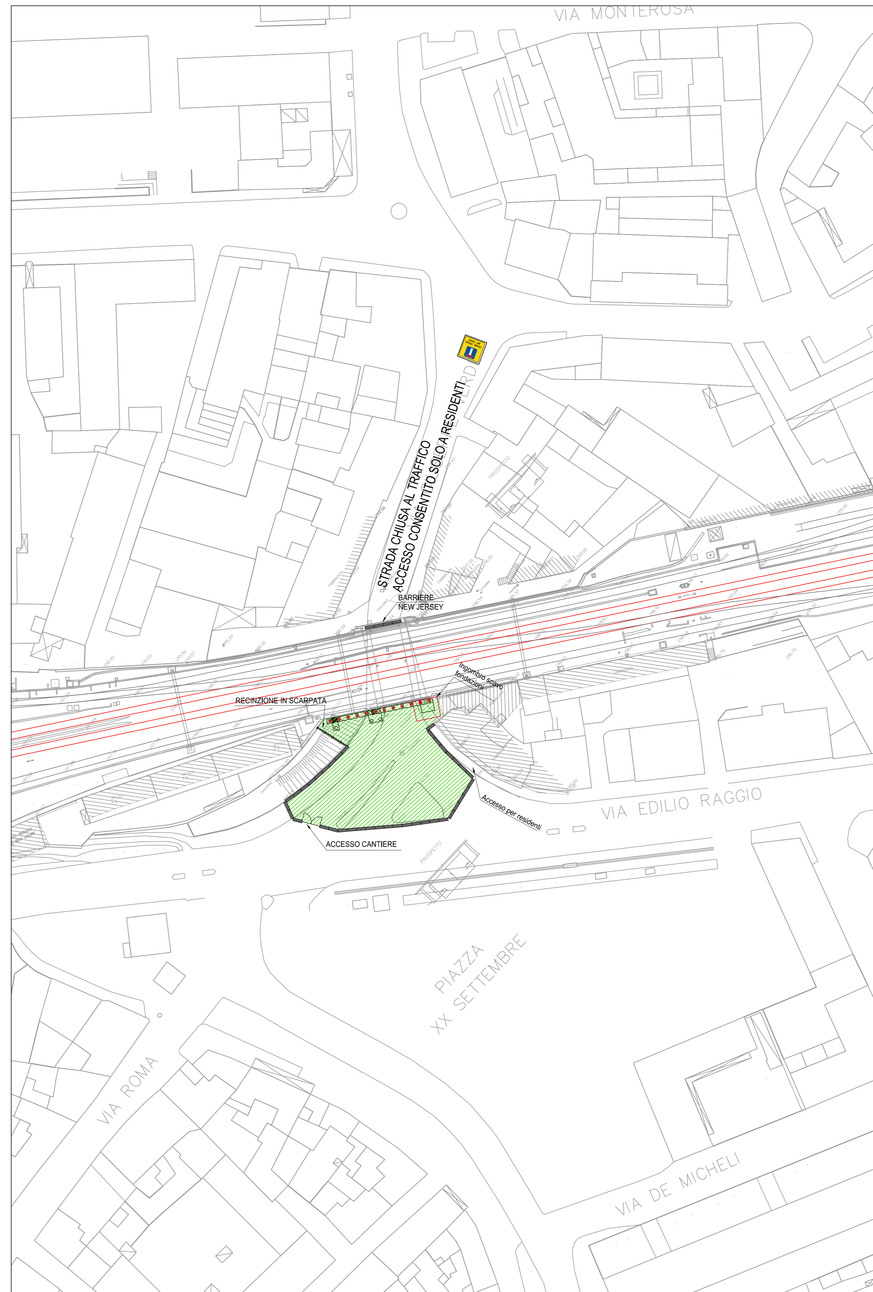
AREA DI CANTIERIZZAZIONE 5: 2° FASE Scala: 1:500
