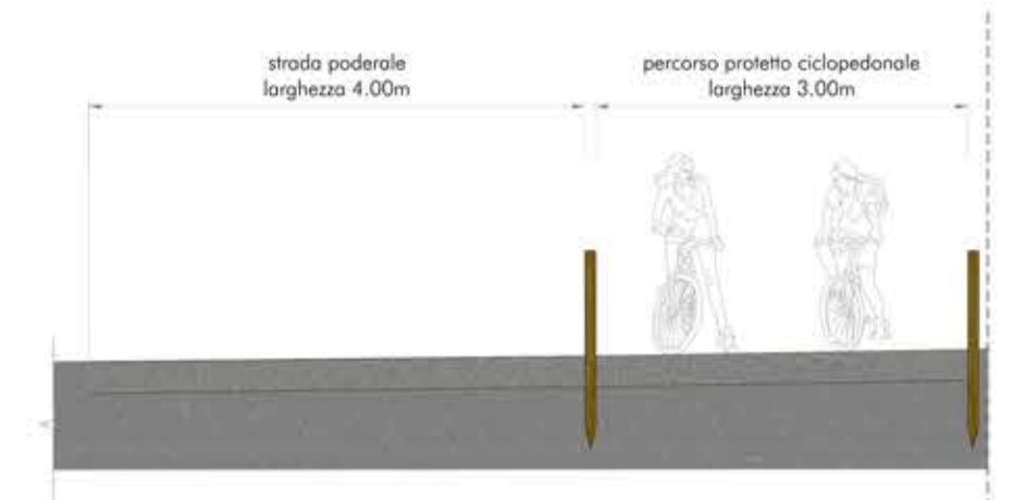
Percorso promiscuo protetto di mobilità dolce ciclopedonale
