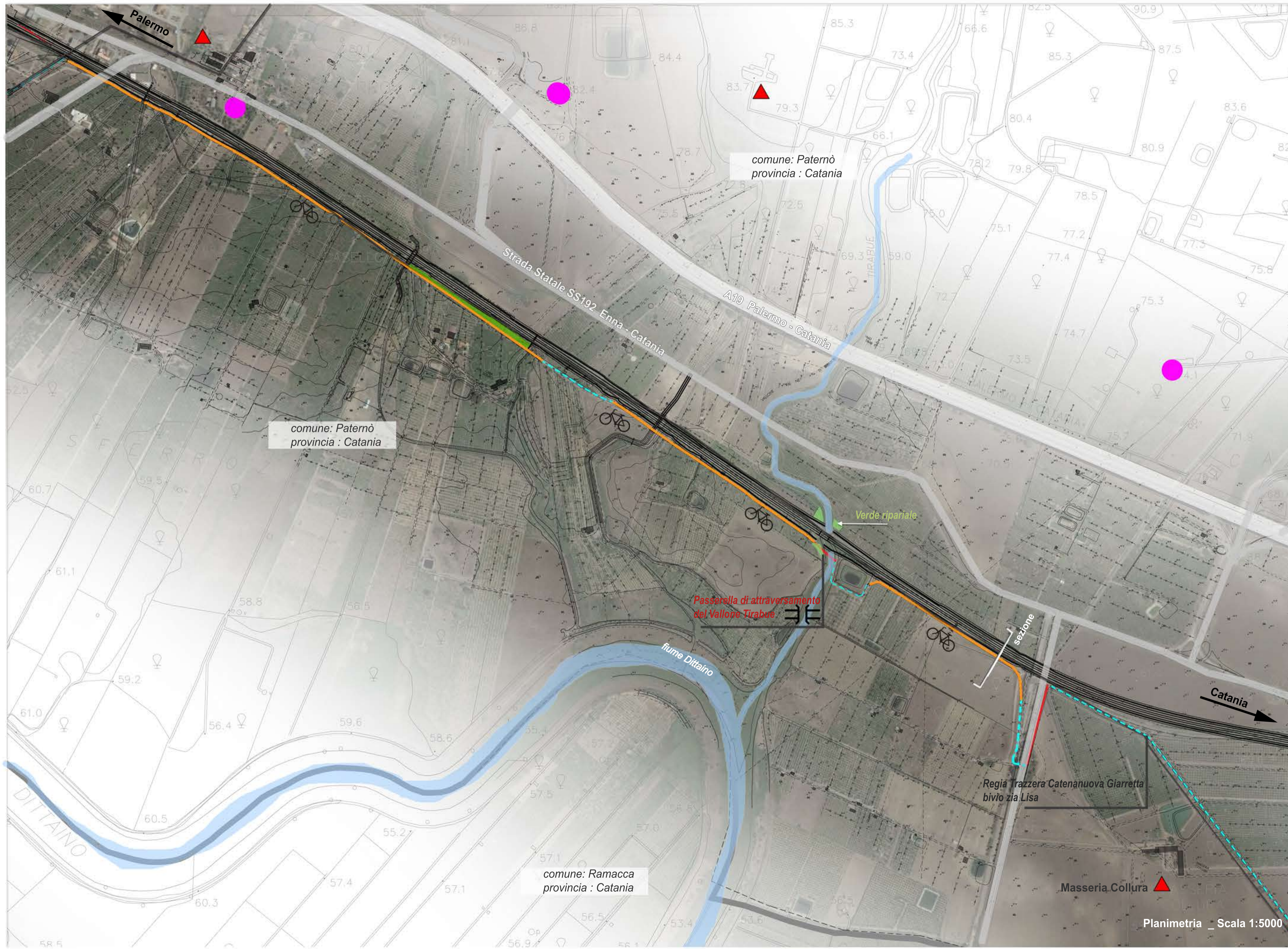
Percorso promiscuo protetto di mobilità dolce ciclopedonale
