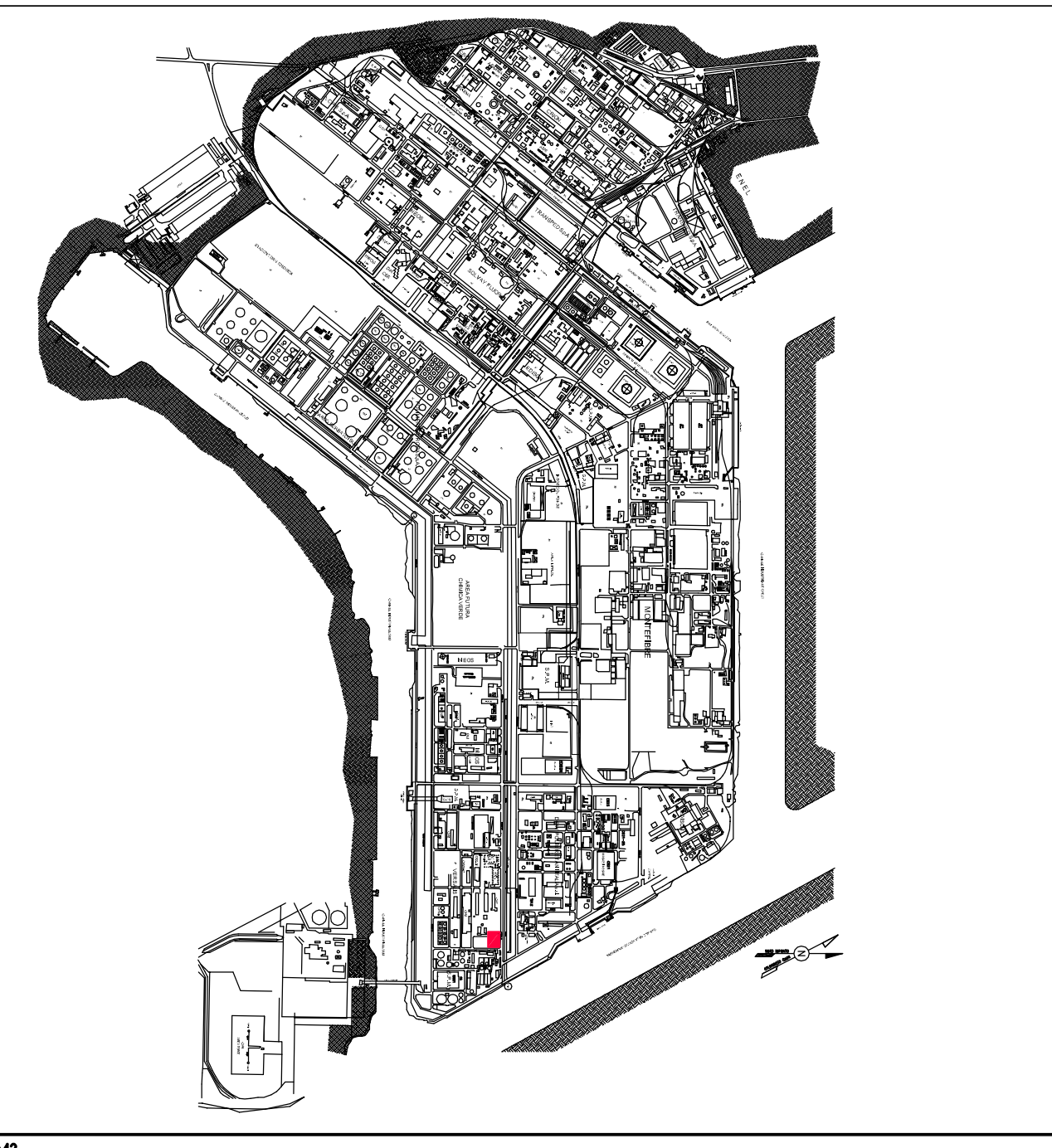
KEY-PLAN
