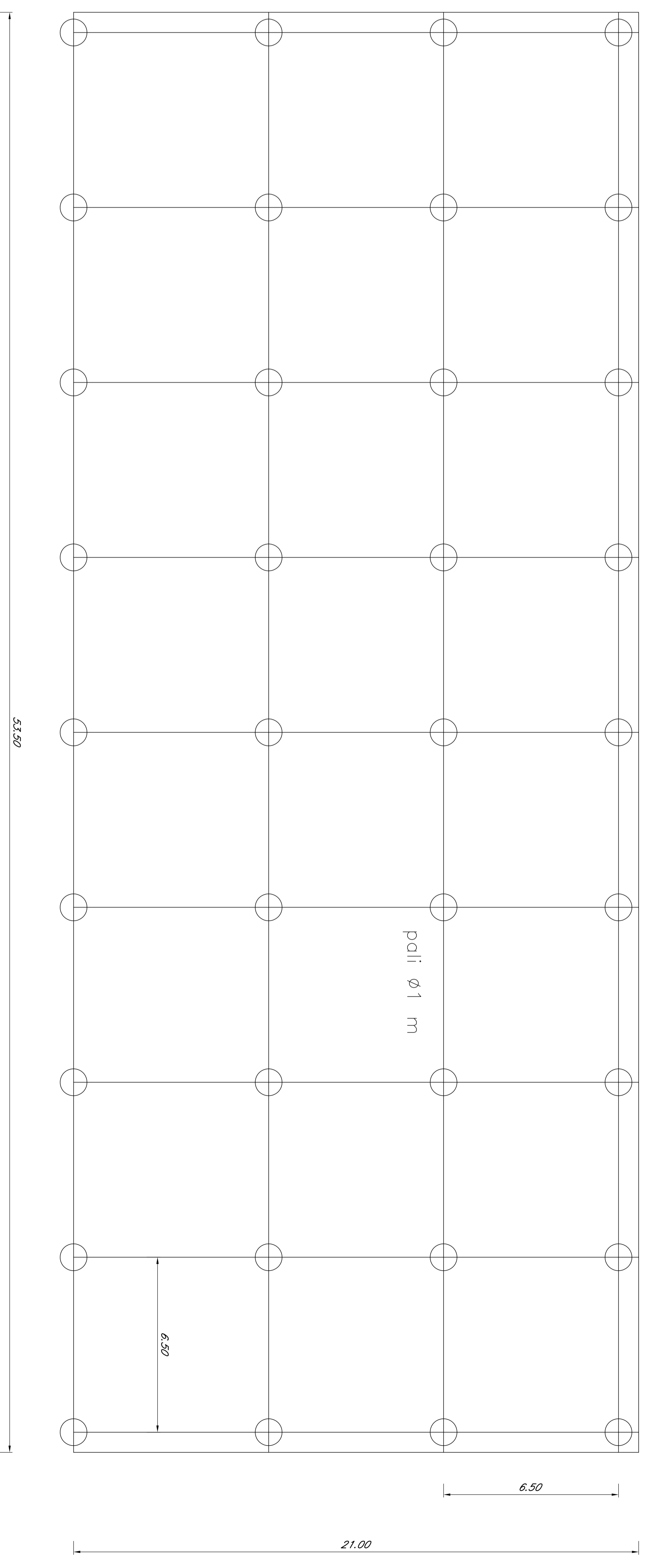
PIANTA STRUTTURALE BANCHINA DI ATTRACCO
