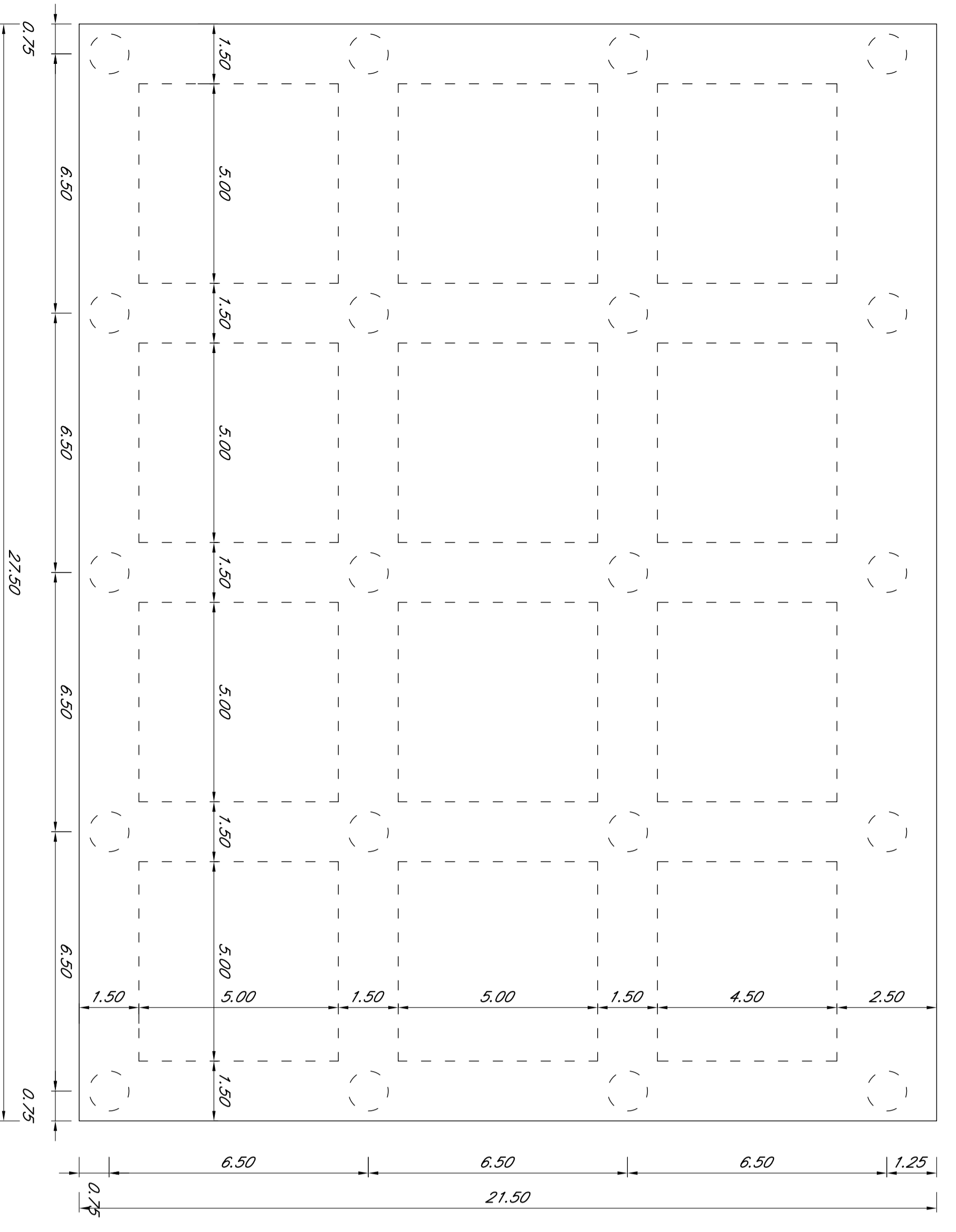
PIANTA STRUTTURALE BANCHINA DI ATTRACCO
