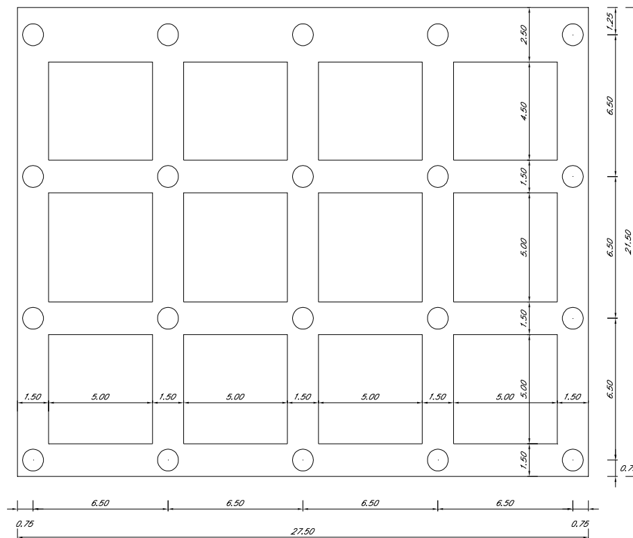
Figura 14 - Molo d'attracco della Società Diano. Pianta
