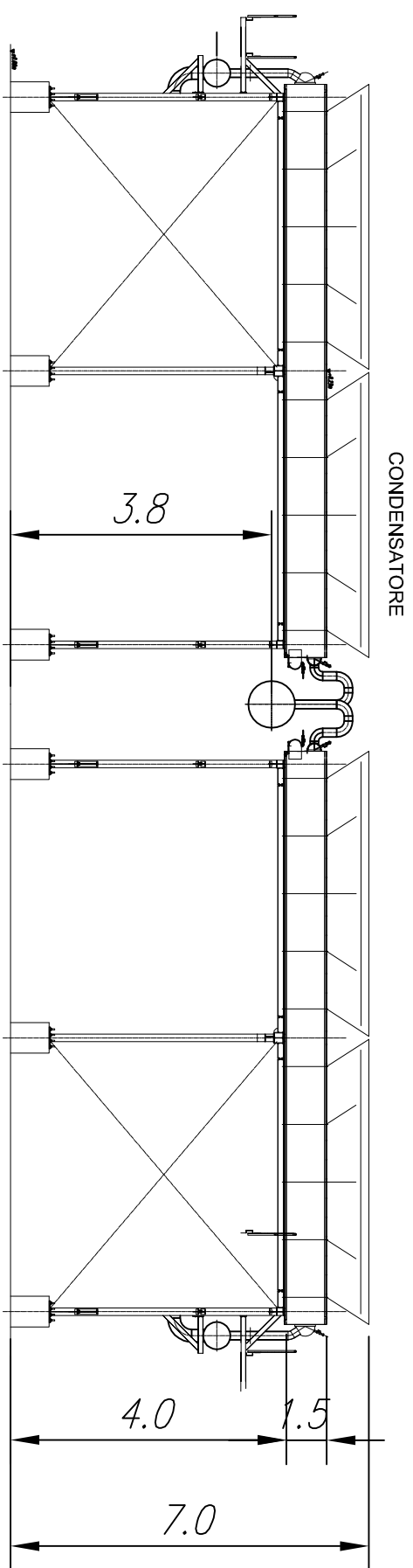
VISTA A-A
