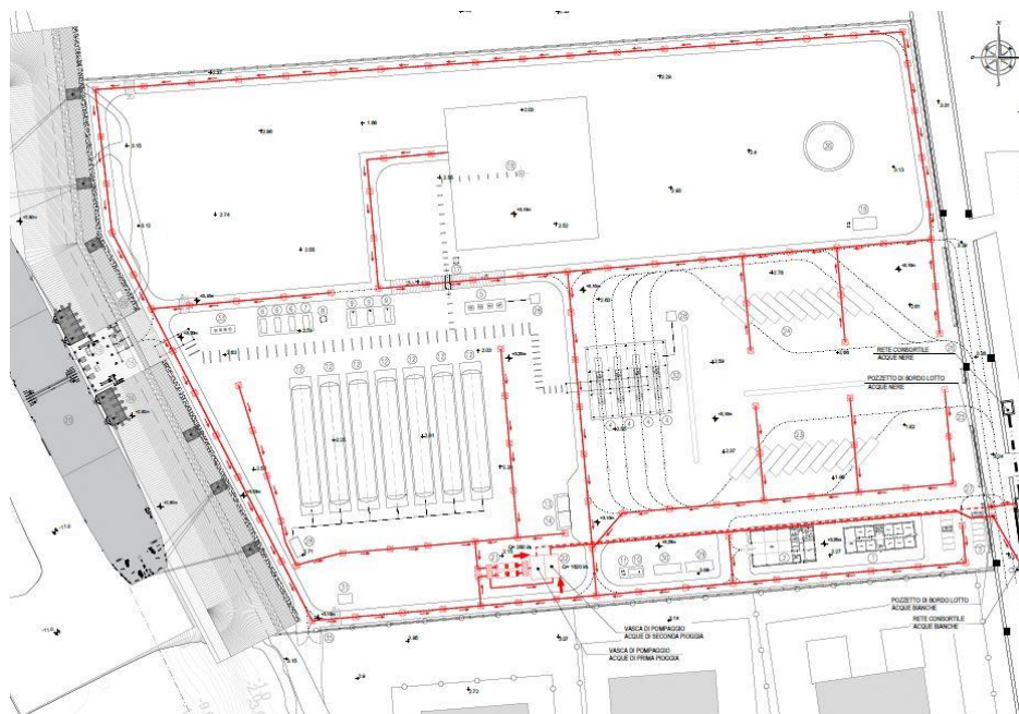
Figura 3.3: Planimetria rete di smaltimento acque meteoriche
