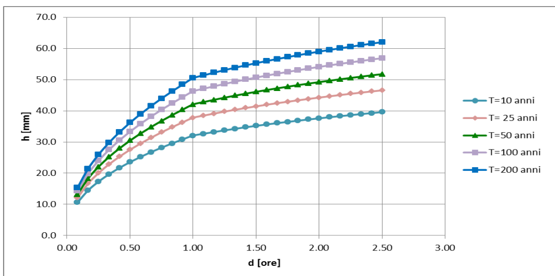
Figura 2.1: Curve di probabilità pluviometrica
