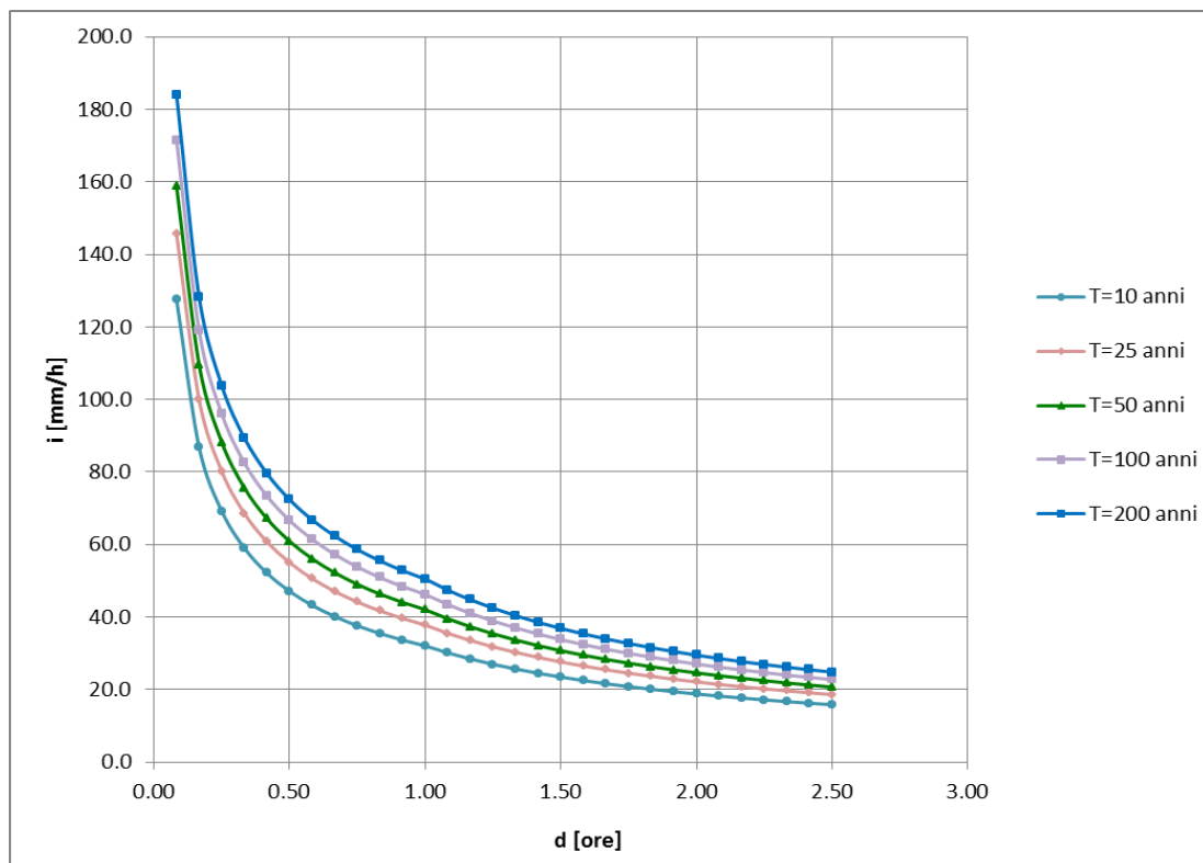
Figura 2.2: Curve intensità-durata-frequenza (IDF)
