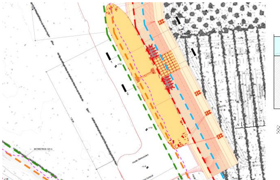
Figura 1.1: Opera a Mare e Posizione della Gasiera all'Ormeggio
