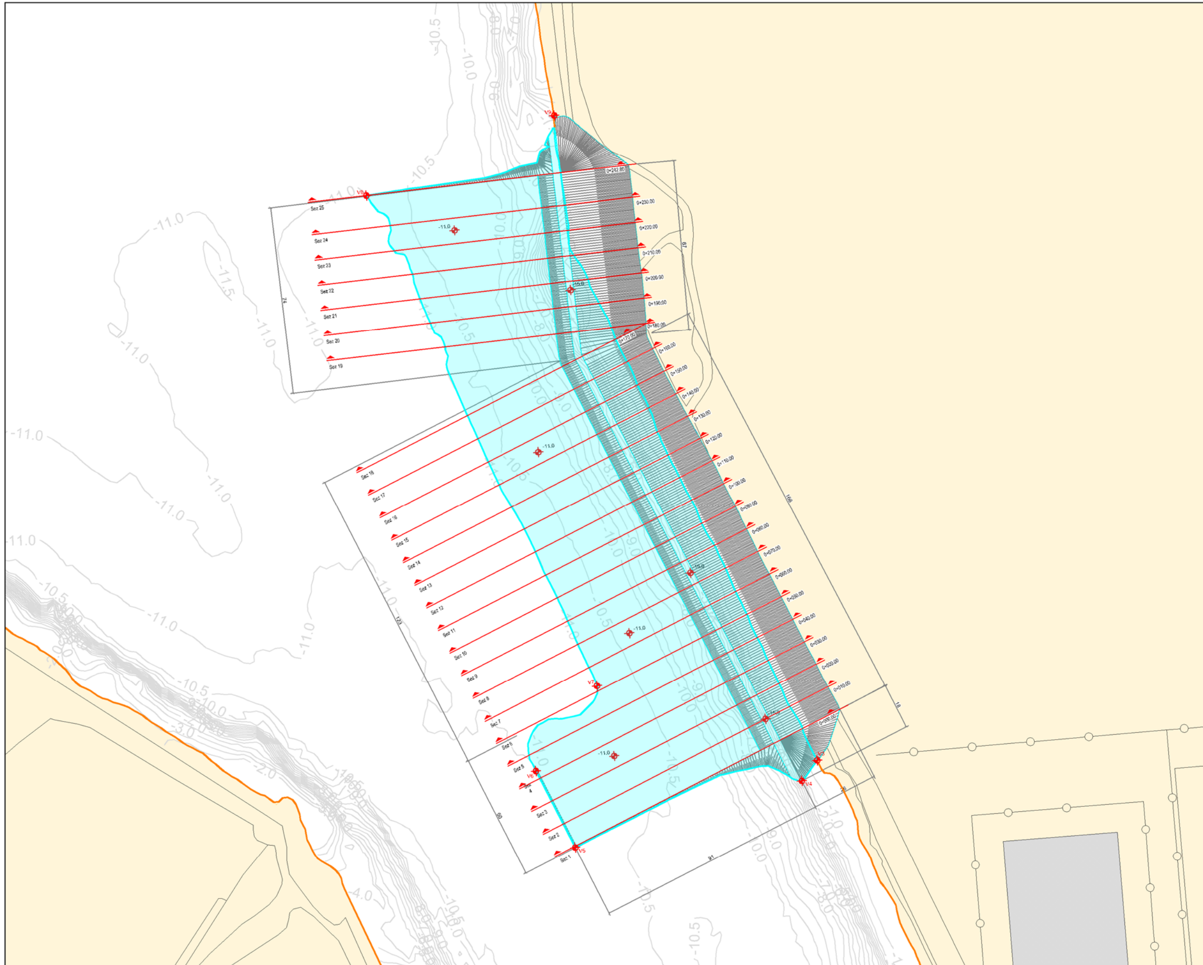
FIGURA 3.4a PLANIMETRIA DRAGAGGIO
