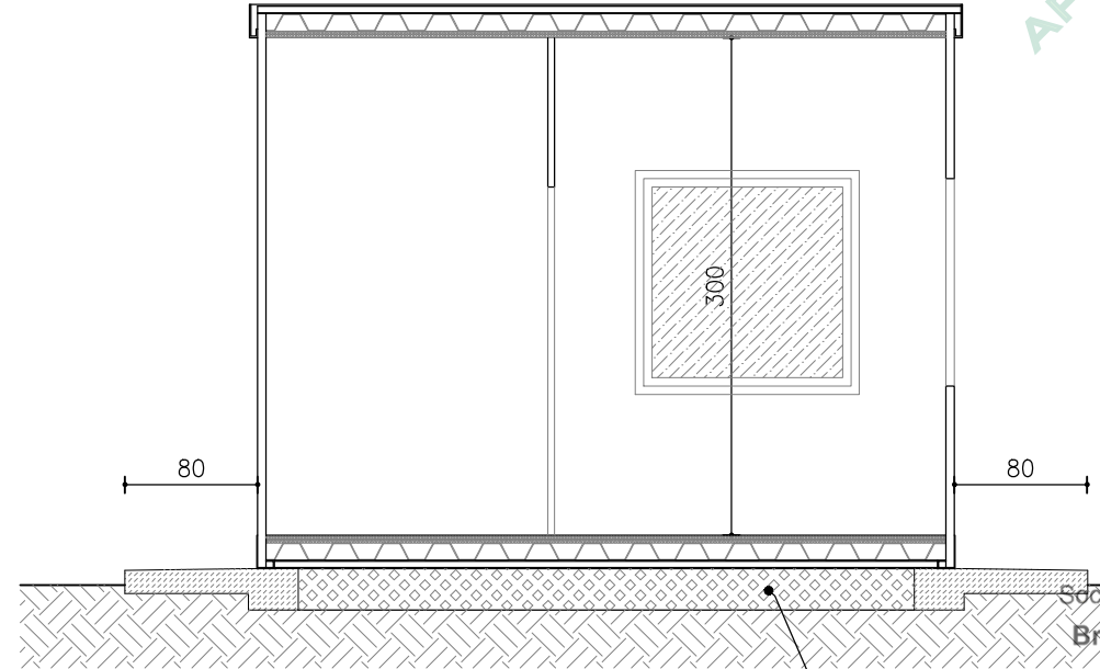
SEZIONE E-E 1:50
