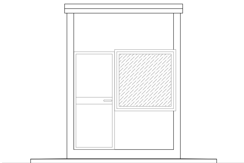
PROSPETTO "C" 1:50
