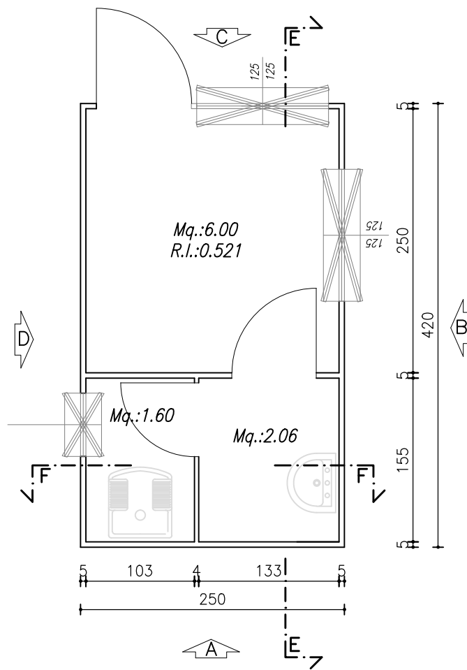
PIANTA GUARDIOLA "1" 1:50
