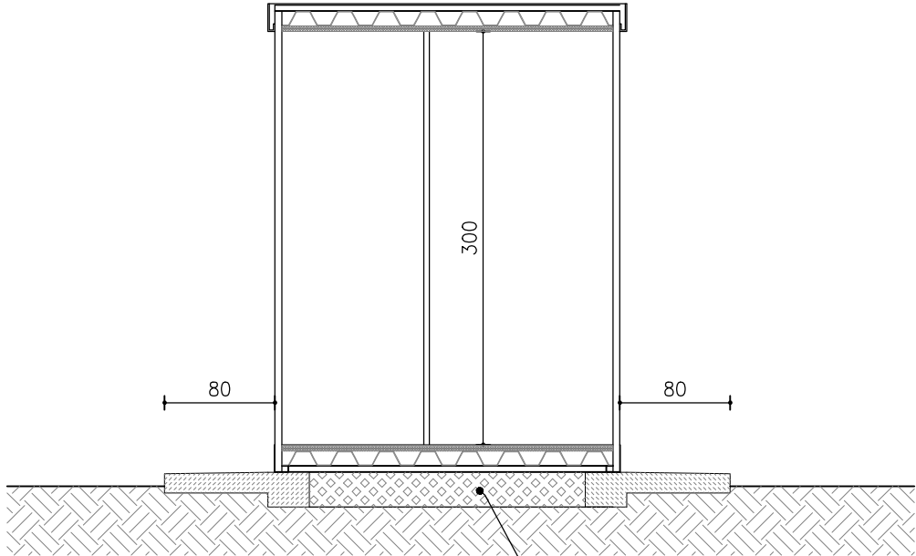
SEZIONE F-F 1:50
