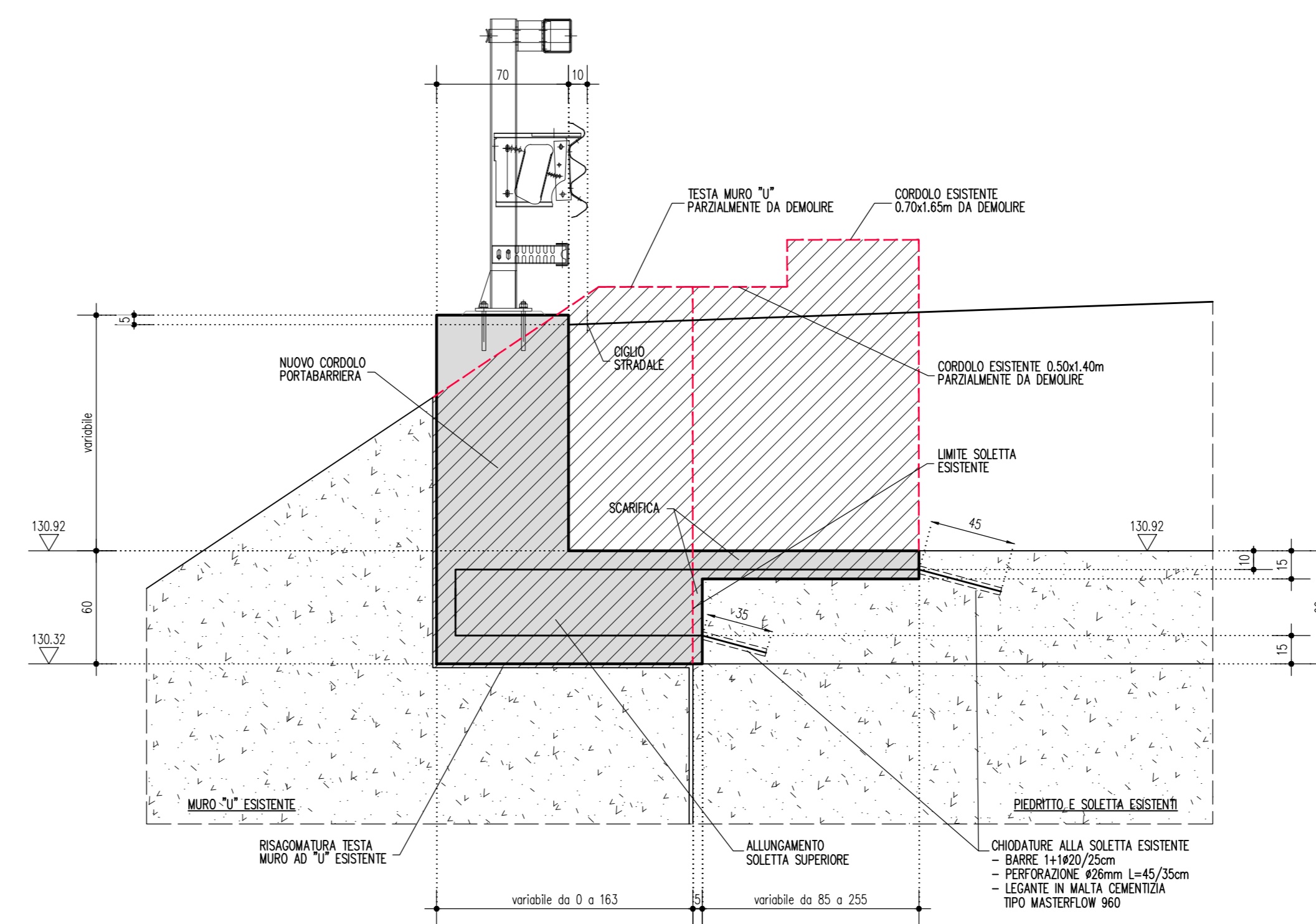
CORDOLO -1- ALLUNGAMENTO SOLETTA ESISTENTE 1:25
