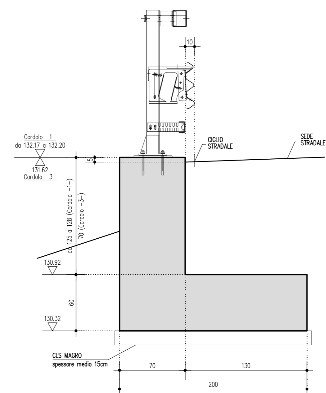
CORDOLI -1- / -3- MURTO AD "L" - SEZIONE TRASVERSALE 1:25
