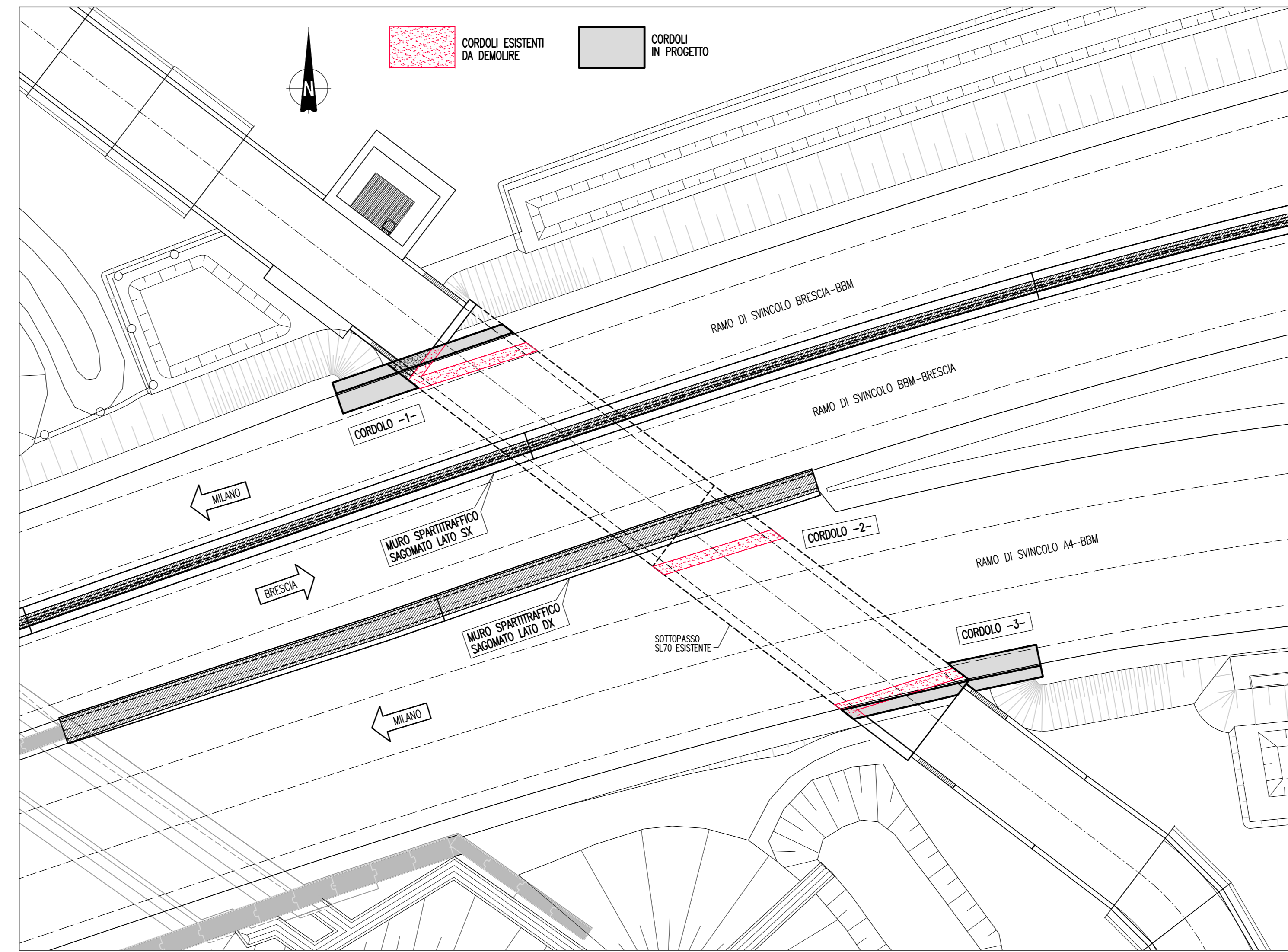
PIANTA CHIAVE 1:200
