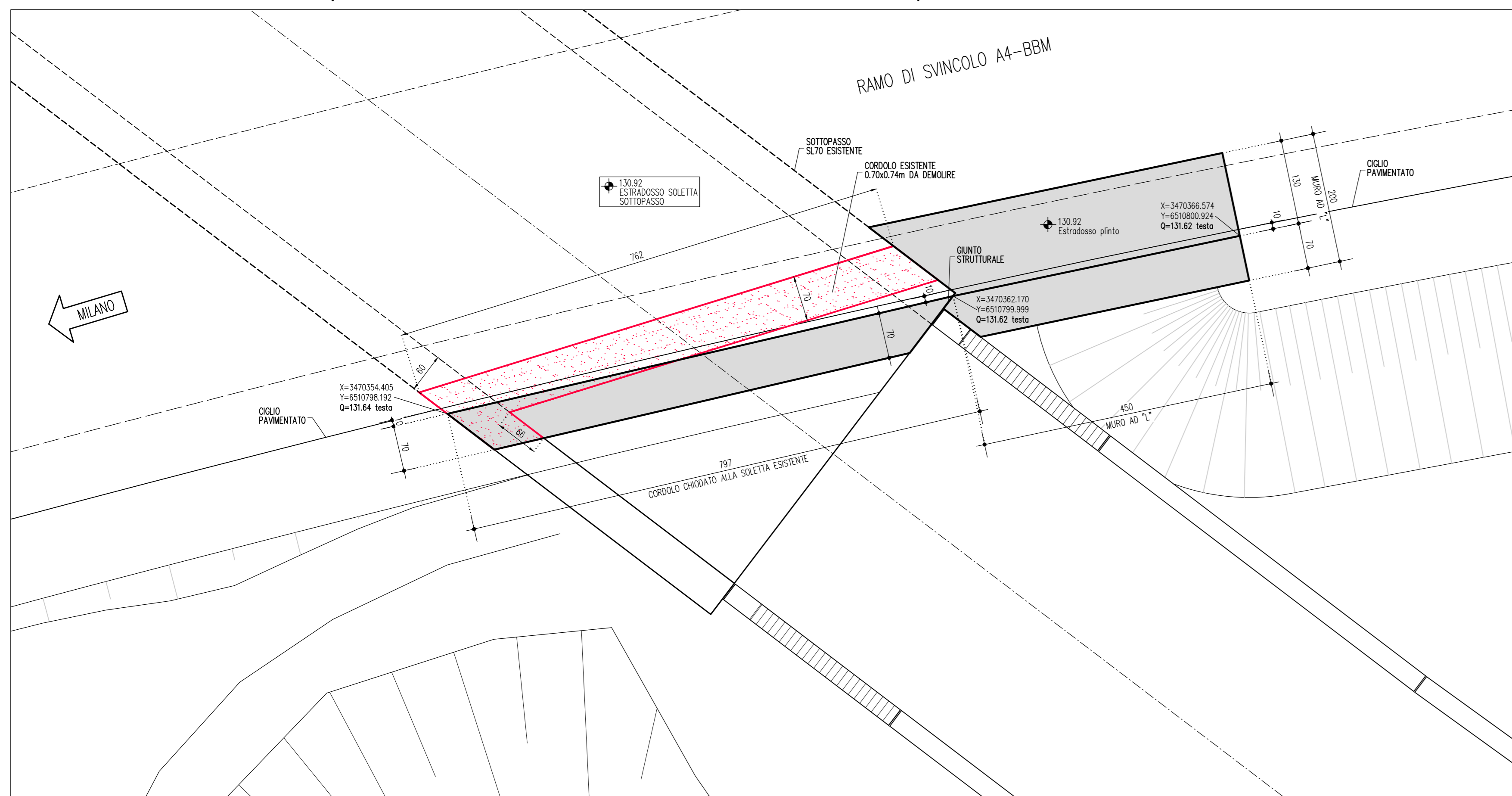
PIANTA CORDOLO -3- (demolizione cordolo esistente, chiodatura nuovo cordolo al sottopasso esistente, nuovo muro ad "L" 1:50
