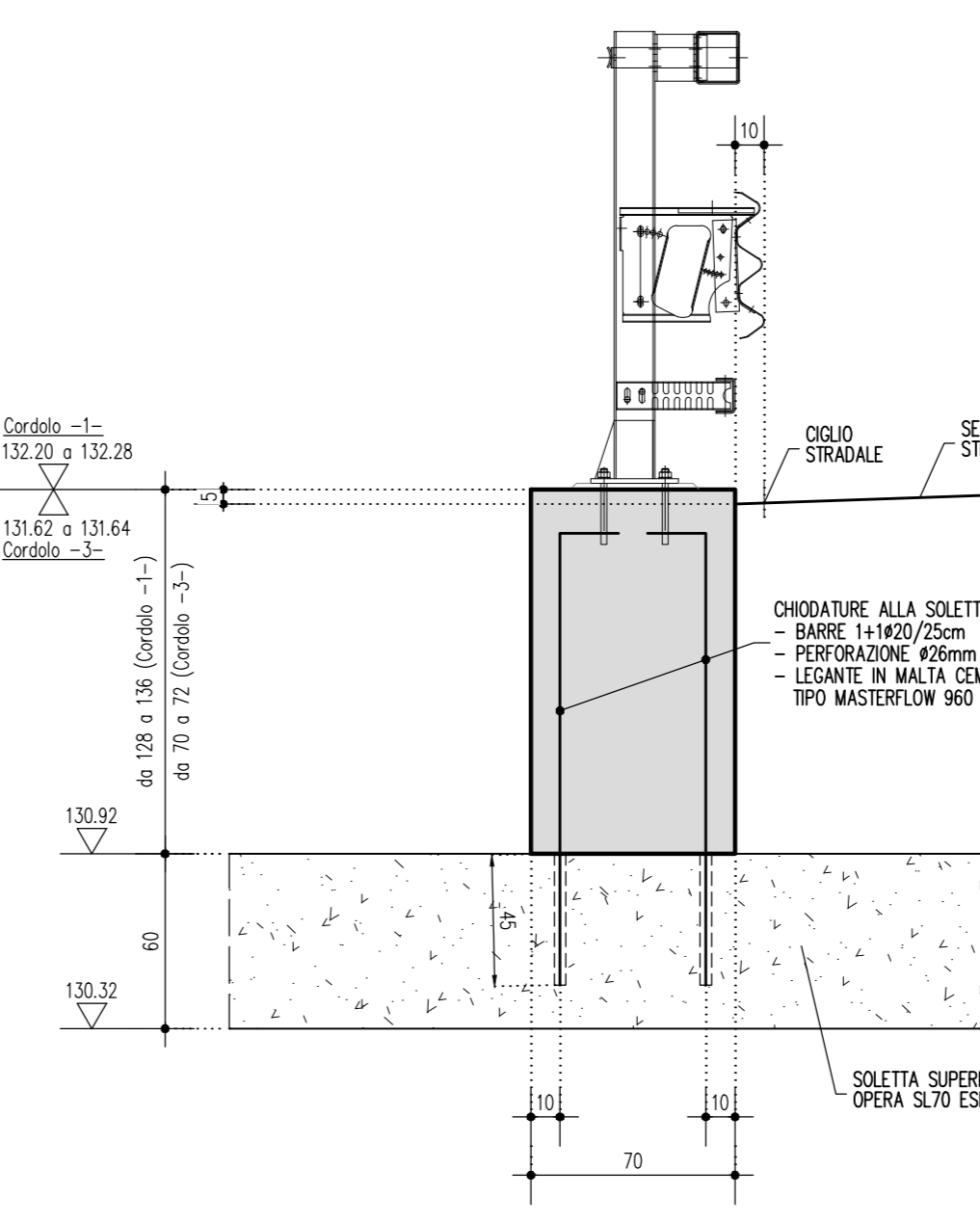
CORDOLI -1- / -3- CHIODATURA ALLA SOLETTA ESISTENTE 1:25
