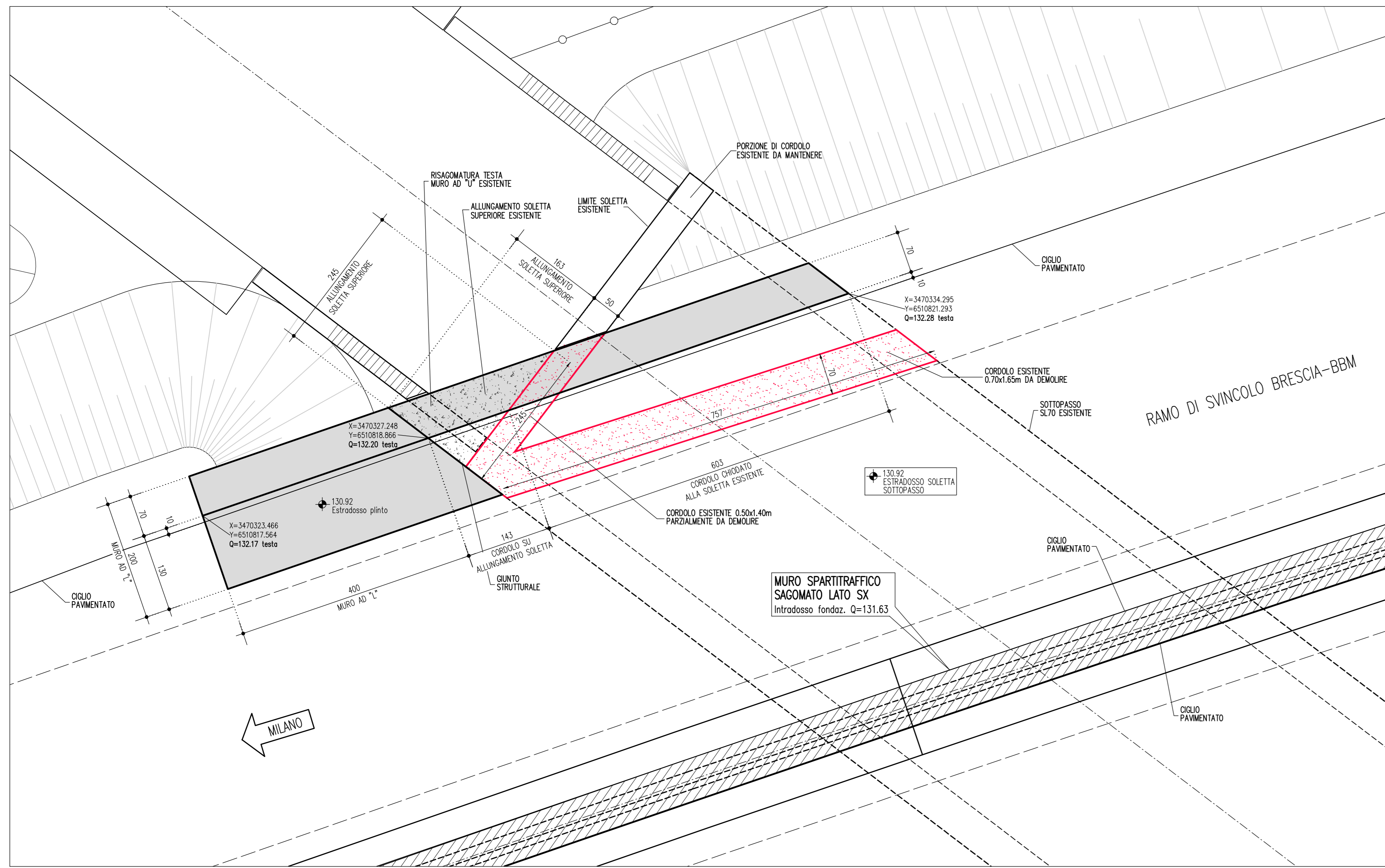
PIANTA CORDOLO -2- (demolizione cordolo esistente) 1:50
