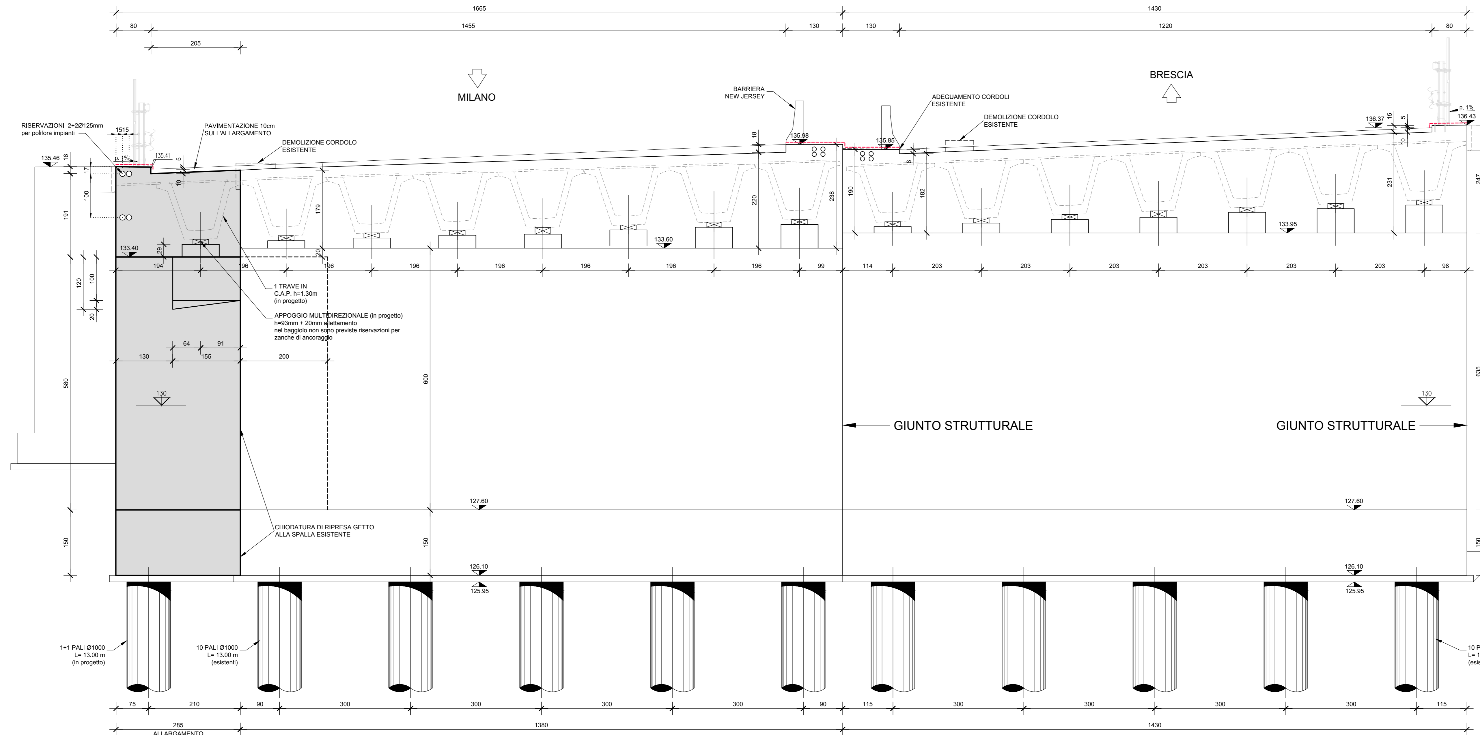
PROSPETTO SPALLA 4 Scala 1:50
