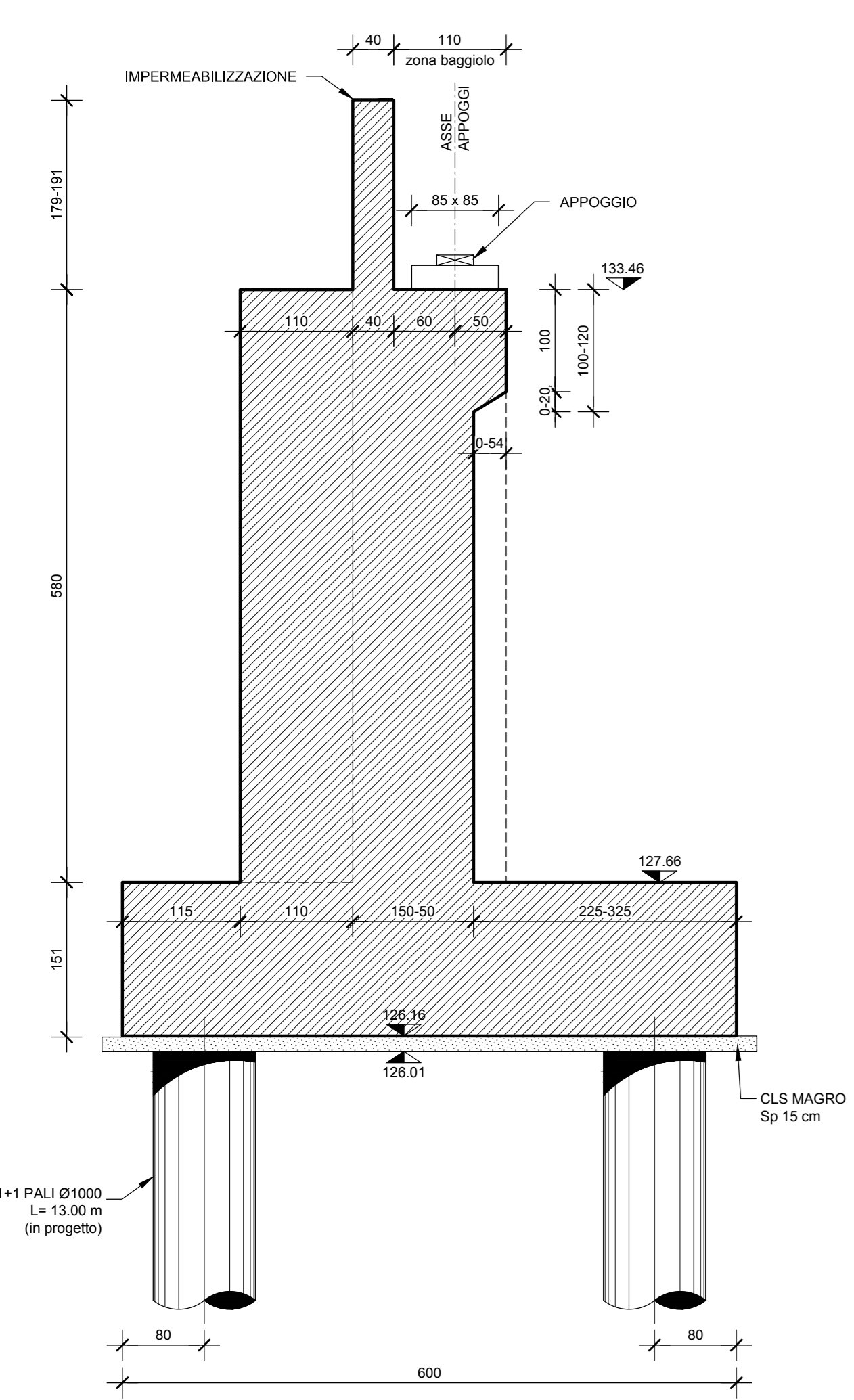
SEZIONE TRASVERSALE ALLARGAMENTO Scala 1:50
