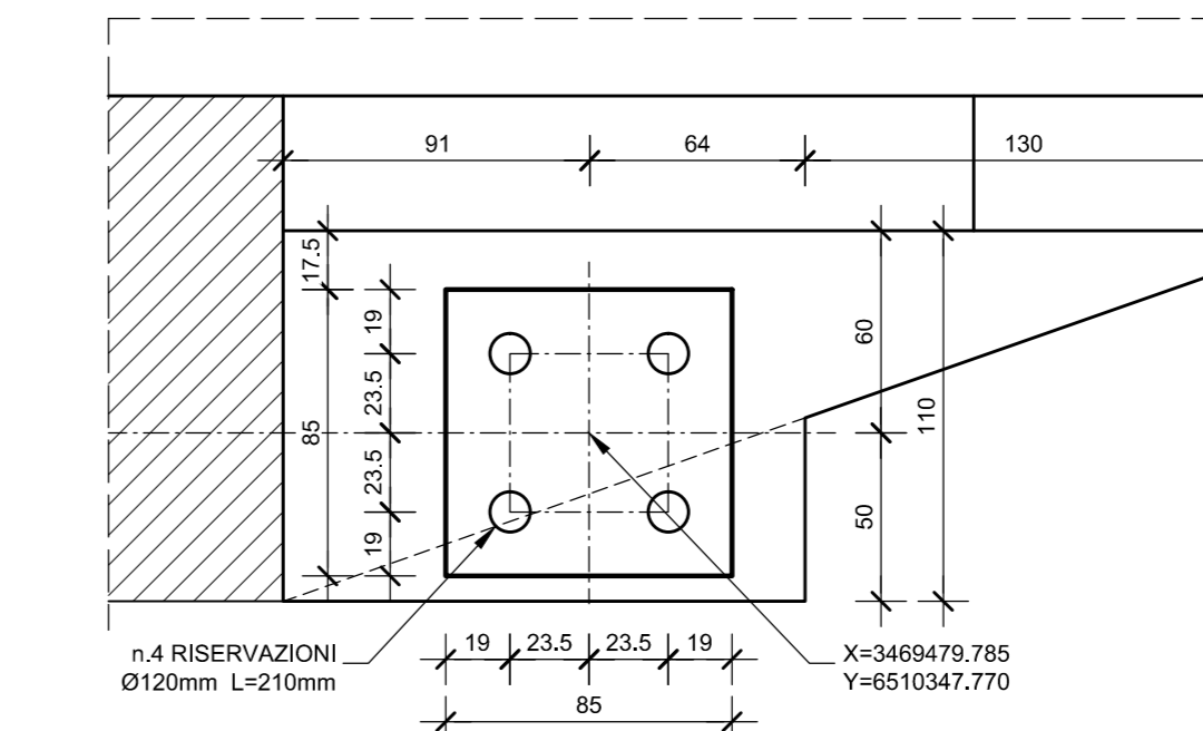
DETTAGLIO BAGGIOLO Scala 1:25
