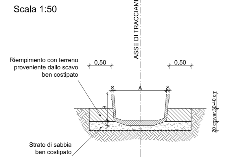
SEZIONE TIPO Elemento in cls prefabbricato tipo Bertazzoli 120/60 Scala 1:50
