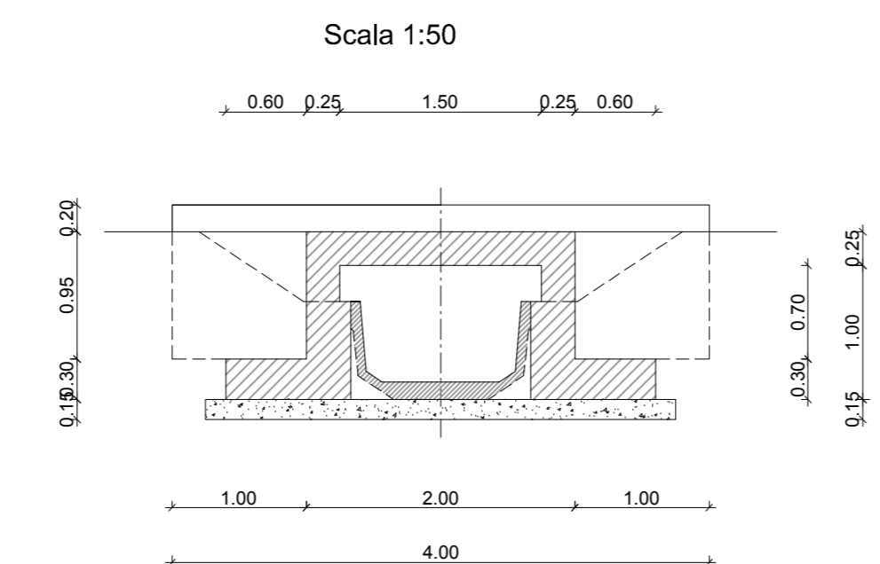
SEZIONE TIPO Cavalcafoso tipo B1 canaletta Bertazzoli 120/60 Scala 1:50
