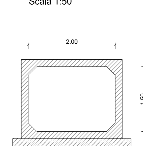
SEZIONE TIPO Tombino scatolare 150x200 Scala 1:50
