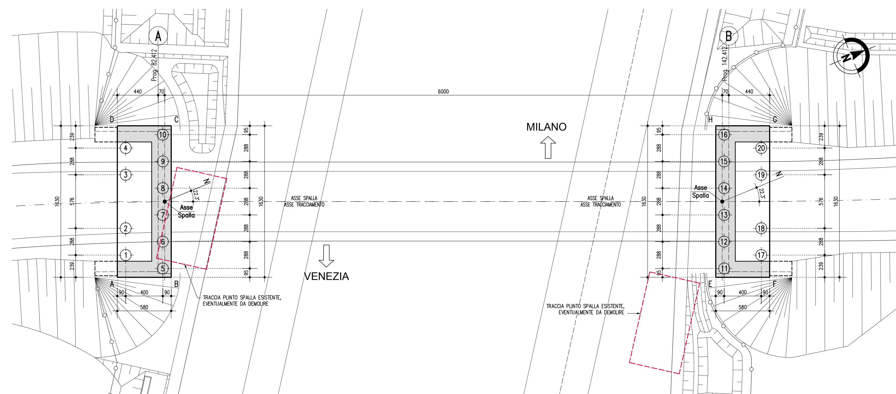
PIANTA TRACCIAMENTO PALI E PLINTI DI FONDAZIONE 1:200
