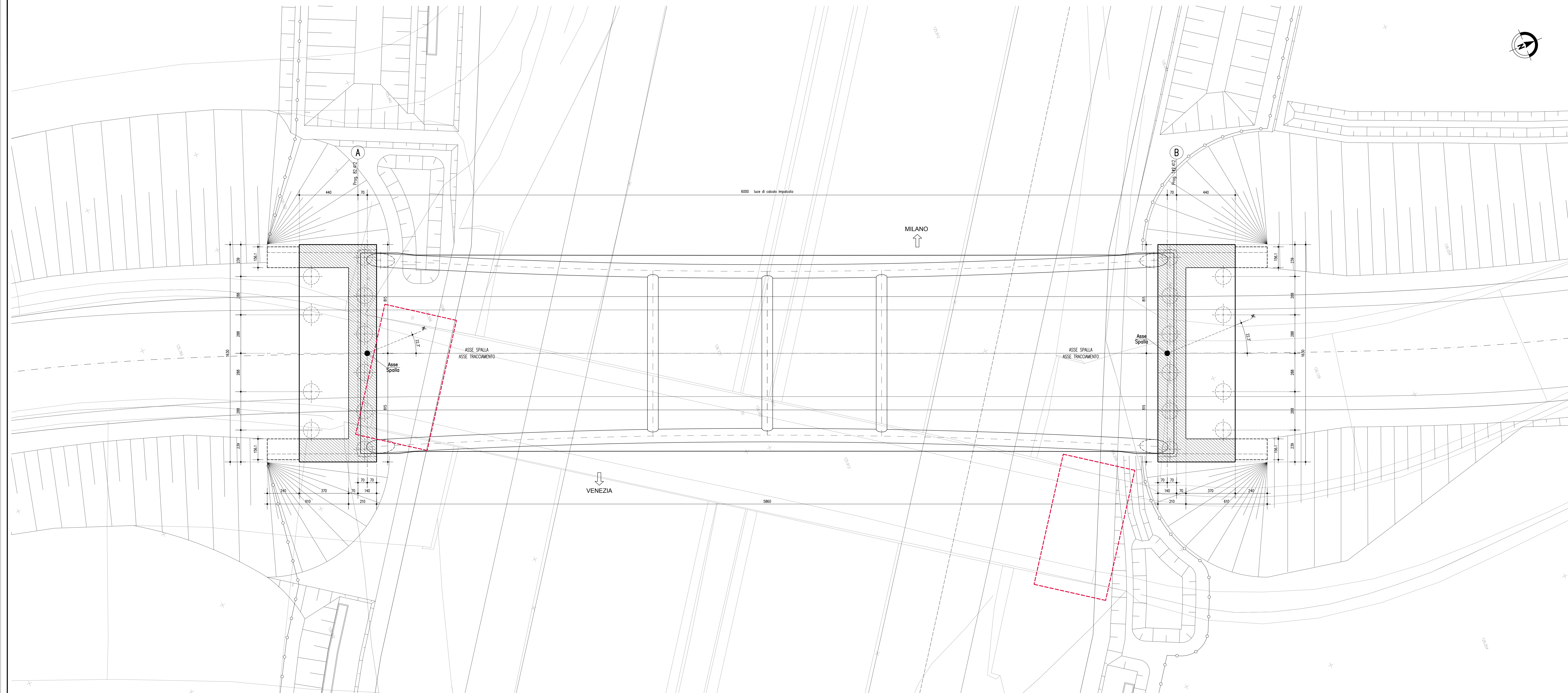
PIANTA FONDAZIONI 1:200
