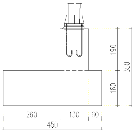
SEZIONE A-A
