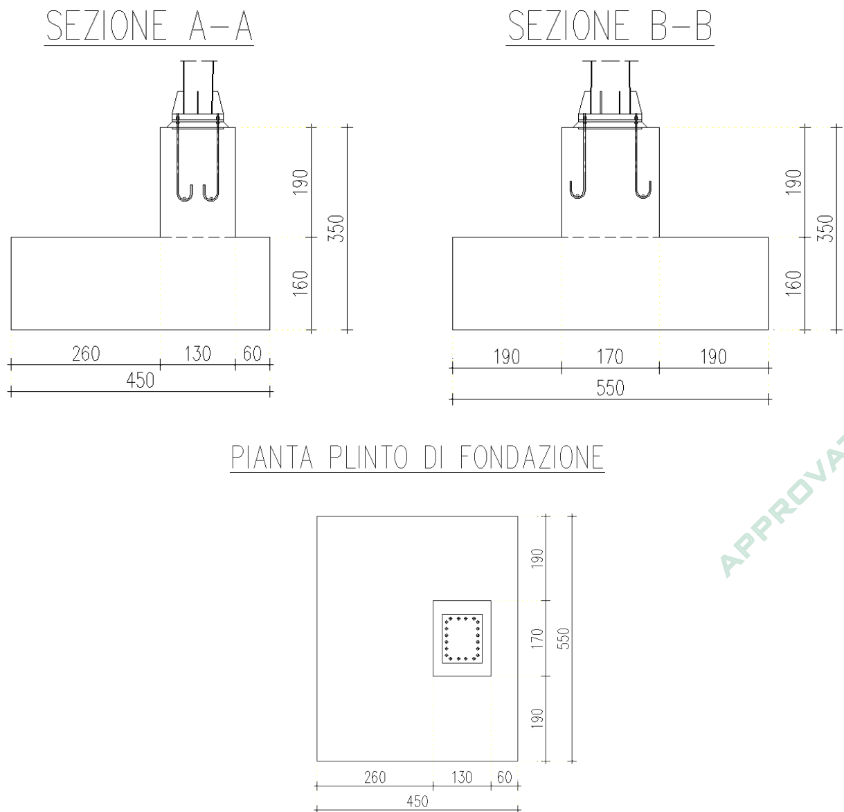
Figura 2 – Geometria delle strutture di fondazione
