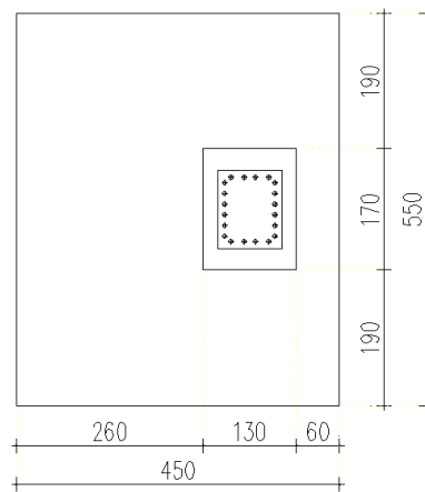
Figura 1 – Geometria dell'apparato fondale.
