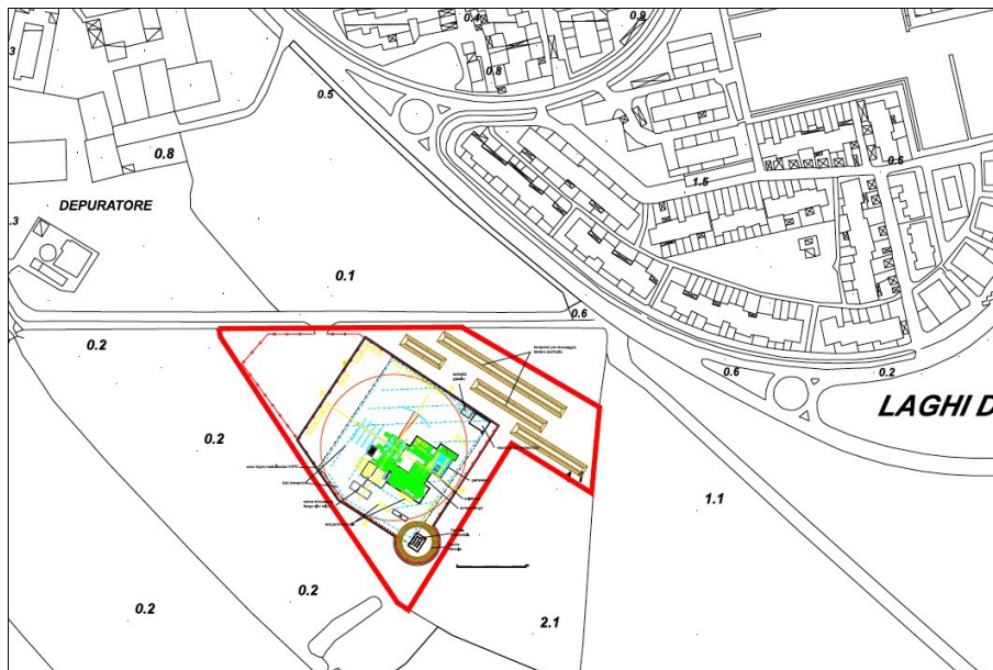
Figura 4 – Planimetria dell'impianto temporaneo di perforazione
