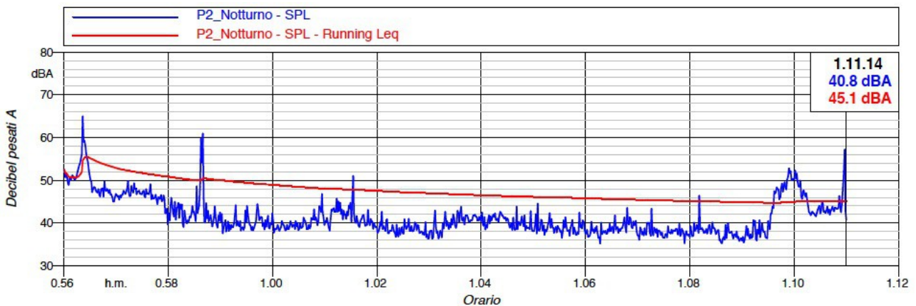
Grafico 4 – Andamento temporale dei livelli sonori misurati nel Punto 02 nel periodo notturno
