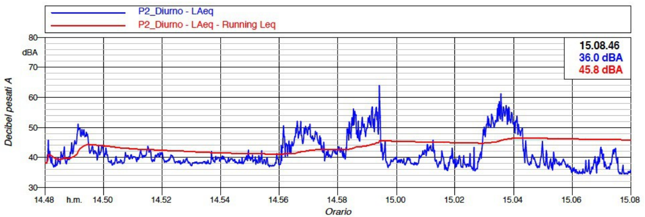
Grafico 3 – Andamento temporale dei livelli sonori misurati nel Punto 02 nel periodo diurno
