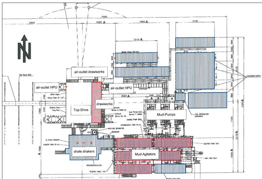
Figura 5 – Localizzazione delle sorgenti rumorose previste nell'impianto di progetto
