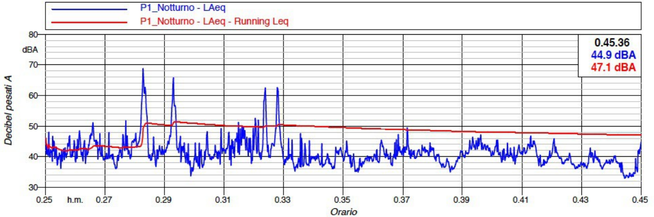
Grafico 2 – Andamento temporale dei livelli sonori misurati nel Punto 01 nel periodo notturno
