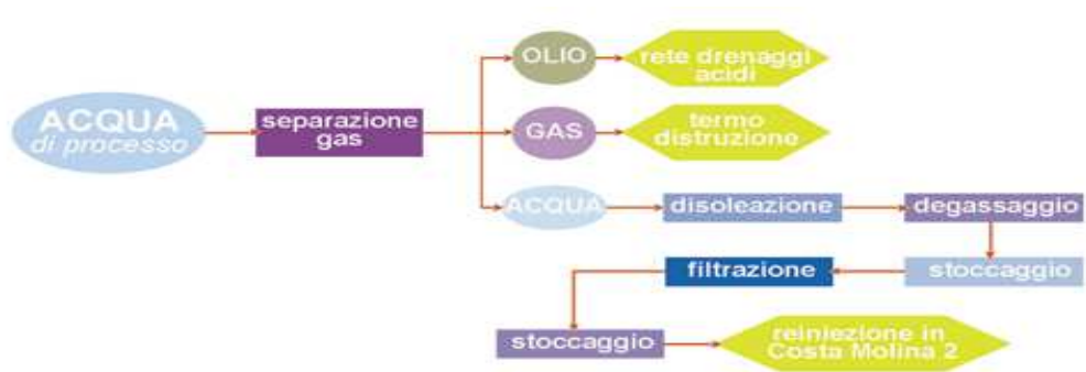
figura 5.1. ciclo dell'acqua di processo nel Centro Oli Val d'Agri
