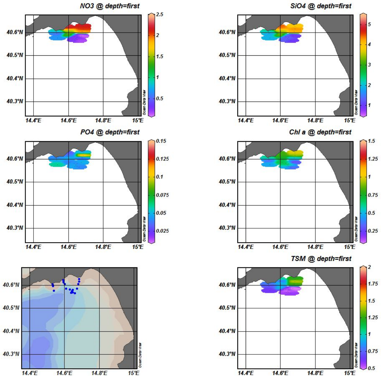
Figura 1.4 - Distribuzione superficiale di NO 3 , SiO 4 e PO 4 (mmol m -3 ), Chl a (mg m -3 ) e TSM (g m -3 ) durante la campagna effettuata in corrispondenza del 20% del materiale dragato (20/03/2004).
