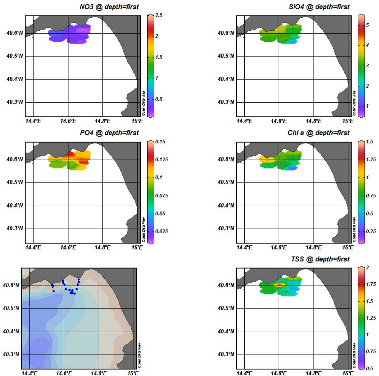
Figura 1.15 - Distribuzione superficiale di \text{NO}_3 , \text{SiO}_4 e \text{PO}_4 ( \text{mmol m}^{-3} ), Chl a ( \text{mg m}^{-3} ) e TSS ( \text{g m}^{-3} ) durante la campagna effettuata al termine dei lavori di dragaggio (26-27/04/2004).
