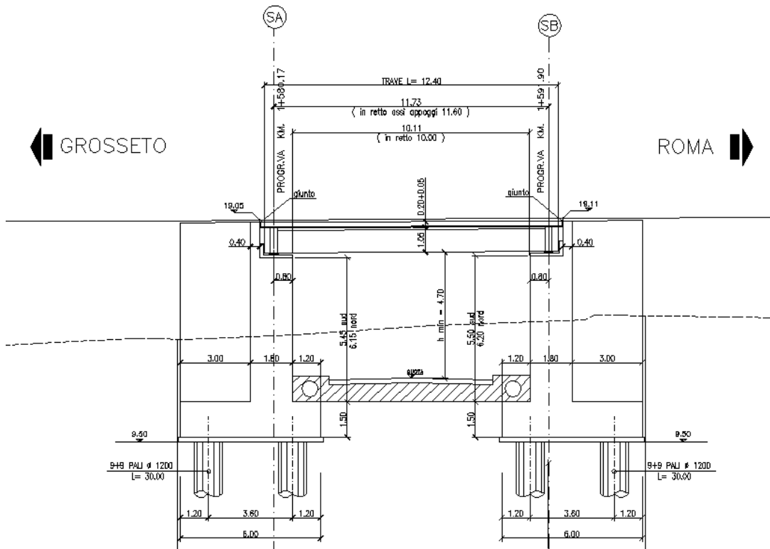
SEZIONE LONGITUDINALE-ST05
