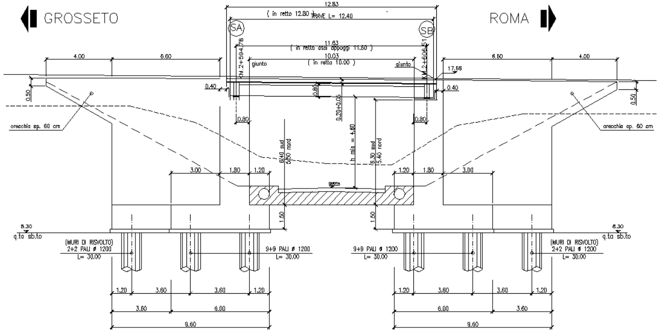
SEZIONE LONGITUDINALE-ST02
