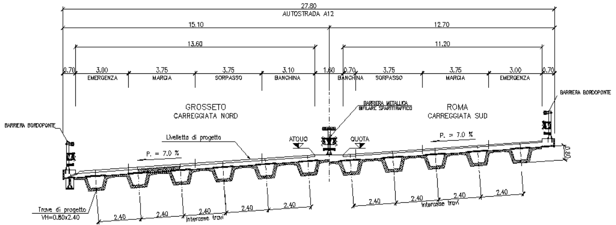
SEZIONE TRASVERSALE-ST02
