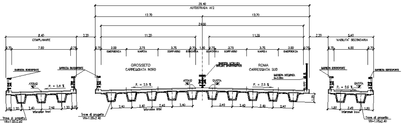
SEZIONE TRASVERSALE
