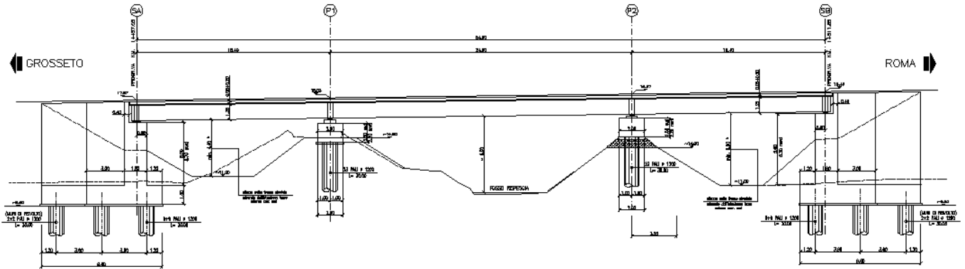
PROFILO LONGITUDINALE
