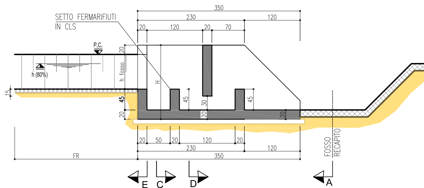
SEZIONE B-B
