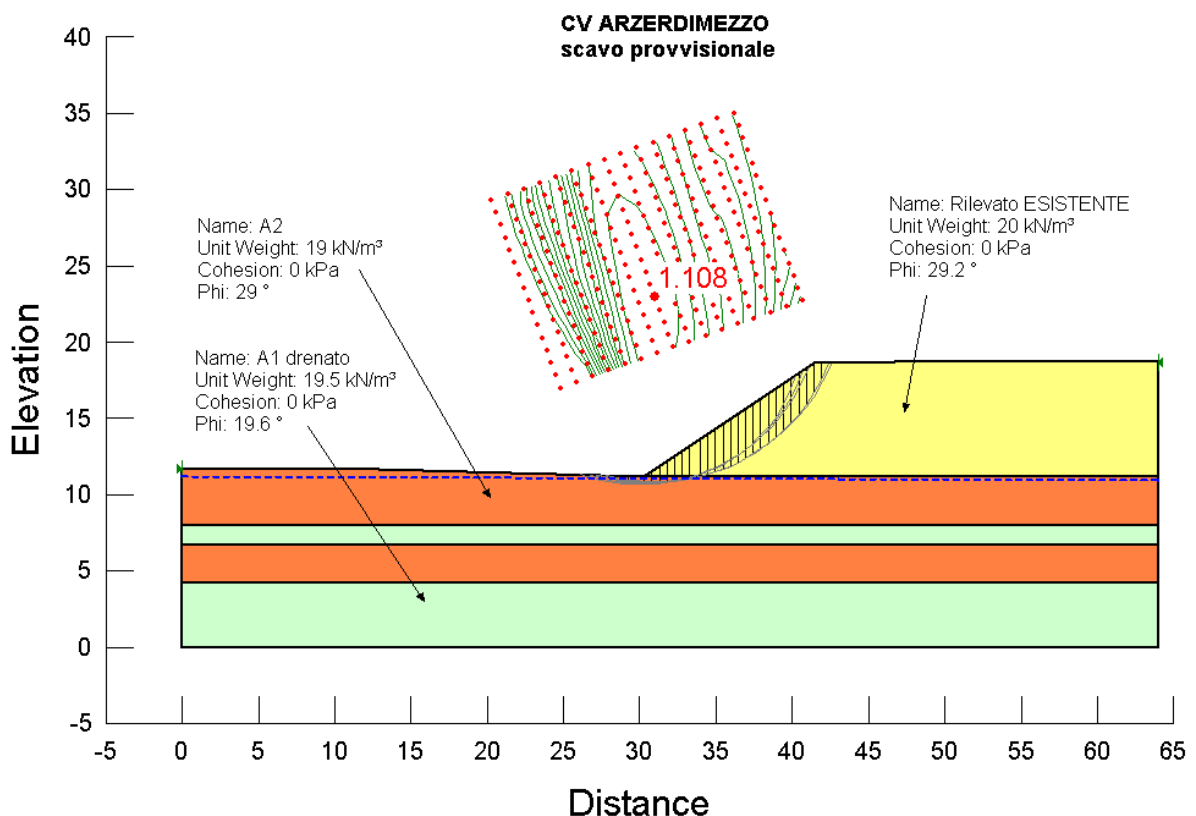
Figura 1: Verifica di stabilità globale dello scavo provvisorio
