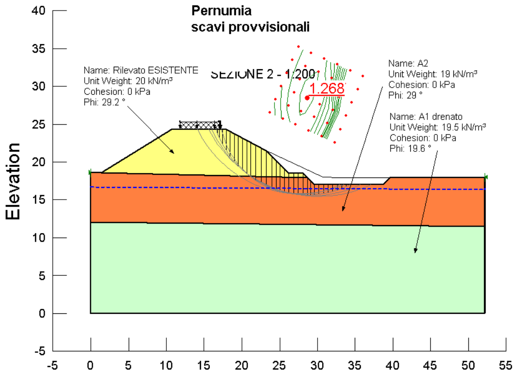
: Figura 25: Verifica di stabilità globale palancola sez. 2
