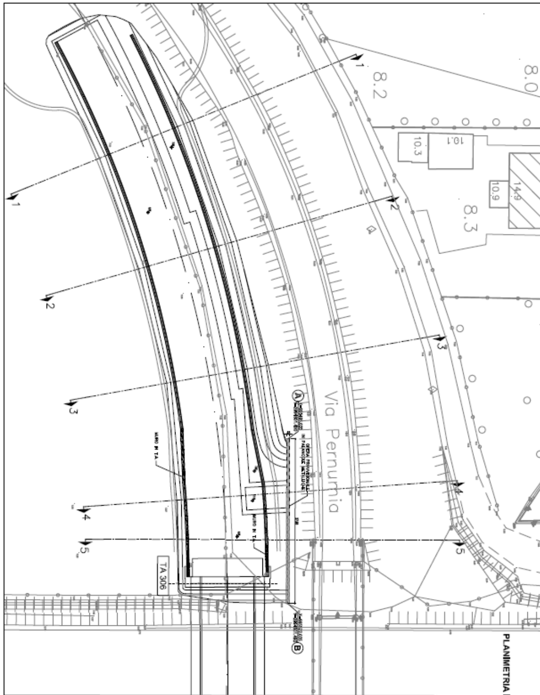
Figura 8-1 - Muro TA306: sviluppo in pianta palancole
