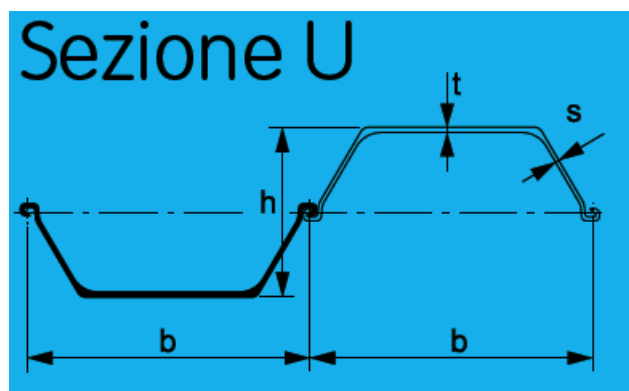
Figura 8-15: Sezione tipo delle palancole
