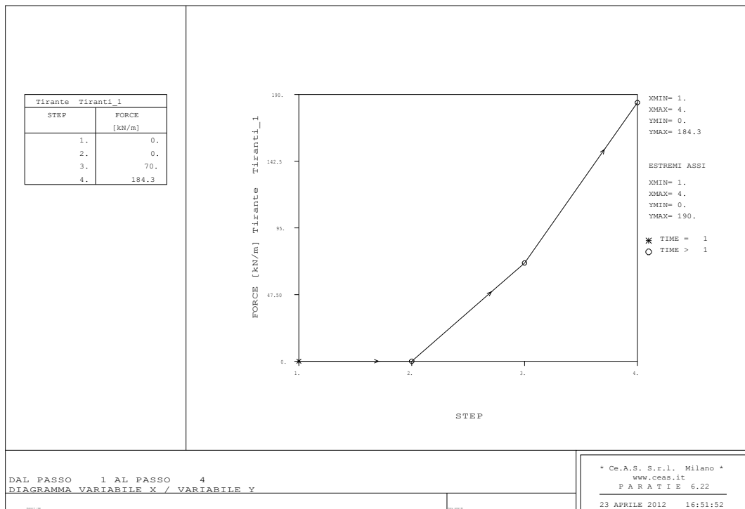
Figura 8-8: SLU A1 - Schema 1, Azione assiale massima nei tiranti del 1° ordine
