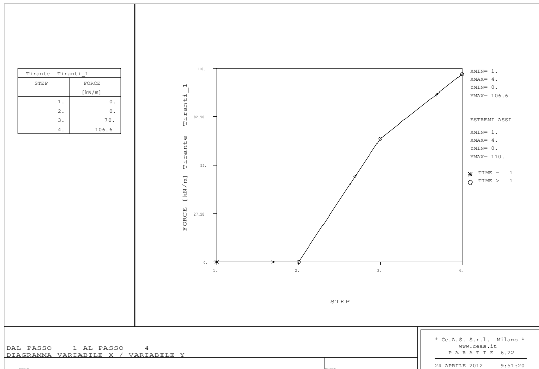
Figura 8-20: SLU A1 - Schema 3, Azione assiale massima nei tiranti del 1° ordine
