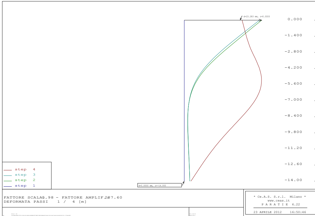
Figura 8-5: SLE – Schema 1, Diagramma di spostamento
