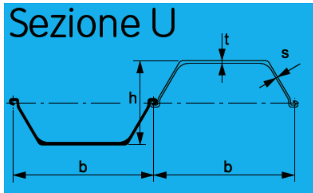
Figura 8-21: Sezione tipo delle palancole
