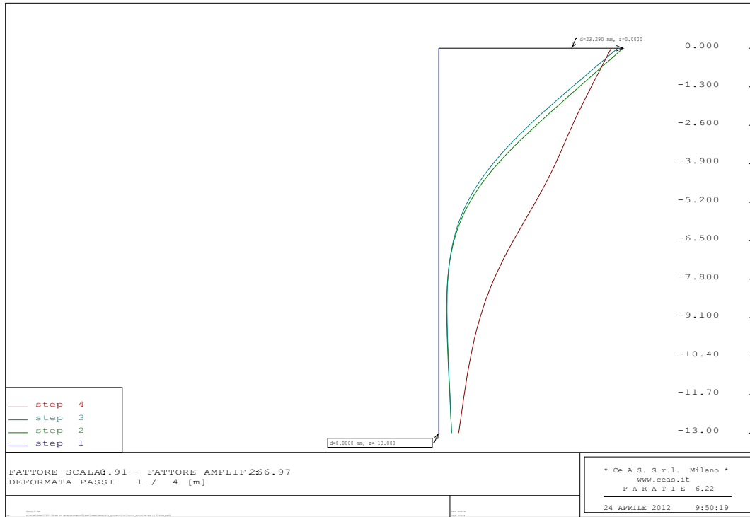
Figura 8-17: SLE - Schema 3, Diagramma di spostamento
