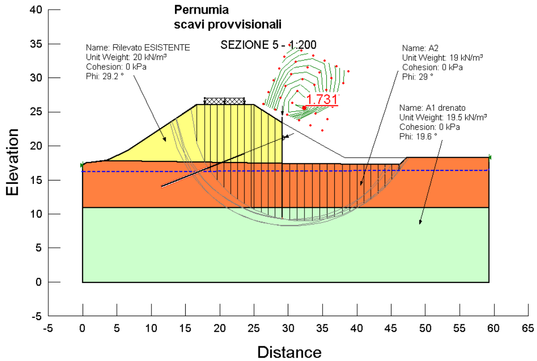
Figura 24: Verifica di stabilità globale palancola sez. 5
