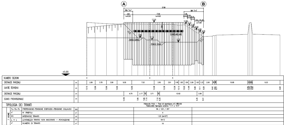
Figura 8-3 - Muro TA306: prospetto
