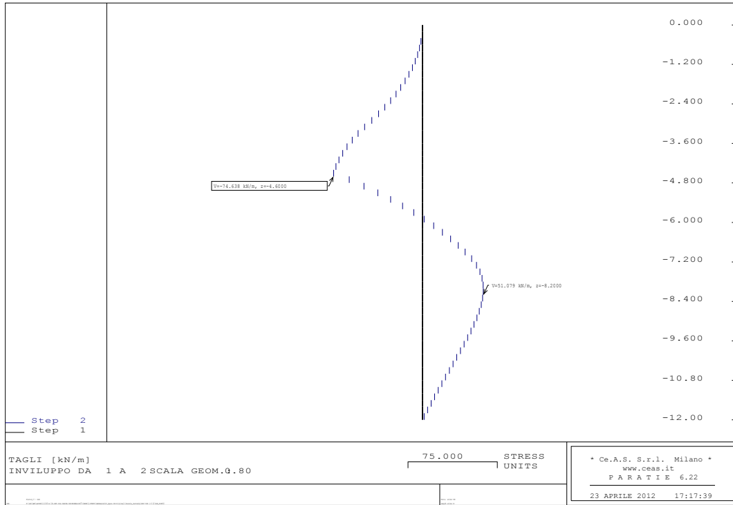
Figura 8-14: SLU A1 - Schema 2, Diagramma del taglio
