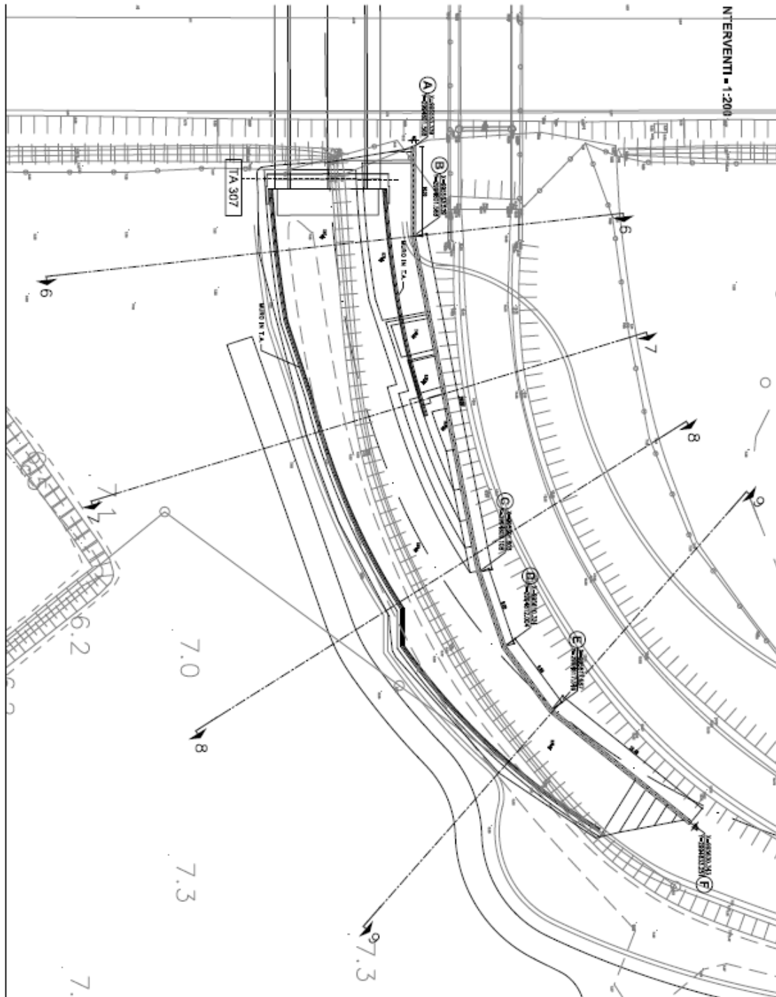
Figura 8-2 – Muro TA307: sviluppo in pianta palancola
