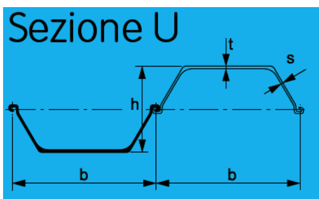
Figura 8-9: Sezione tipo delle palancole
