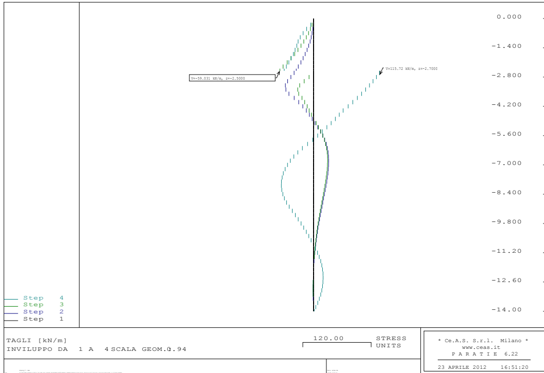
Figura 8-7: SLU A1 - Schema 1, Diagramma del taglio
