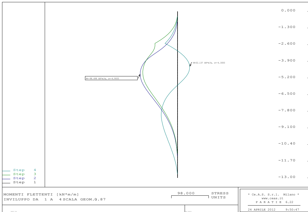
Figura 8-18: SLU A1 - Schema 3, Diagramma del momento flettente
