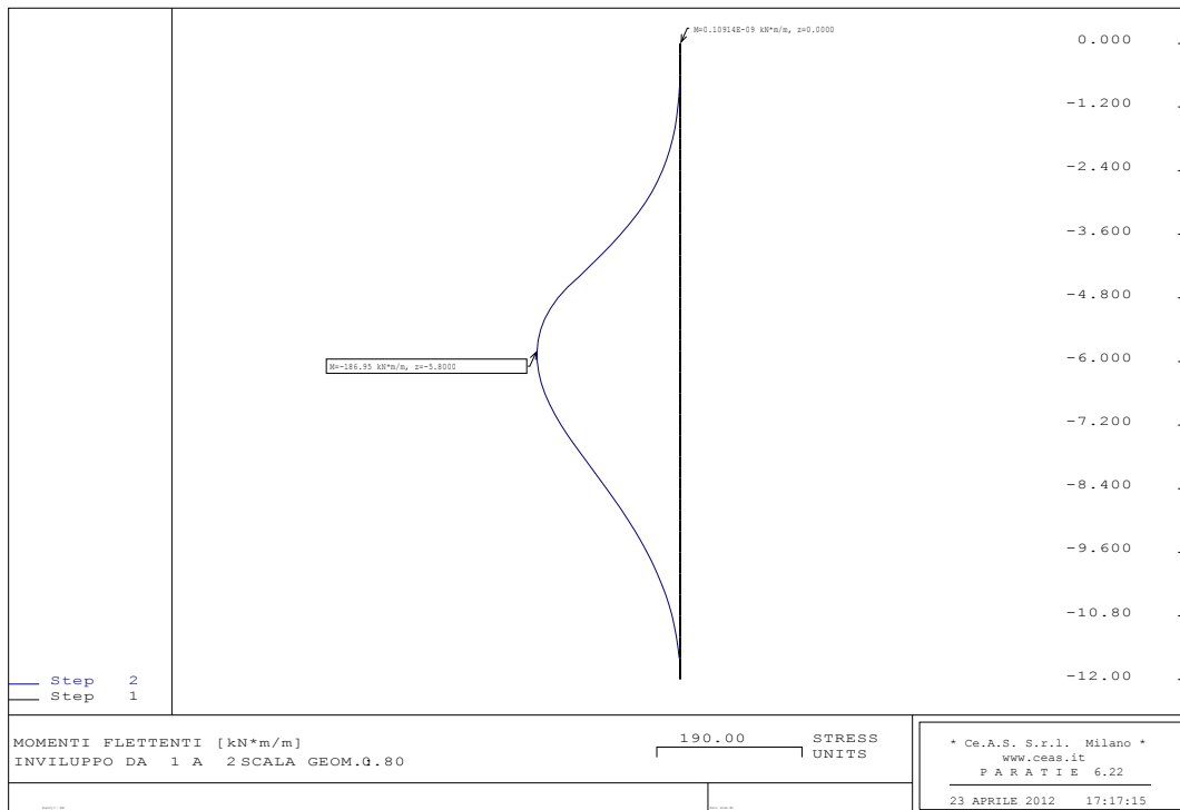
Figura 8-13: SLU A1 - Schema 2, Diagramma del momento flettente
