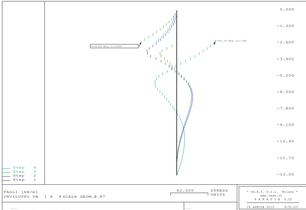
Figura 8-19: SLU A1 - Schema 3, Diagramma del taglio
