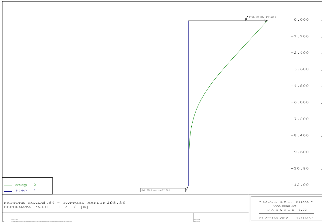
Figura 8-12: SLE - Schema 2, Diagramma di spostamento
