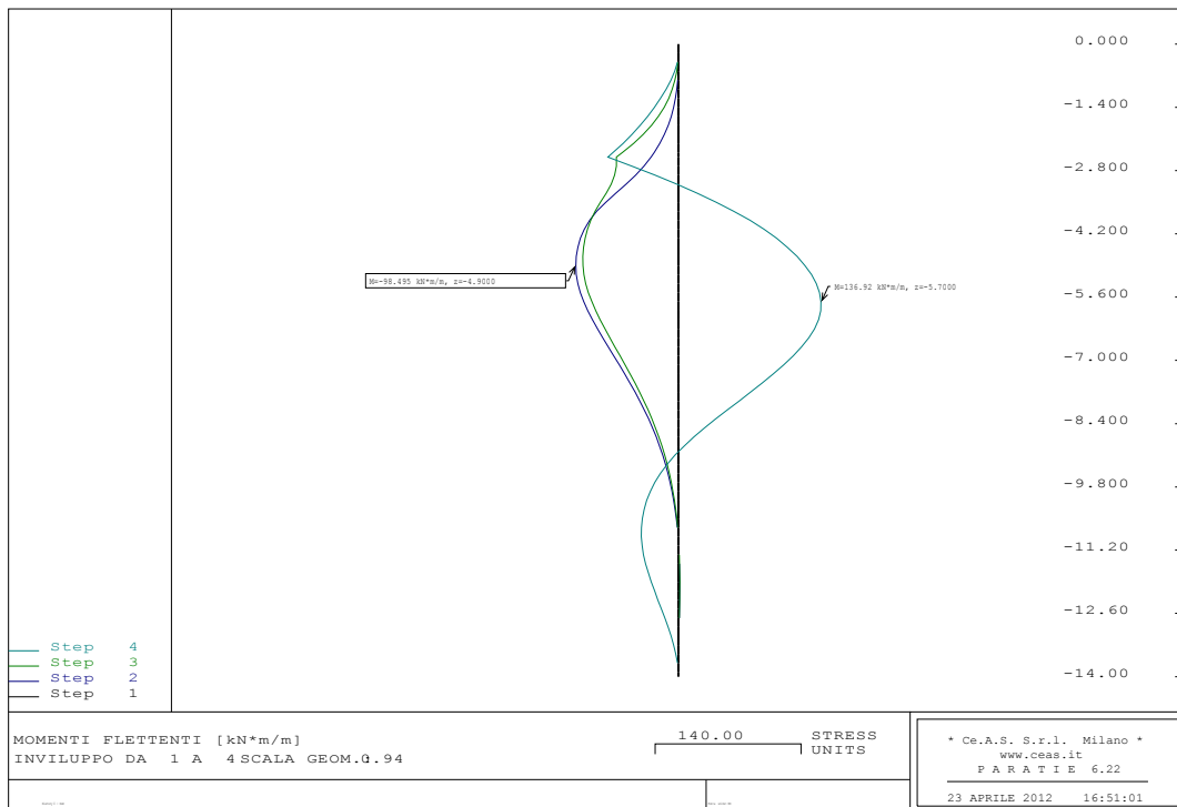
Figura 8-6: SLU A1 - Schema 1, Diagramma del momento flettente
