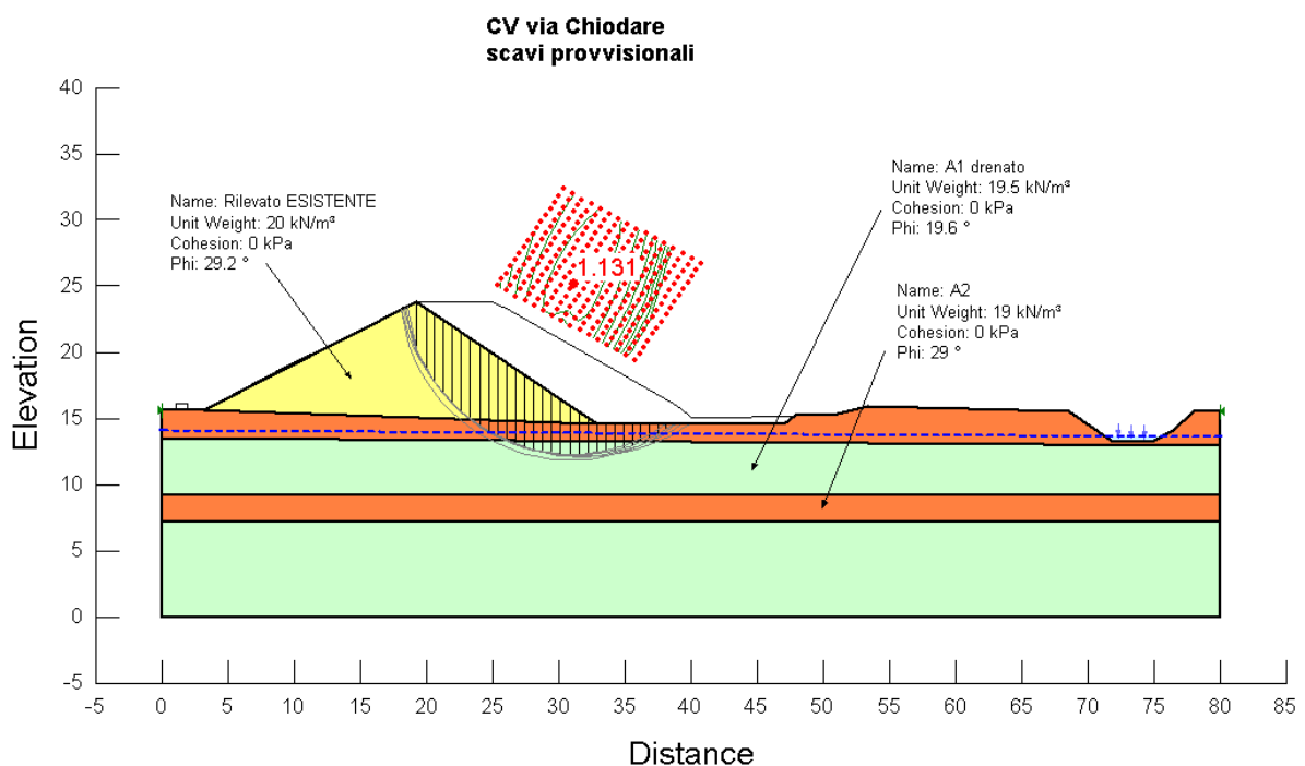
Figura 1: Verifica di stabilità globale dello scavo provvisorio
