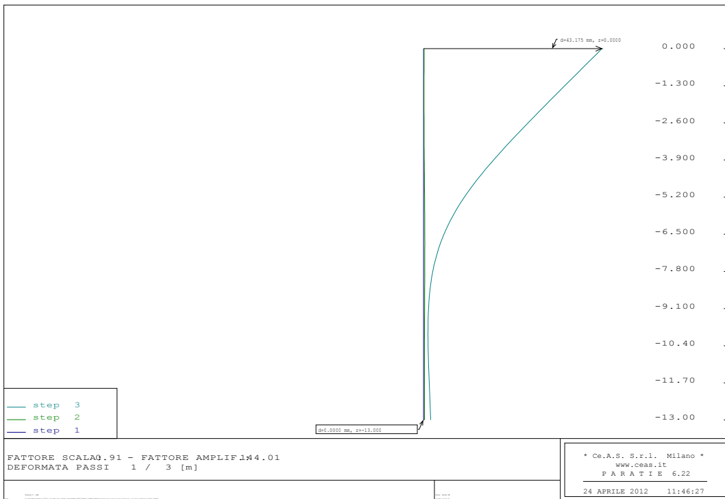
Figura 8-4: SLE – Schema 1, Diagramma di spostamento
