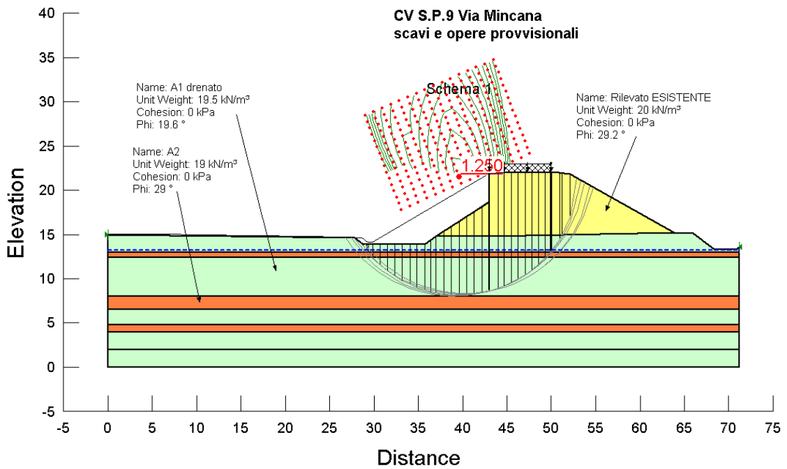
Figura 16: Verifica di stabilità globale palancola SCHEMA 1
