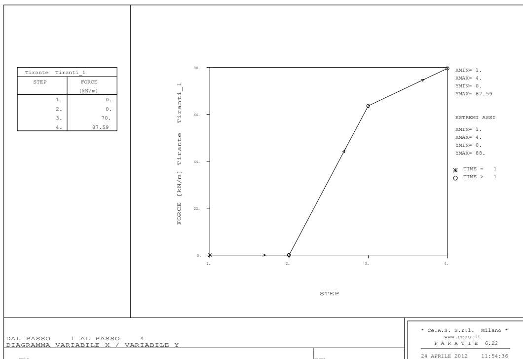
Figura 8-12: SLU A1 - Schema 2, Azione assiale massima nei tiranti del 1° ordine
