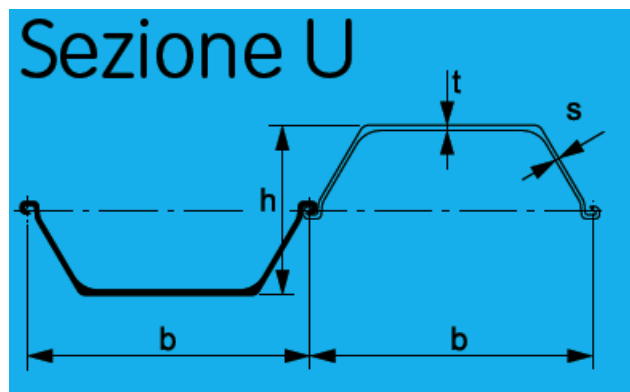
Figura 8-7: Sezione tipo delle palancole
