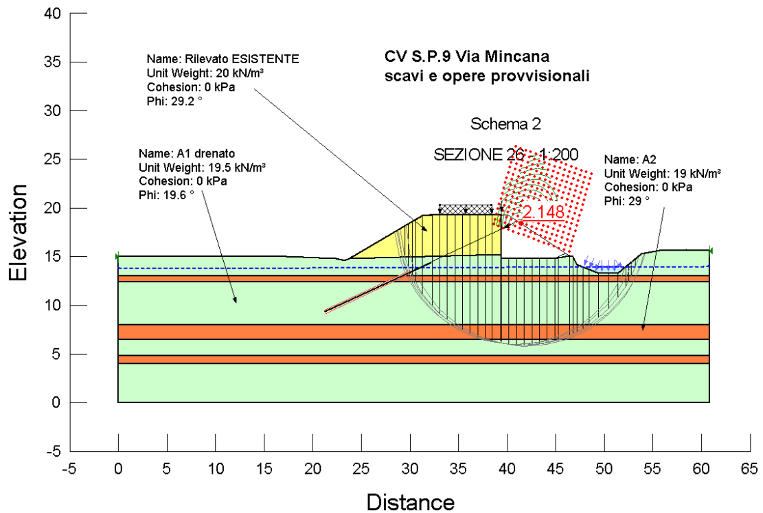
Figura 17: Verifica di stabilità globale palancola SCHEMA 2
