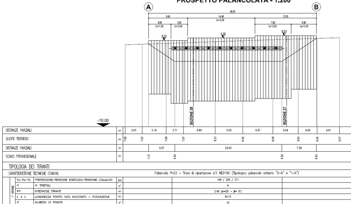
PROSPETTO PALANCOLATA - 1:200
