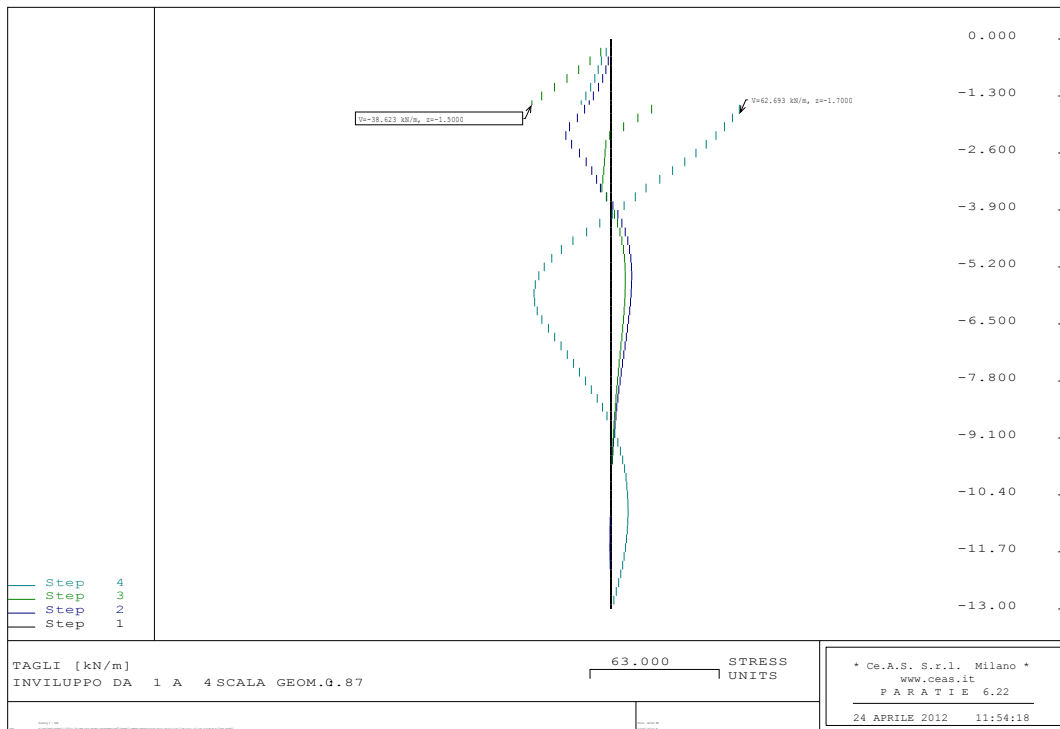
Figura 8-11: SLU A1 - Schema 2, Diagramma del taglio
