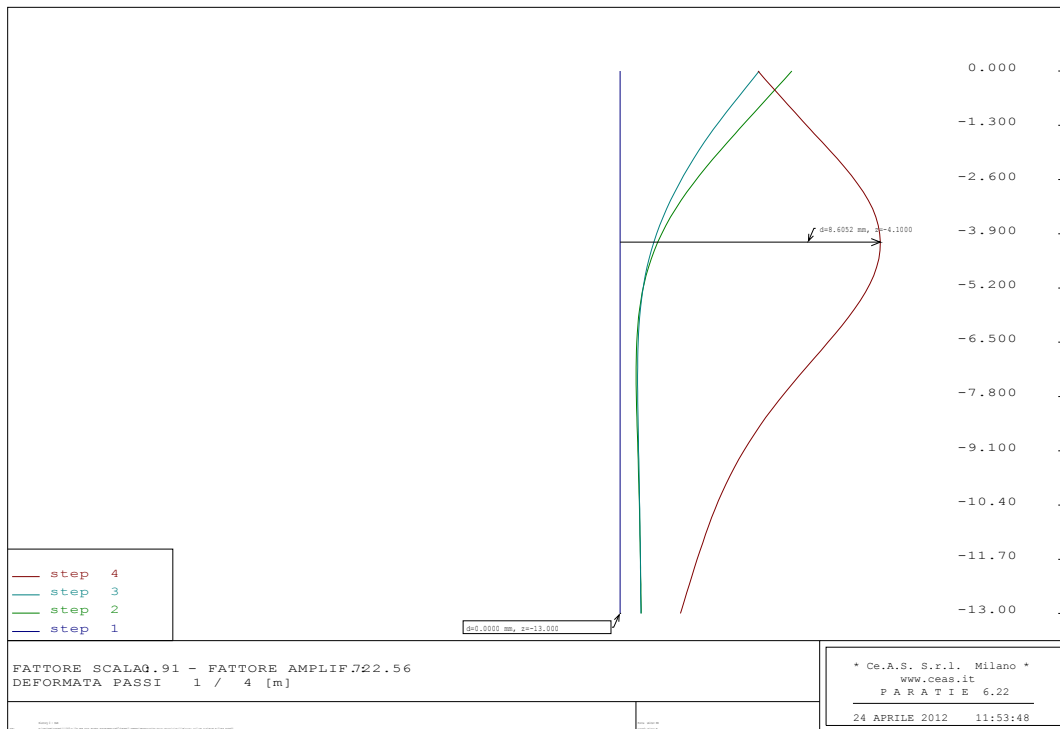
Figura 8-9: SLE - Schema 2, Diagramma di spostamento
