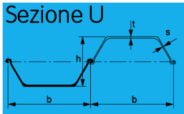
Figura 8-13: Sezione tipo delle palancole
