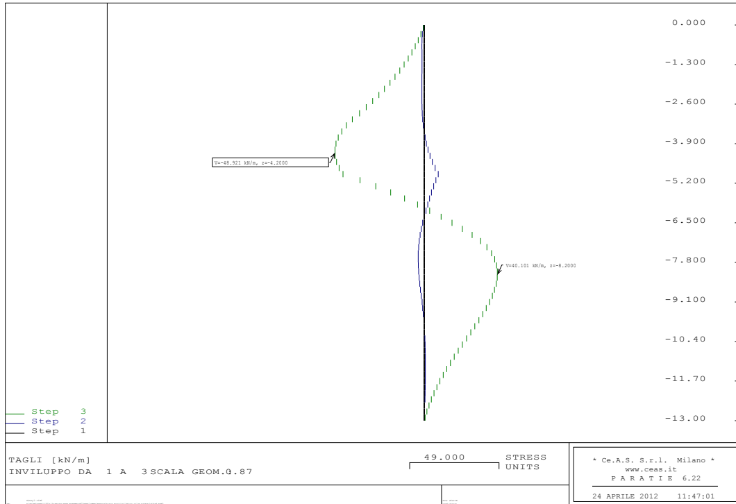
Figura 8-6: SLU A1 - Schema 1, Diagramma del taglio
