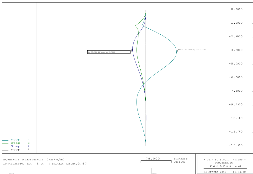
Figura 8-10: SLU A1 - Schema 2, Diagramma del momento flettente
