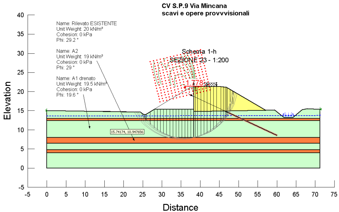
Figura 19: Verifica di stabilità globale palancola SCHEMA 1-h
