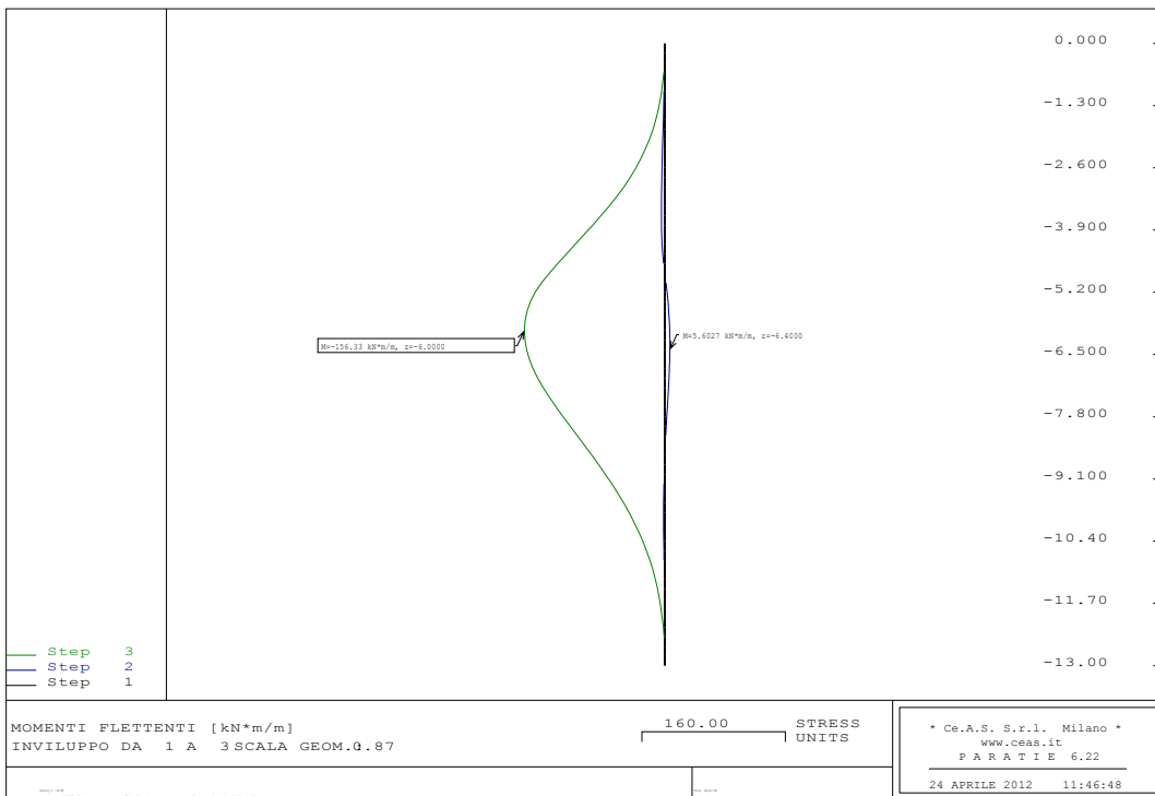
Figura 8-5: SLU A1 - Schema 1, Diagramma del momento flettente
