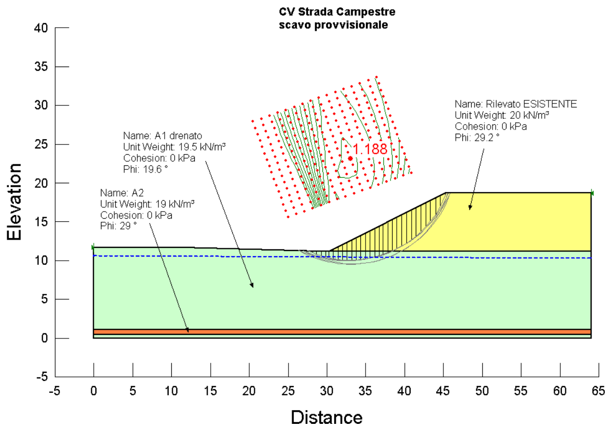
Figura 1: Verifica di stabilità globale dello scavo provvisorio
