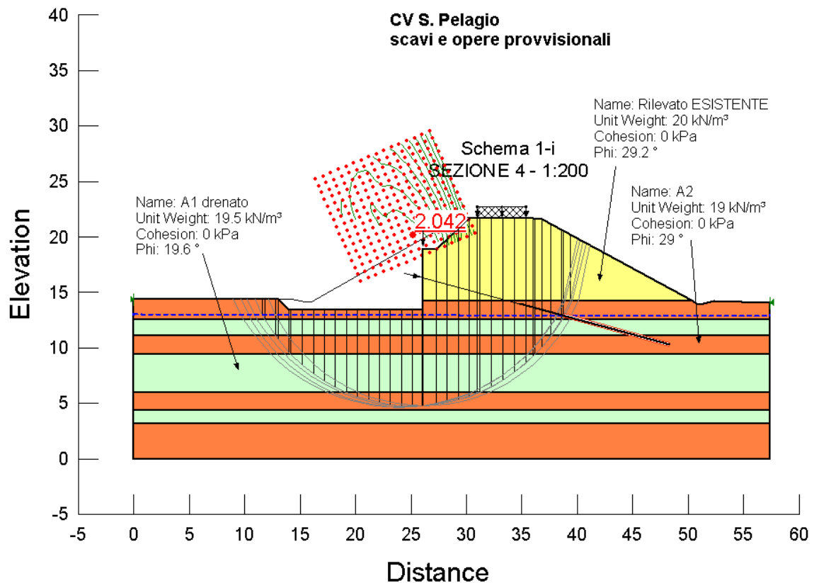
Figura 2: Verifica di stabilità globale palancola SCHEMA 1-i
