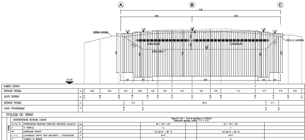
Figura 8-1 - Muro TA331: sviluppo in pianta palanca e prospetto
