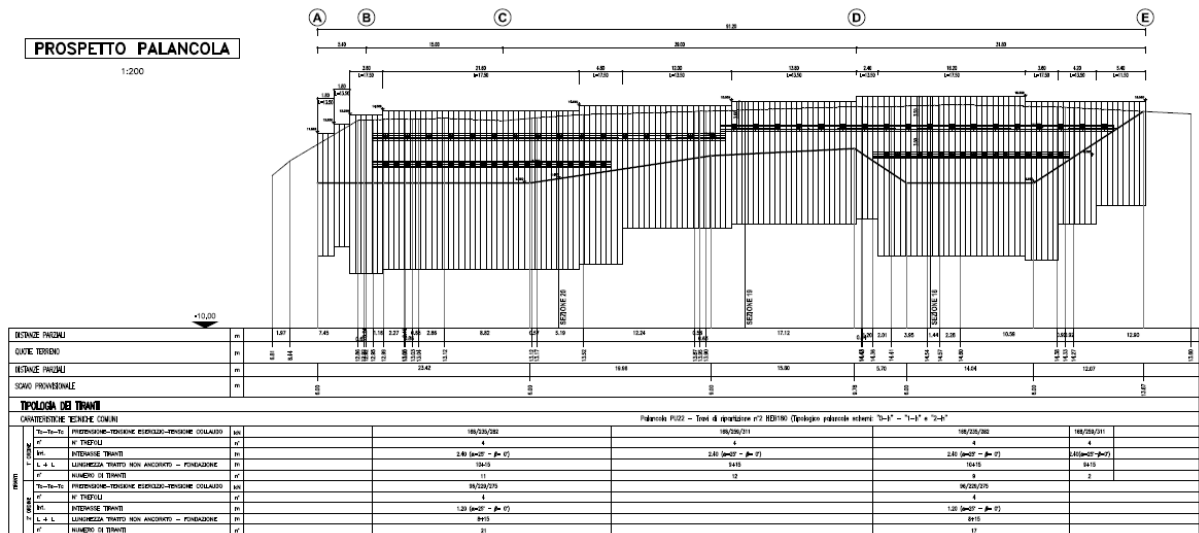
Figura 8-1 - Muro TA342: sviluppo in pianta palancola e prospetto
