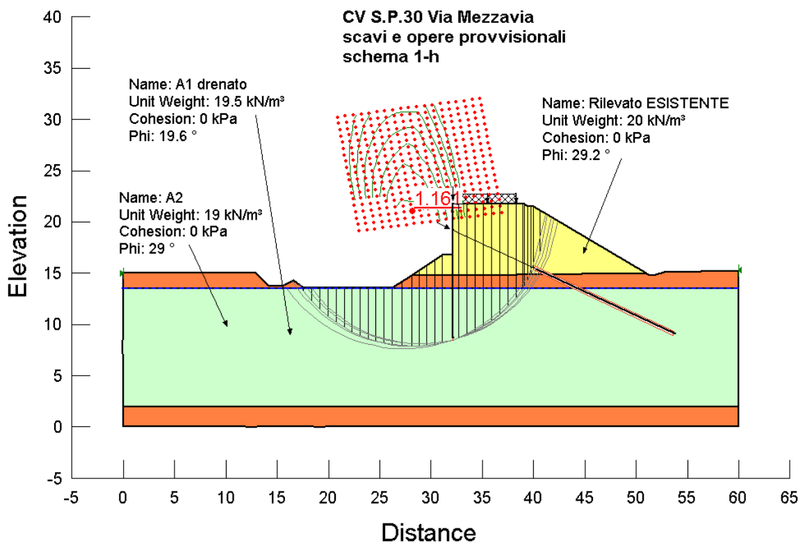
Figura 2: Verifica di stabilità globale palanca SCHEMA 1-h
