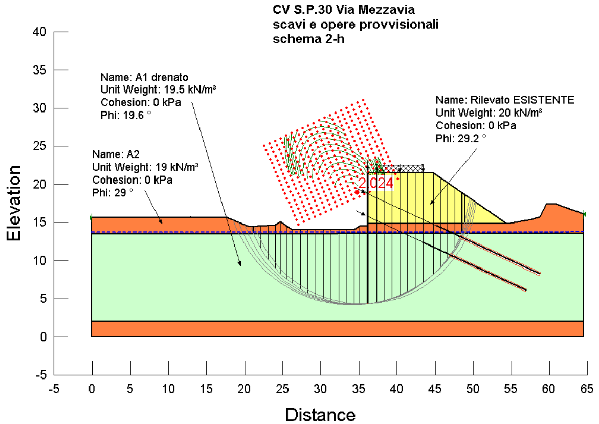
: Figura 3: Verifica di stabilità globale palancola SCHEMA 2-h
