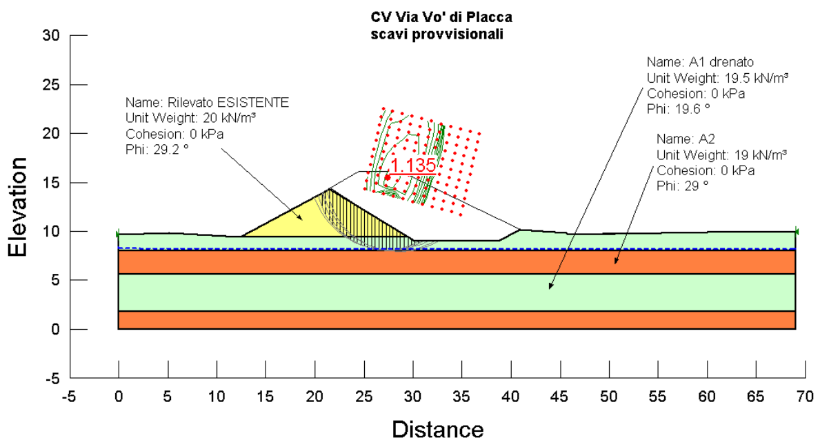
Figura 1: Verifica di stabilità globale dello scavo provvisorio
