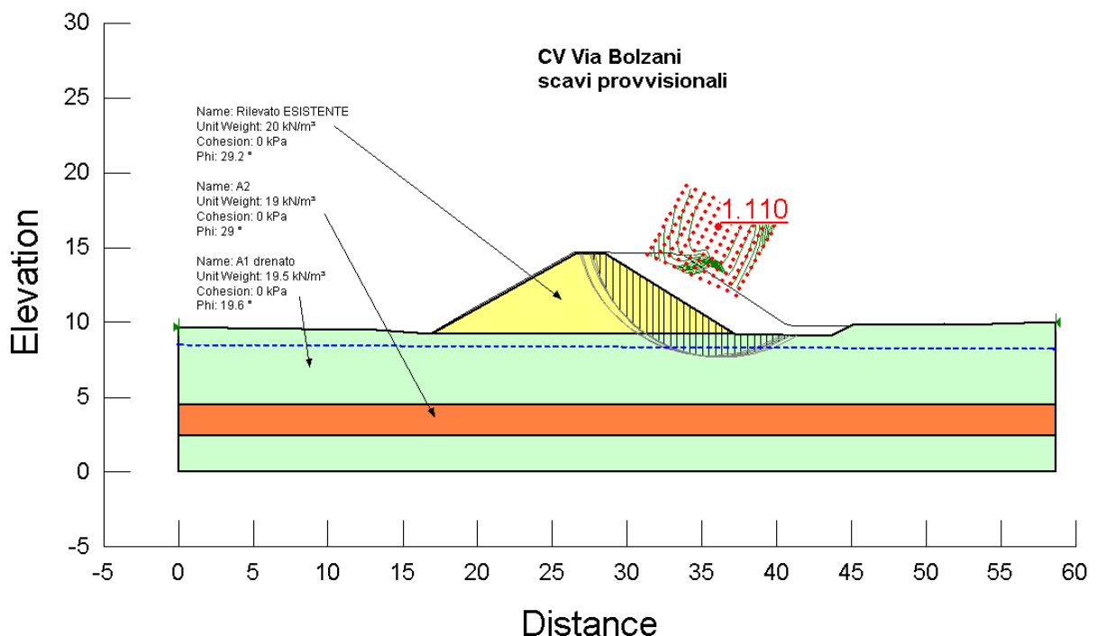
Figura 1: Verifica di stabilità globale dello scavo provvisorio
