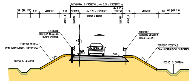
SEZIONE TIPO RACCORDO FRA CORSA SPECIALIZZATA E RAMPA DI SVINCOLO ESISTENTE
