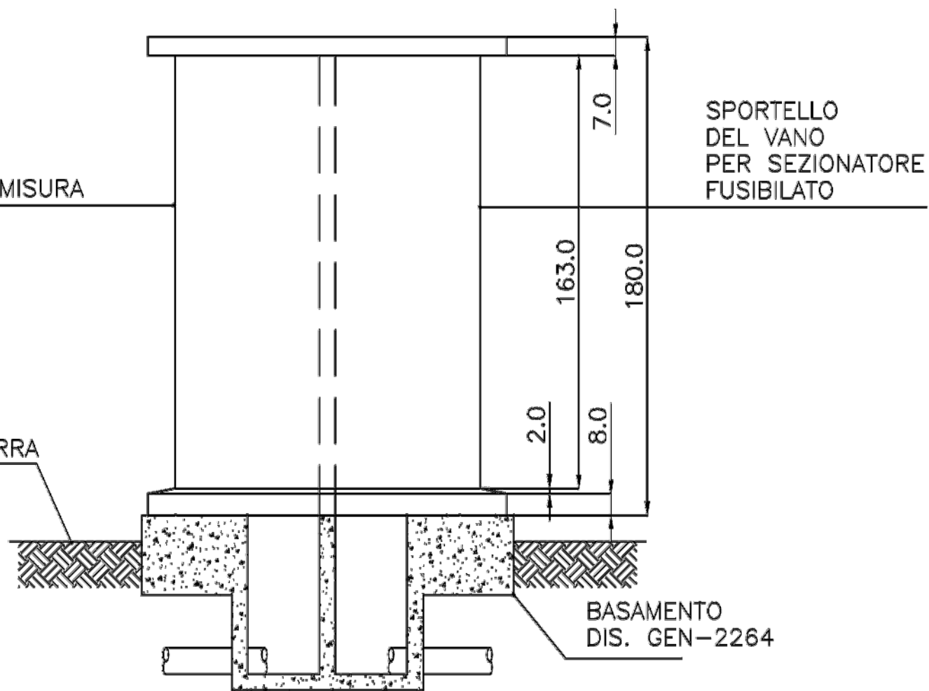
PROSPETTO LATERALE
