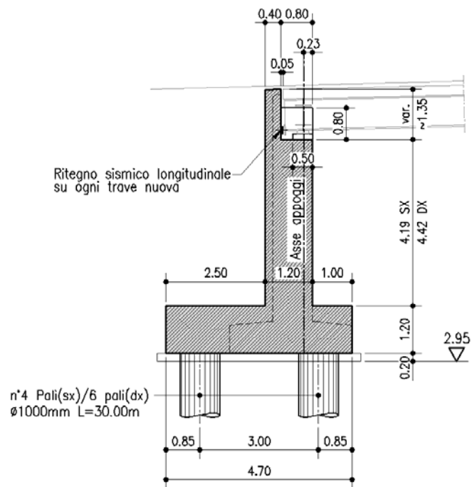
Figura 1-7 - Sezione longitudinale spalla in ampliamento
