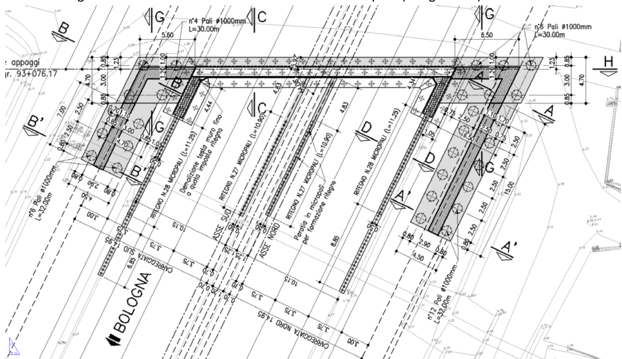
Figura 1-4 - Pianta con localizzazione tiranti a tergo spalla
