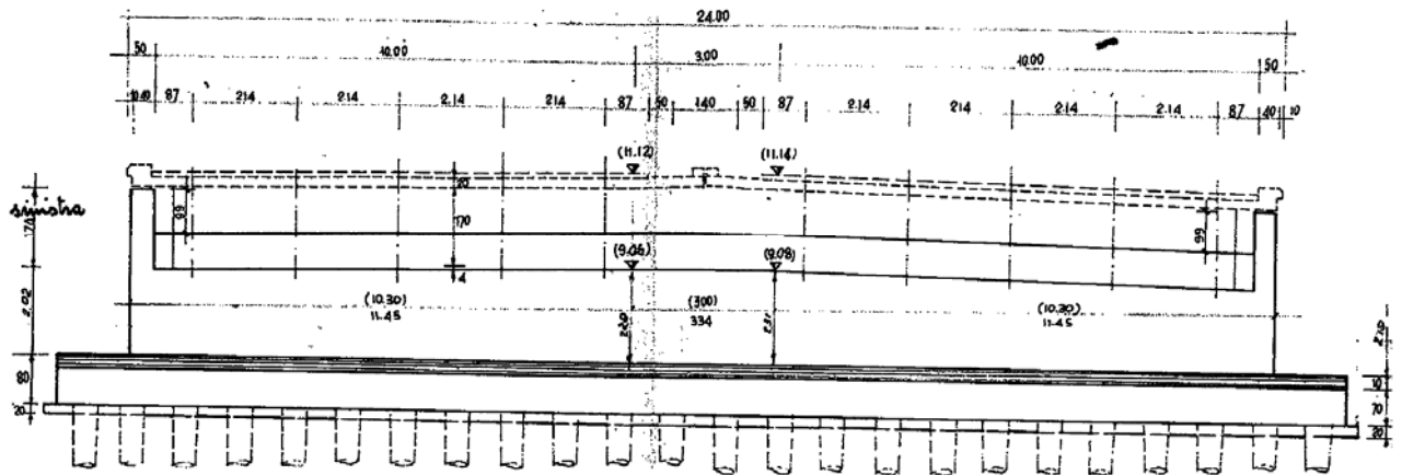
Figura 1-9 - Prospetto pila esistente
