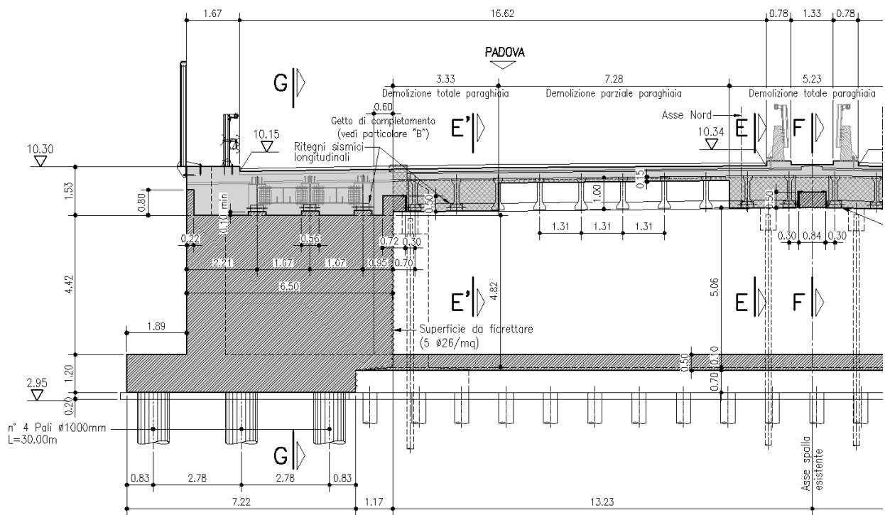
Figura 1-6 - Semi-prospetto spalle con ampliamento
