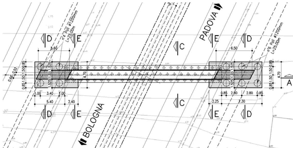
Figura 1-13 - Pianta pile esistenti ed in ampliamento
