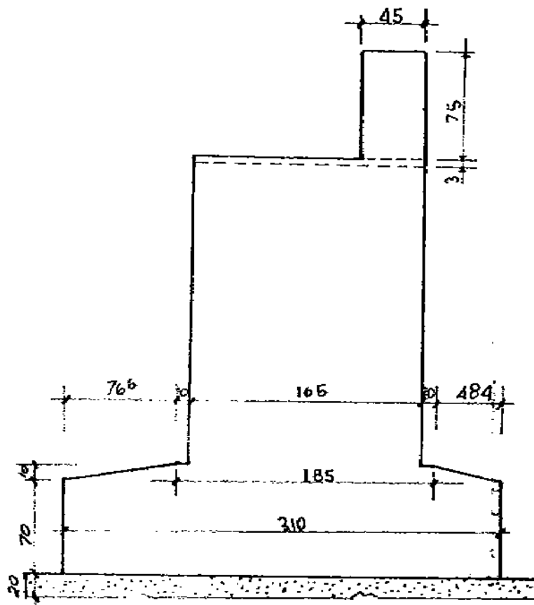
Figura 1-8 - Sezione trasversale pila esistente
