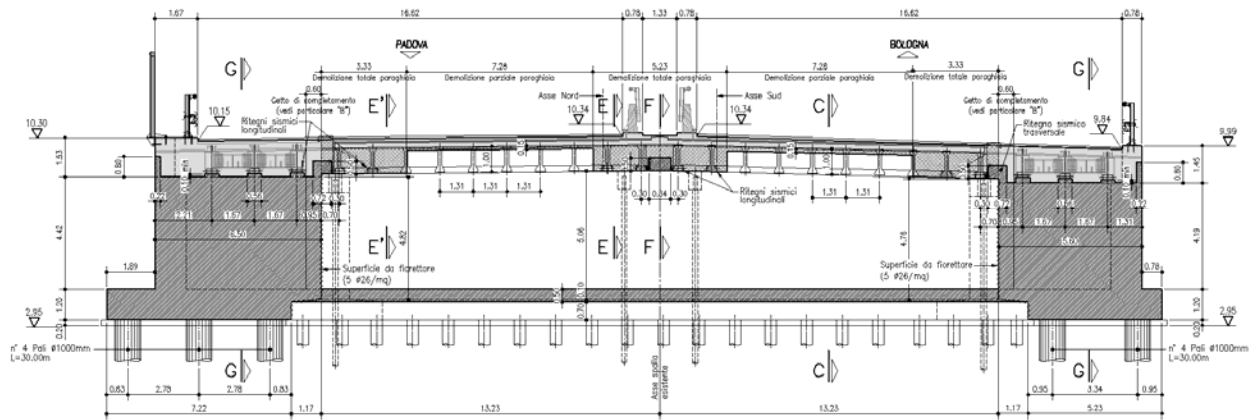
Figura 7-1 - Prospetto spalla con notazione ritegni trasversali (campate laterali)
