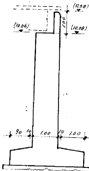
Figura 1-1 - Sezione trasversale spalla esistente
