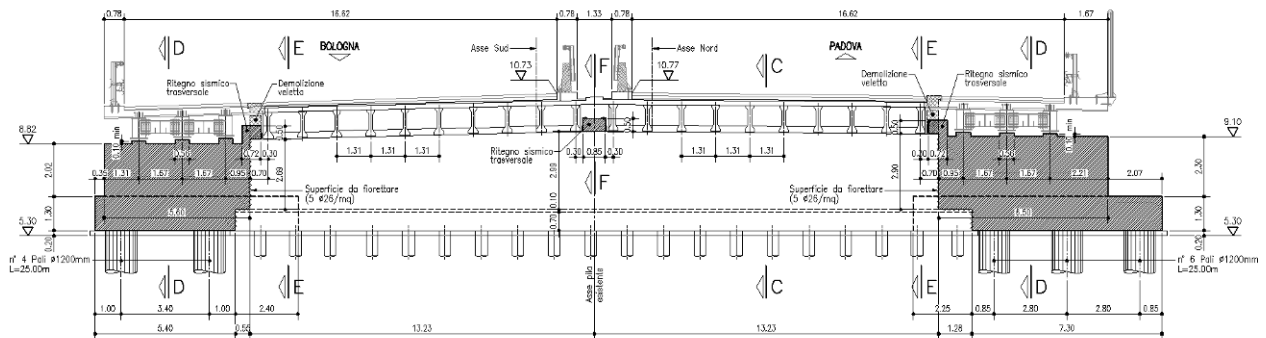
Figura 7-2 - Prospetto pila con notazione ritegni trasversali (campate centrali)
