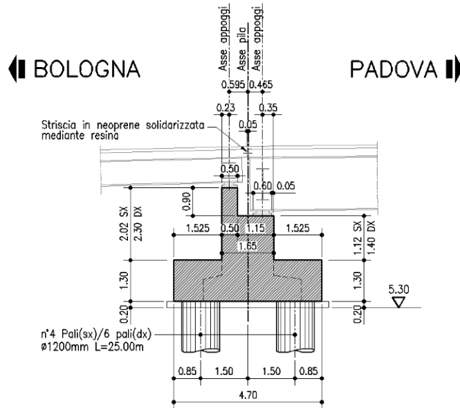
Figura 1-11 - Sezione trasversale pila in ampliamento
