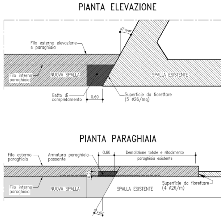
Figura 1-14 - Dettaglio connessione spalla esistente/in ampliamento
