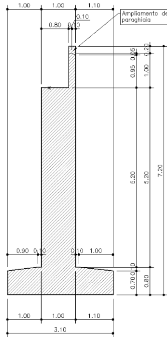
Figura 1-3 - Geometria di calcolo spalla esistente
