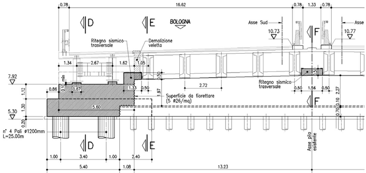
Figura 1-12 - Semi-prospetto pila esistente ed in ampliamento
