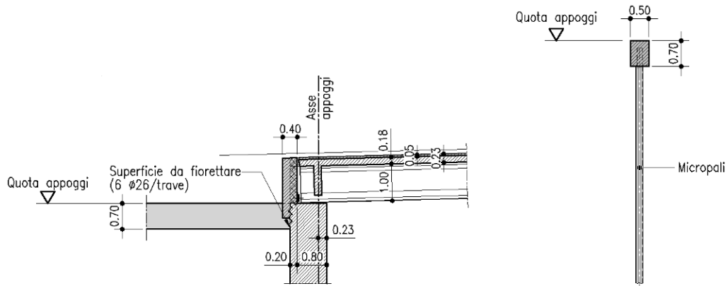
Figura 1-5 - Dettagli tiranti a tergo spalla
