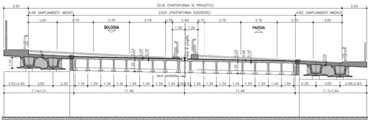
Sezioni trasversali allargate
