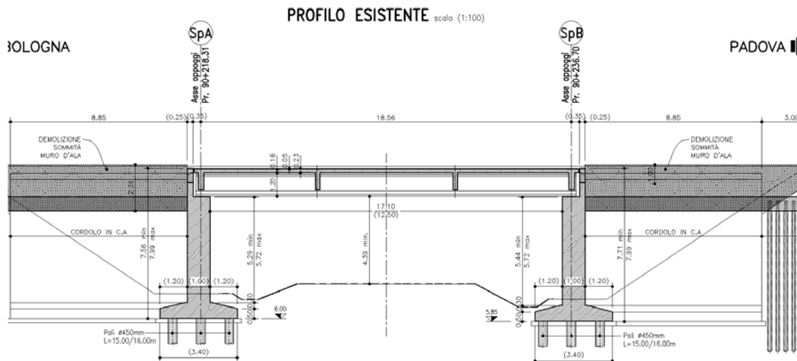
Profilo longitudinale impalcato esistente
