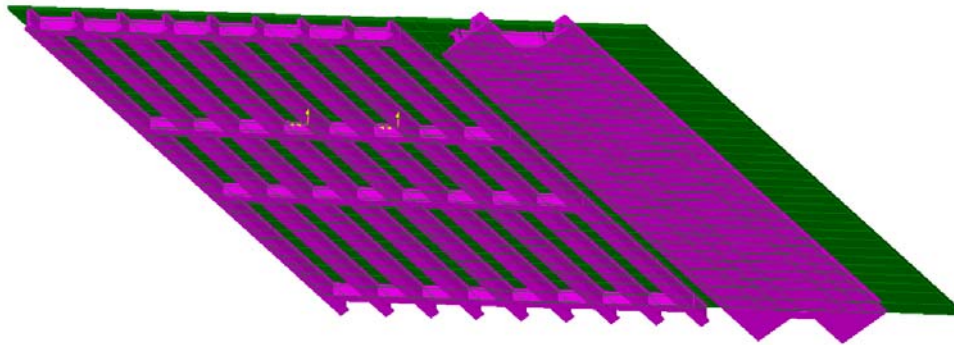
Modello agli E.F. – Campata centrale L calc = 18.20 m
