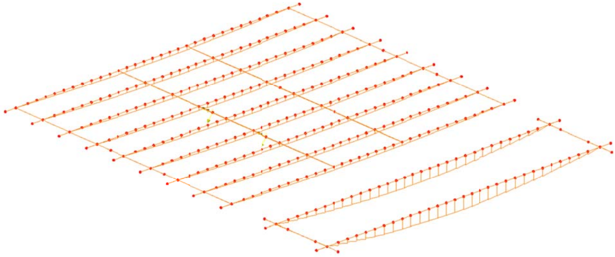
Max/Min Momento flettente - Travi principali e traversi
