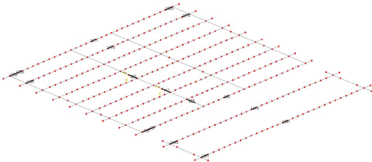
Elementi di verifica – Travi principali e traversi
