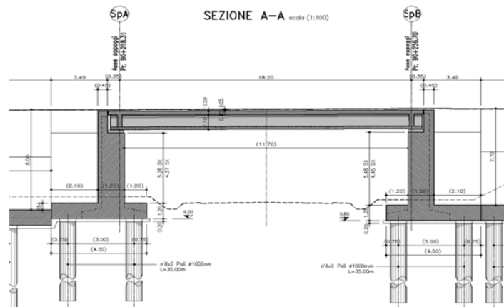
Profilo longitudinale impalcato nuovo
