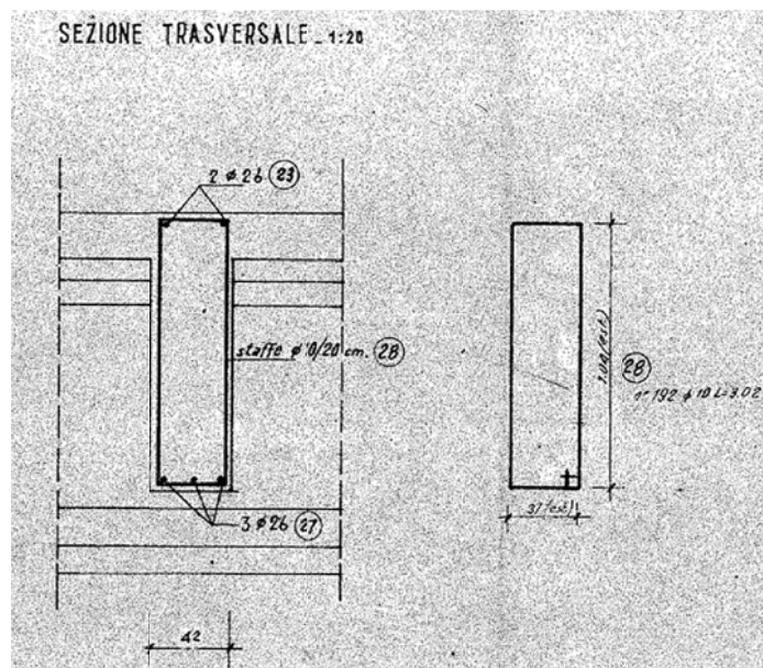
Traversi di campata
