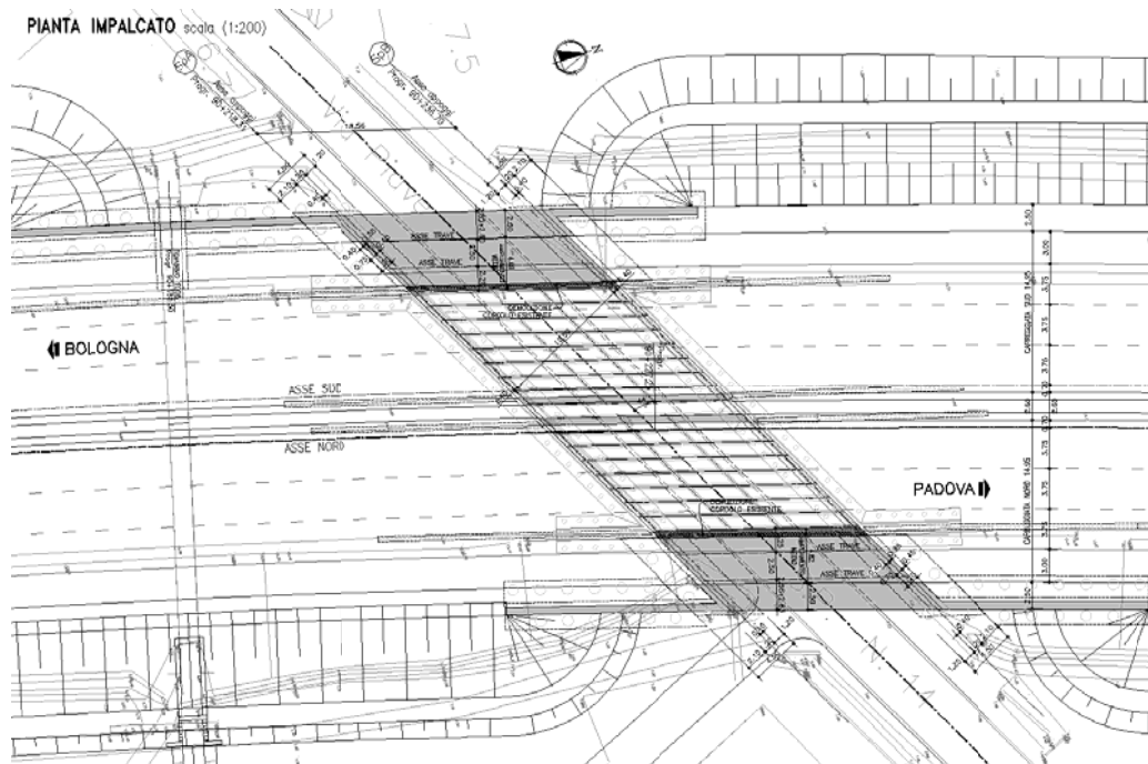
Pianta impalcato allargato
