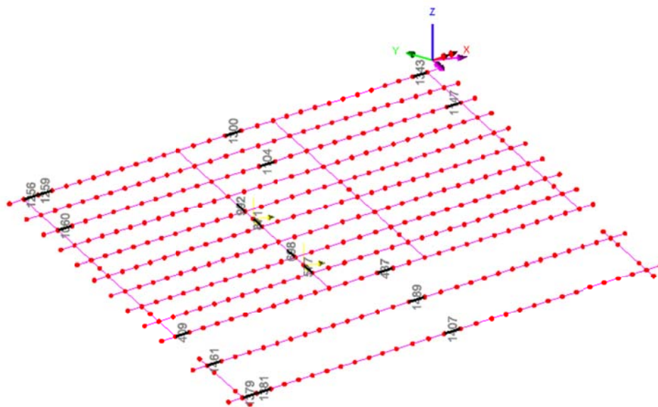
Elementi di verifica – Travi principali e traversi
