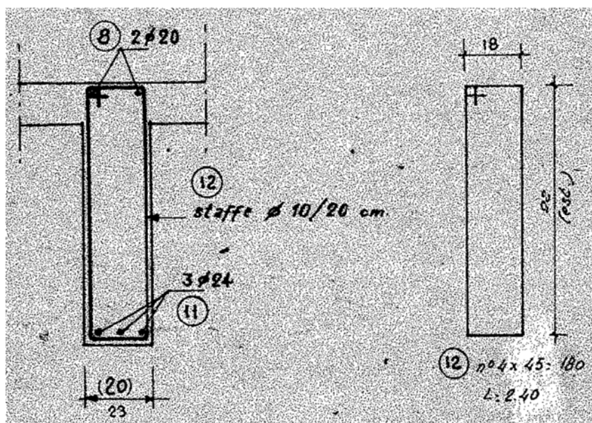
Traversi di campata
