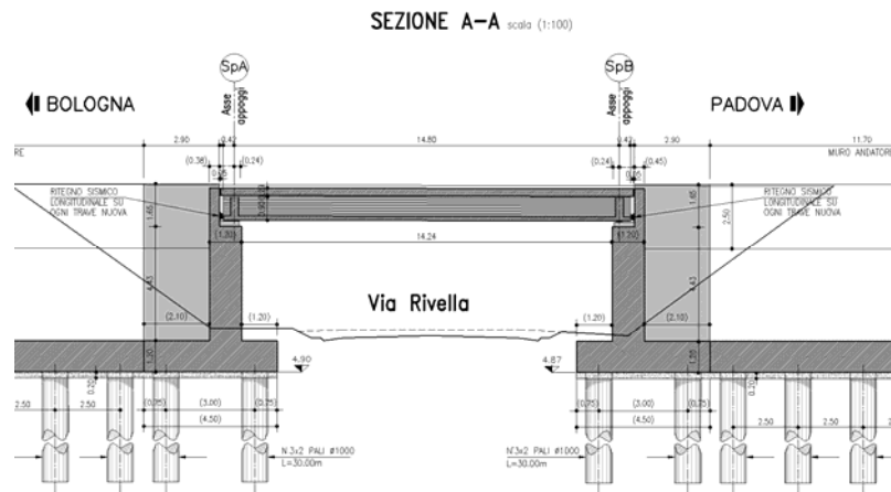
Profilo longitudinale impalcato nuovo
