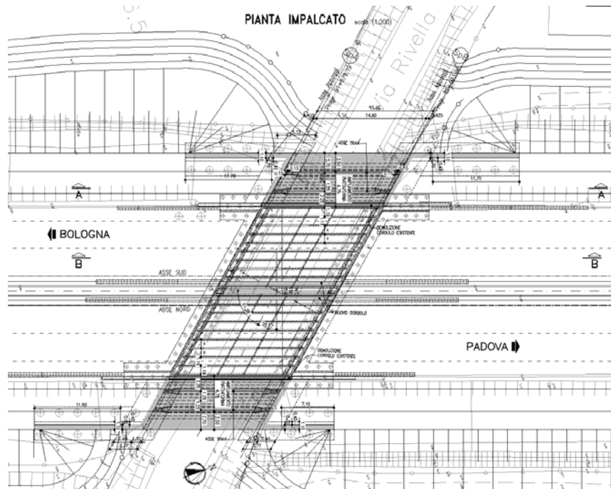
Pianta impalcato allargato
