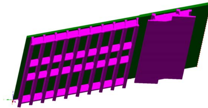
Modello agli E.F. – Campata centrale L_{calc} = 14.80\text{ m}
