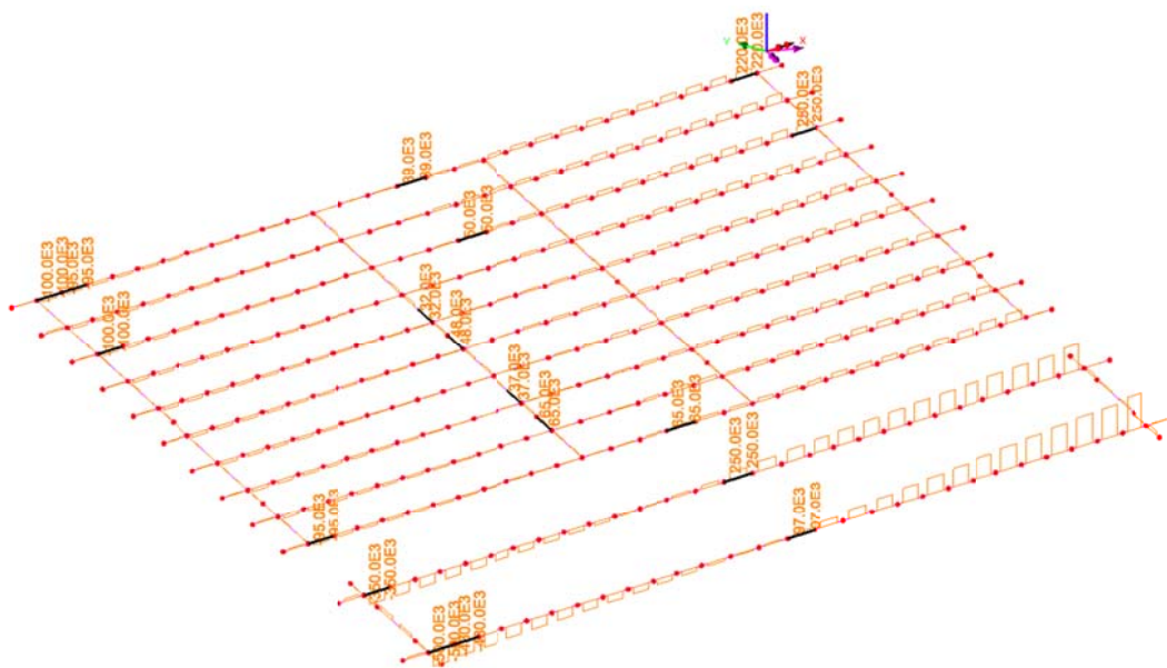
Max Taglio - Travi principali e traversi
