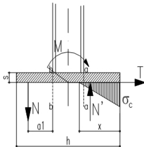
Figura 1-2 - Schematizzazione sollecitazioni alla base della piastra
