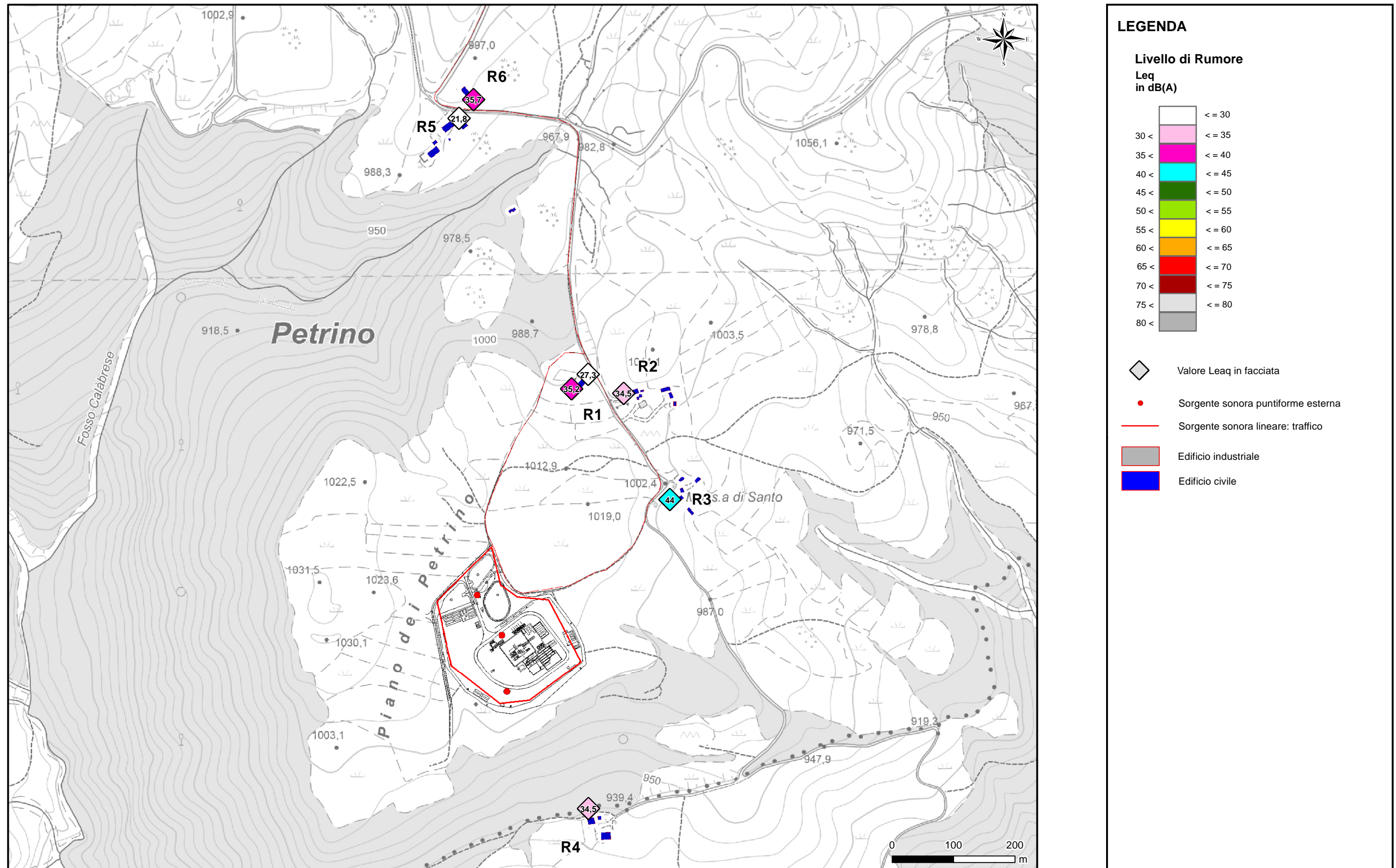
Figura 5.2.3.c Laeq massimo in facciata dei ricettori durante le attività di cantiere nel periodo diurno senza il contributo del traffico esterno
