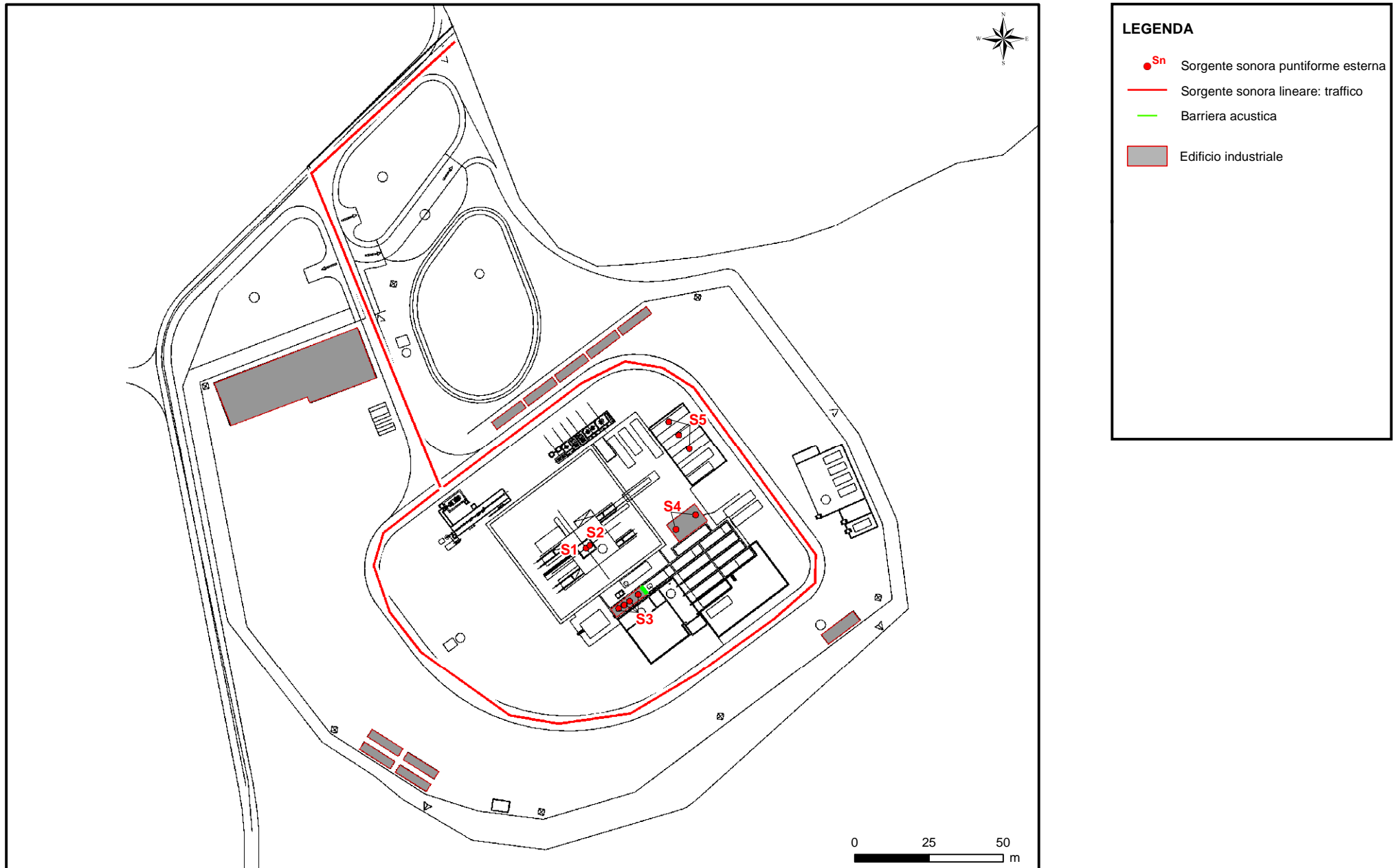
Figura 5.3.1.a Individuazione sorgenti sonore durante la fase di perforazione
