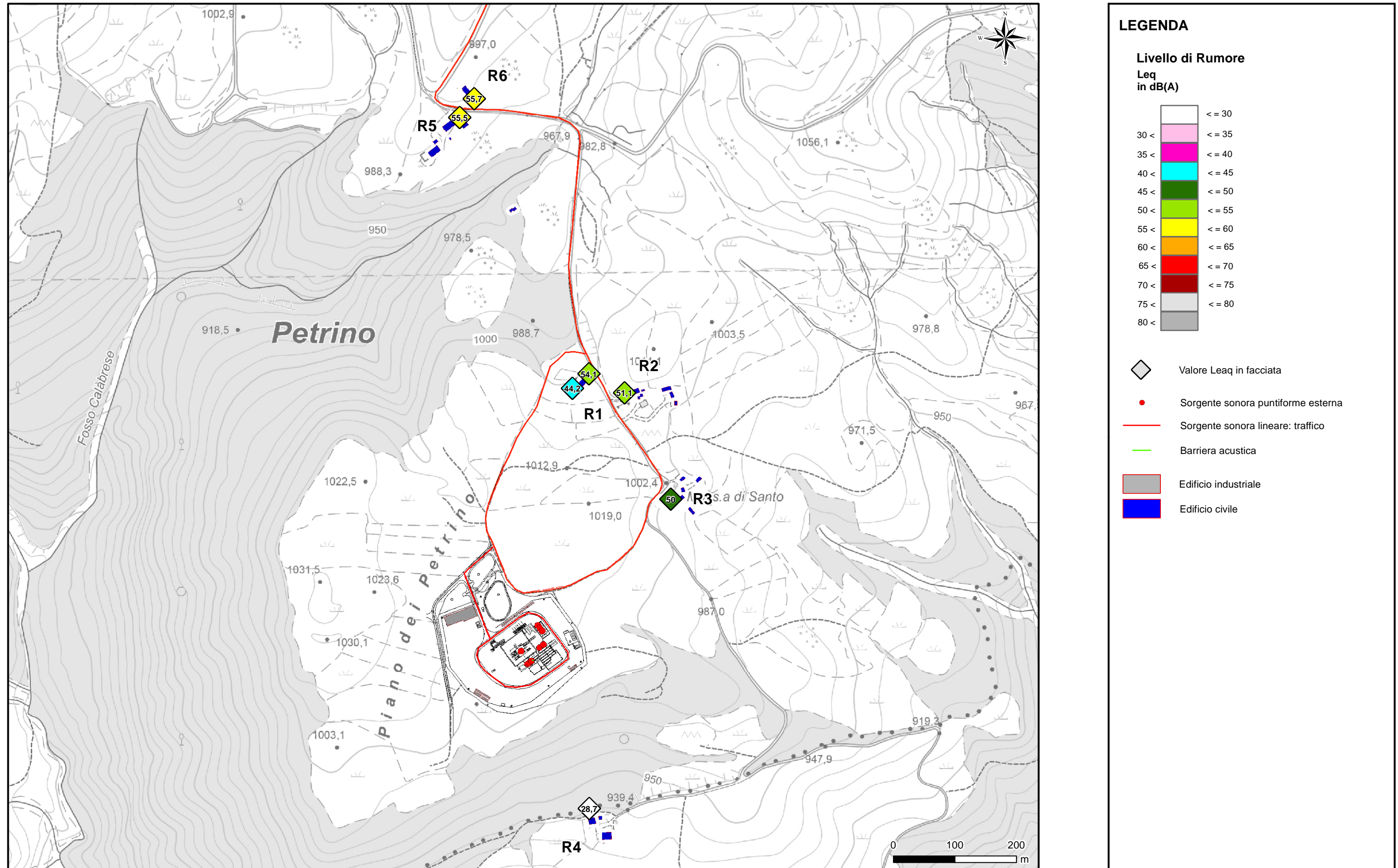
Figura 5.3.2.a Laeq massimo in facciata dei ricettori durante le attività di perforazione nel periodo diurno compreso il contributo del traffico esterno
