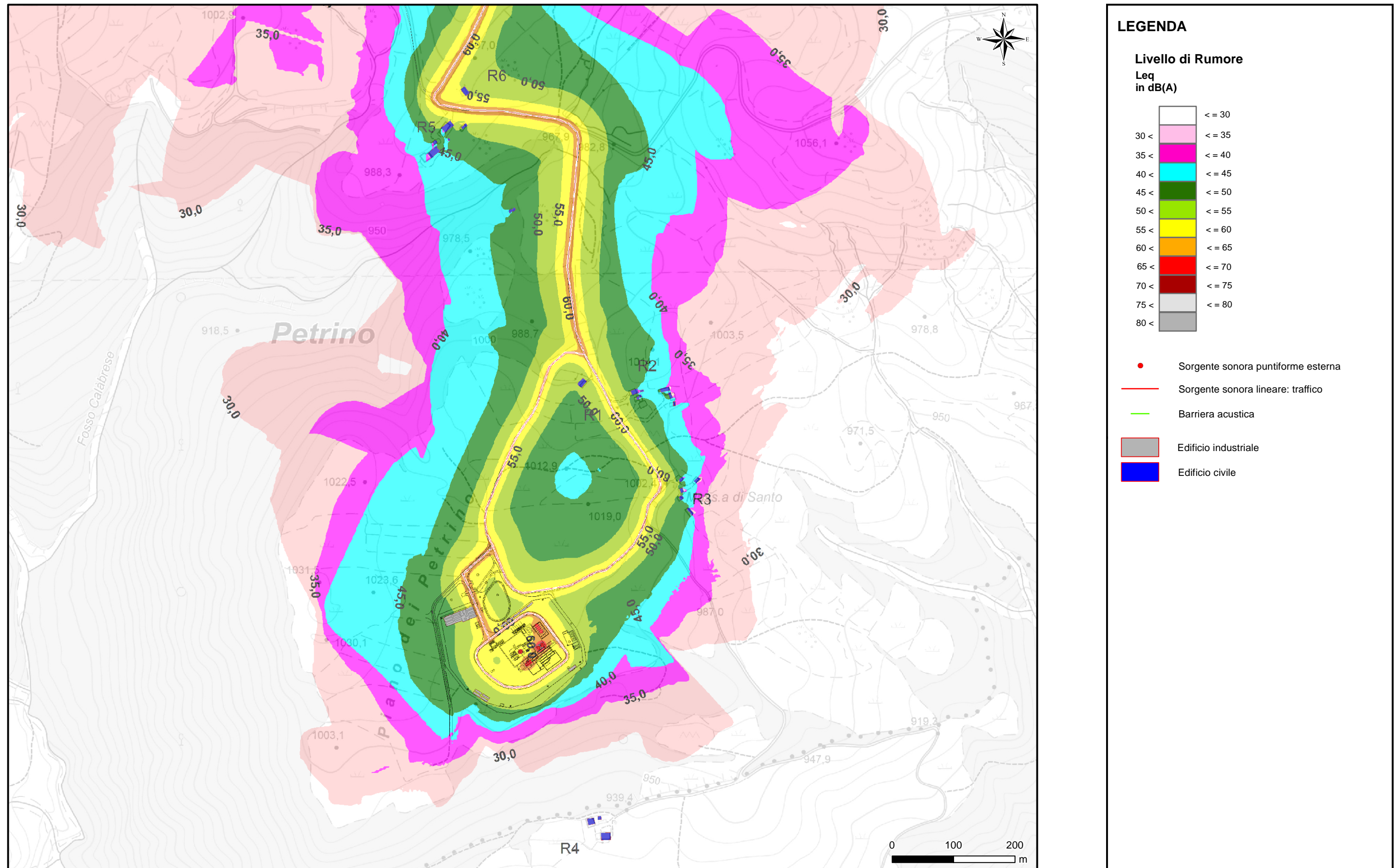
Figura 5.3.2.b Isofoniche durante le attività di perforazione nel periodo diurno compreso il contributo del traffico esterno
