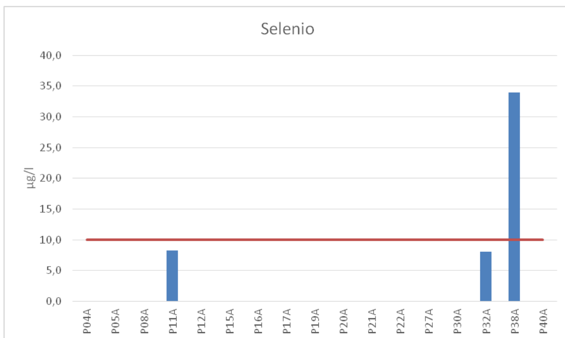
parametro Selenio – luglio/agosto 2016
