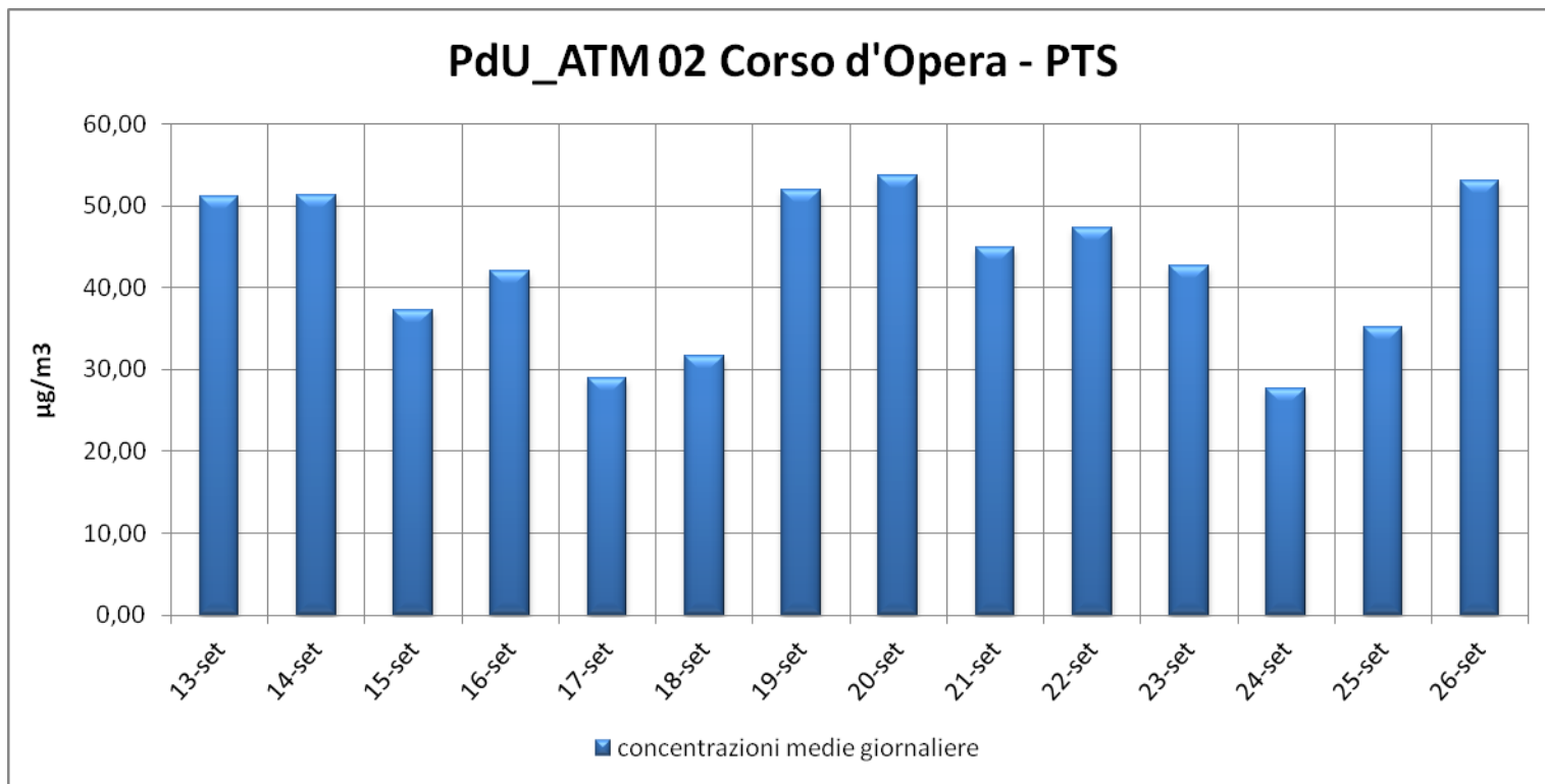
Polveri Totali Sospese (PTS): Trend delle concentrazioni medie giornaliere registrate per il punto PdU_ATM02 in Corso D'Opera
