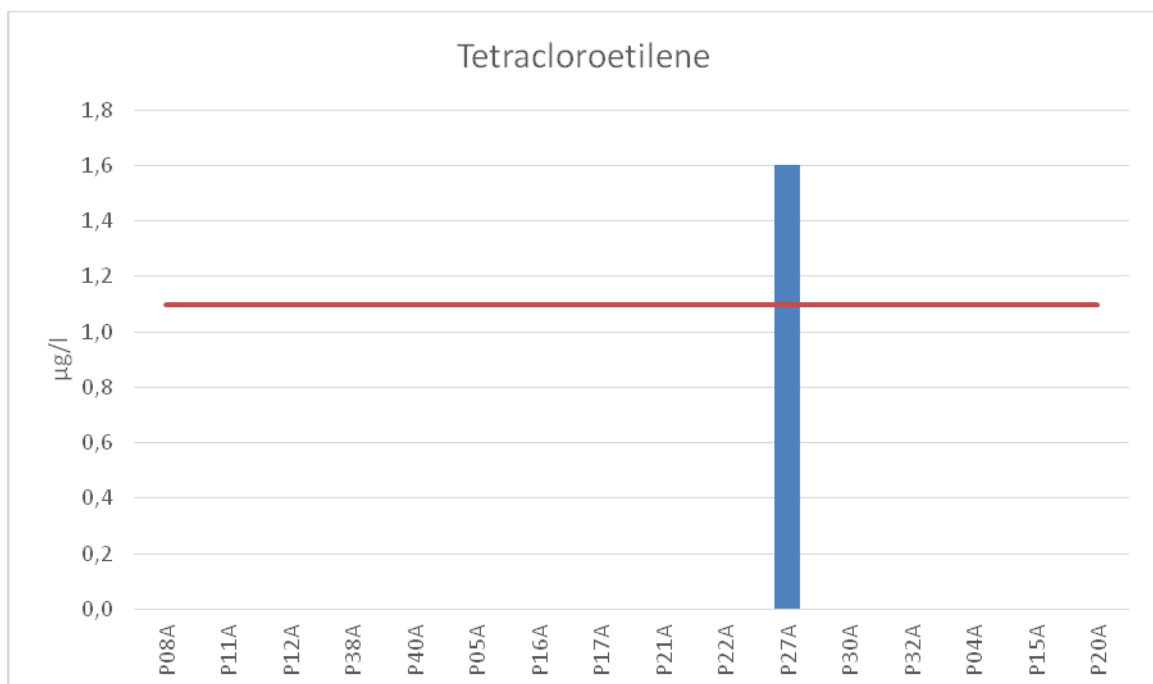
parametro Tetracloroetilene – ottobre 2016
