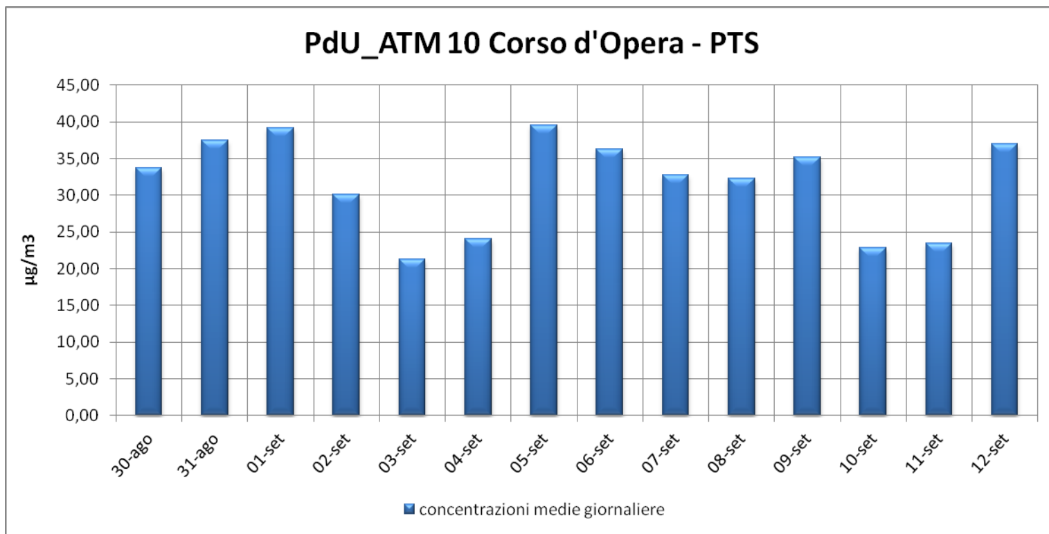
Polveri Totali Sospese (PTS): Trend delle concentrazioni medie giornaliere registrate per il punto PdU_ATM10 in Corso D'Opera
