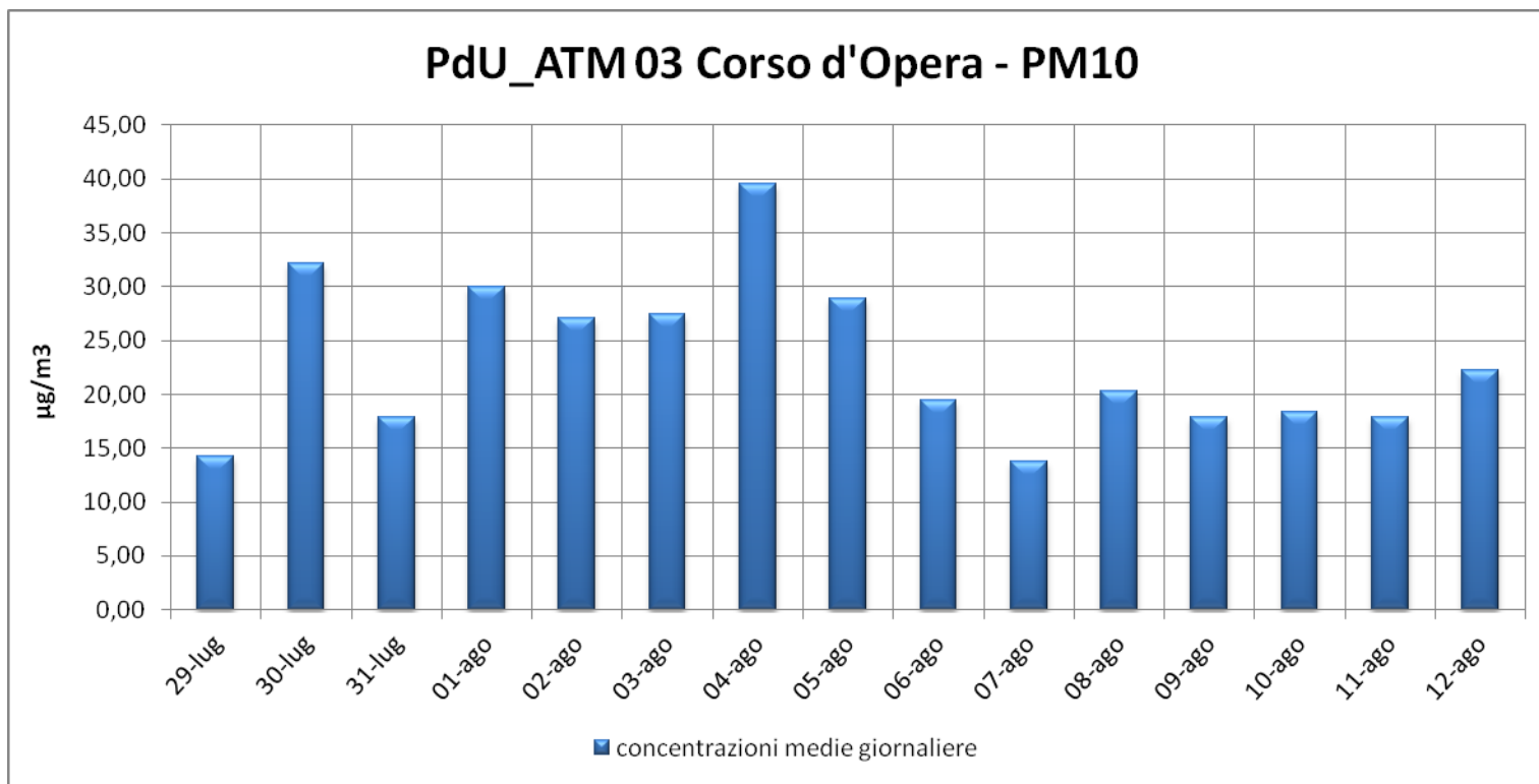
PM10: Trend delle concentrazioni medie giornaliere registrate per il punto PdU_ATM03 in Corso D'Opera
