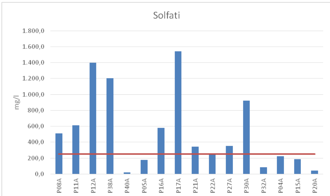
parametro Solfati – ottobre 2016
