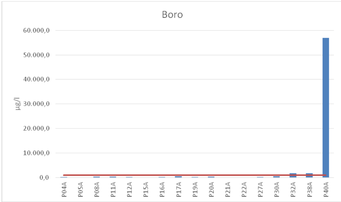
parametro Boro – luglio/agosto 2016
