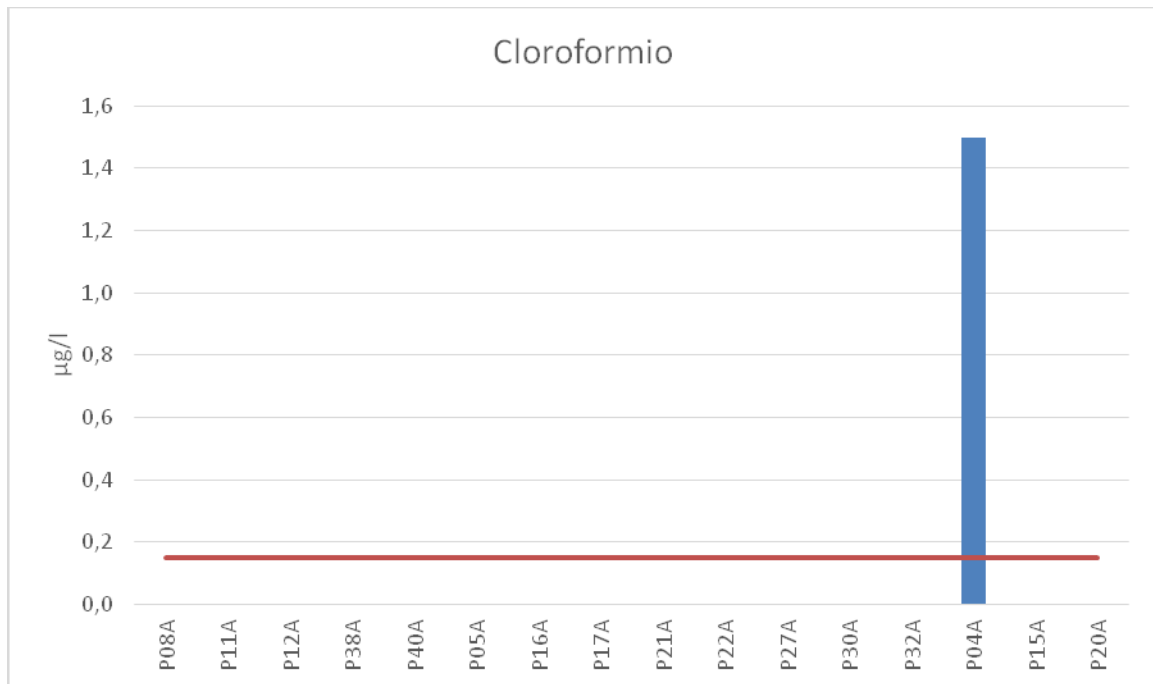
parametro Cloroformio – ottobre 2016
