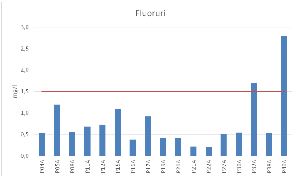
parametro Fluoruri – luglio/agosto 2016
