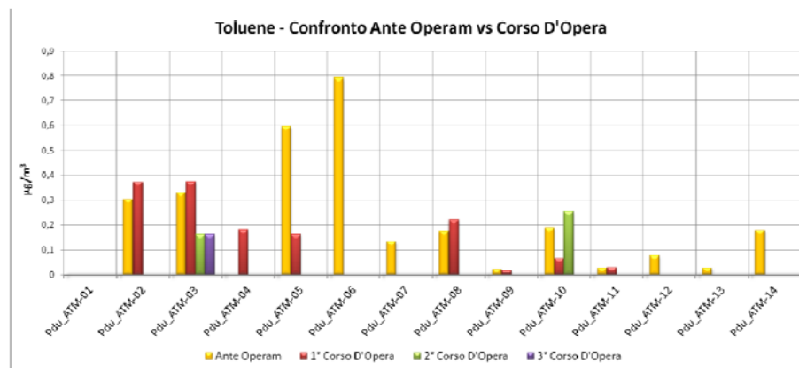
Inquinanti gassosi: Trend delle concentrazioni medie giornaliere rilevate- confronto Ante e Corso D'Opera
