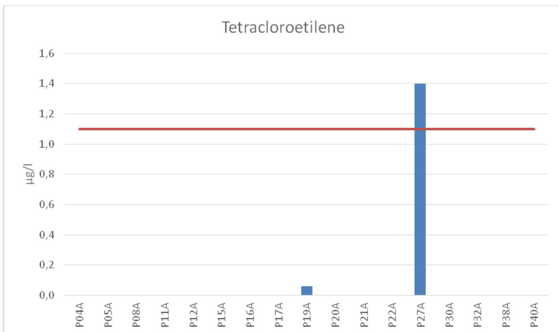
parametro Tetracloroetilene - luglio/agosto 2016
