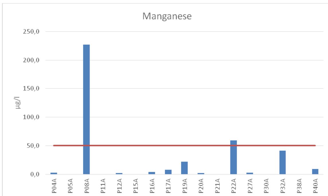
parametro Manganese – luglio/agosto 2016
