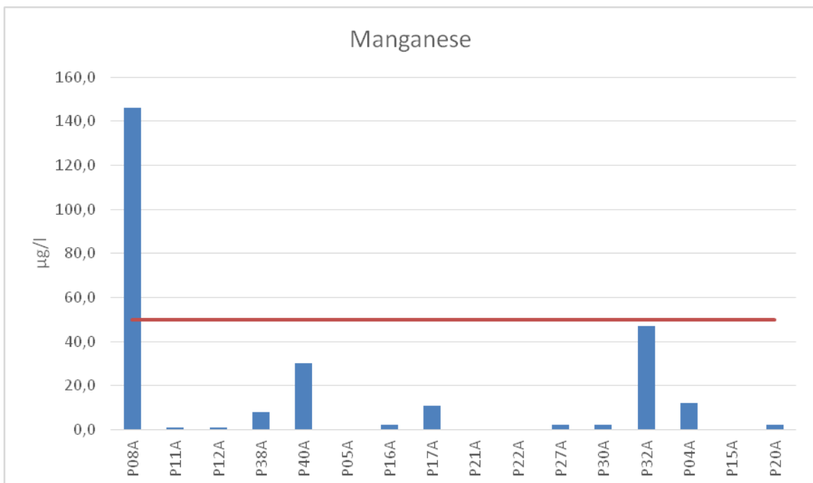
parametro Manganese – ottobre 2016
