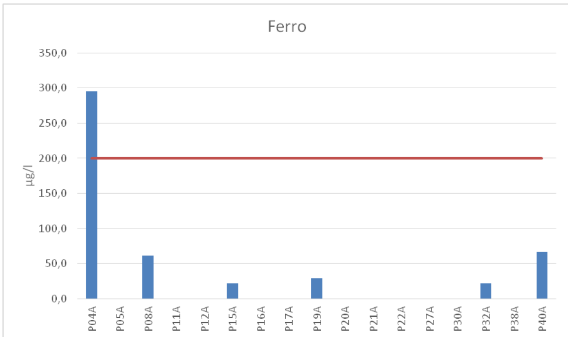
parametro Ferro – luglio/agosto 2016
