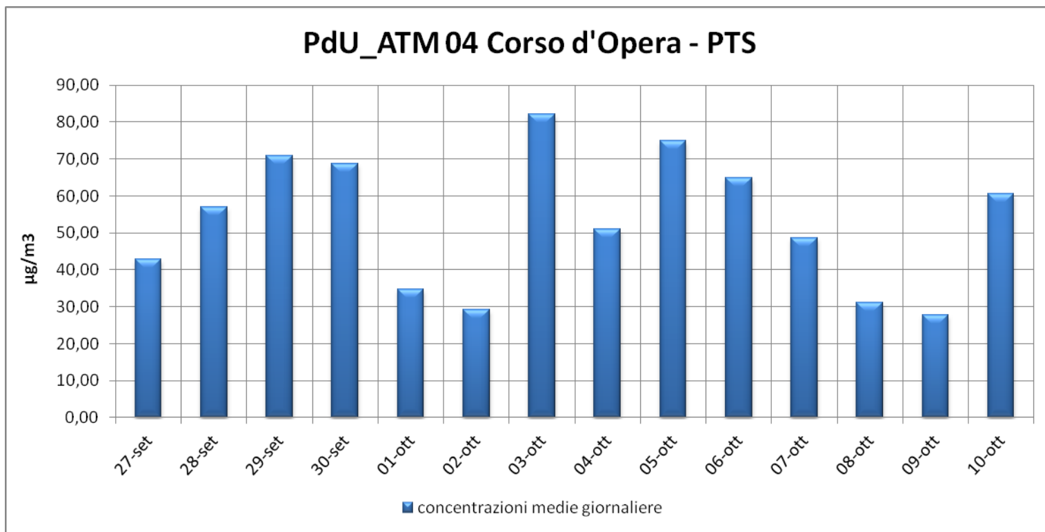
Polveri Totali Sospese (PTS): Trend delle concentrazioni medie giornaliere registrate per il punto PdU_ATM04 in Corso D'Opera
