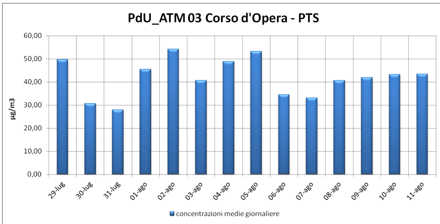
Polveri Totali Sospese (PTS): Trend delle concentrazioni medie giornaliere registrate per il punto PdU_ATM03 in Corso D'Opera
