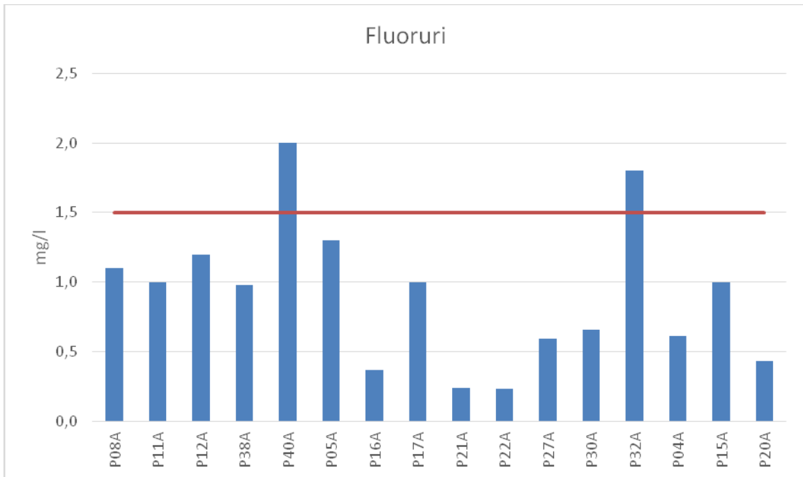
parametro Fluoruri – ottobre 2016
