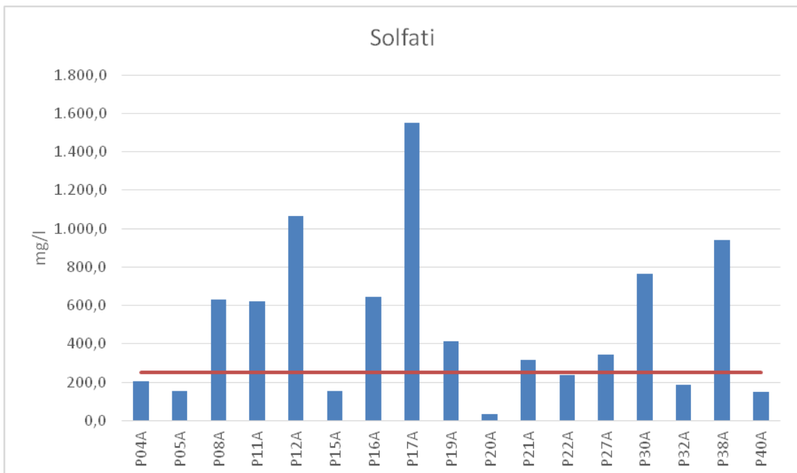
parametro Solfati – luglio/agosto 2016
