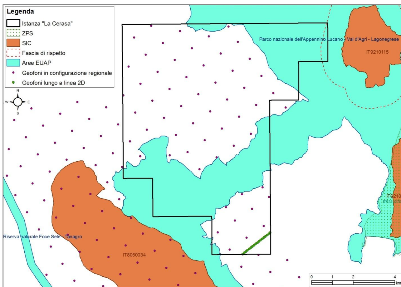
Figura 3.2 - Ubicazione dei geofoni all'interno dell'area in istanza di permesso di ricerca "La Cerasa", sia in configurazione regionale che lungo la linea 2D (fonte dei dati: Shell)
