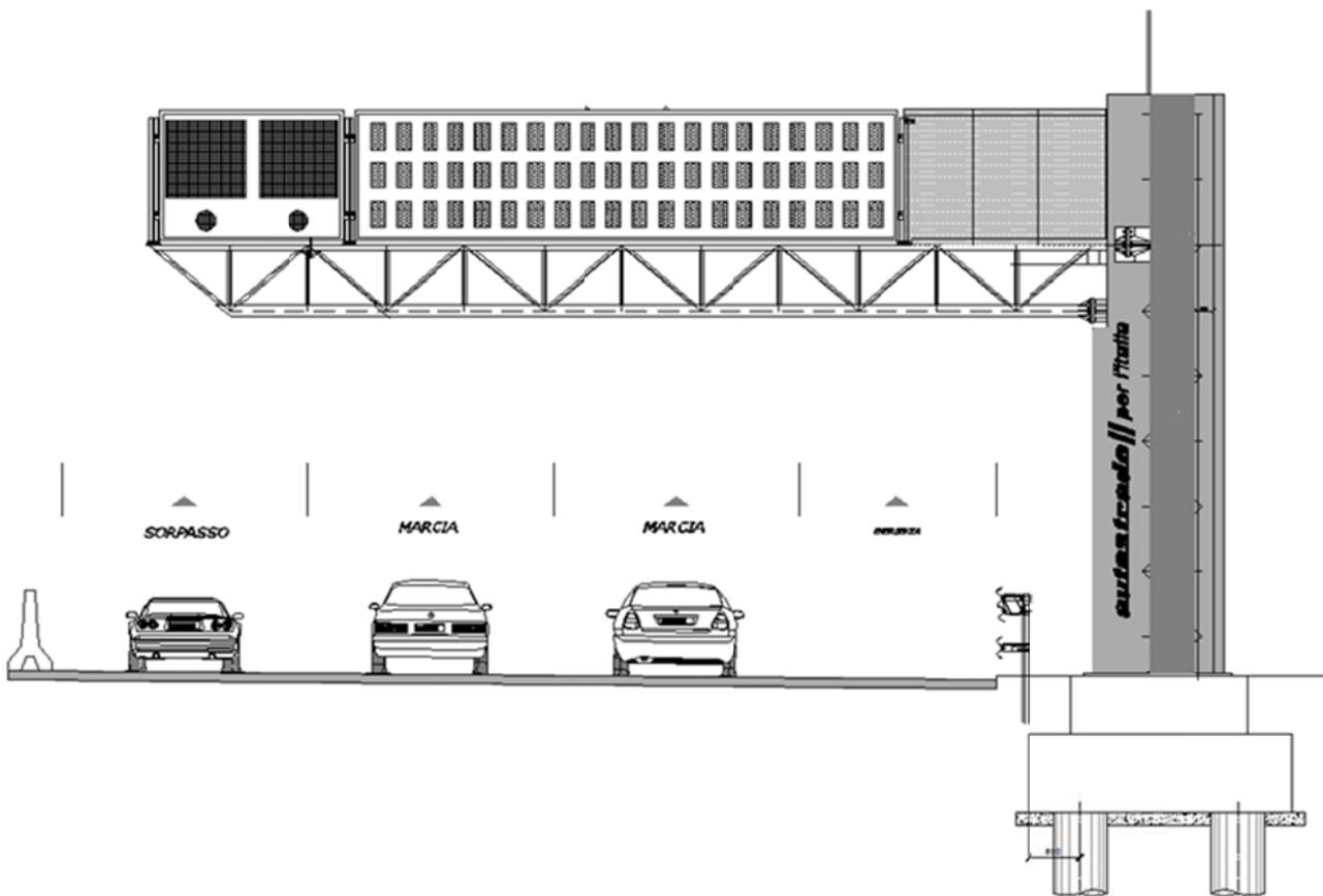
Fig. 1 – Prospetto frontale
