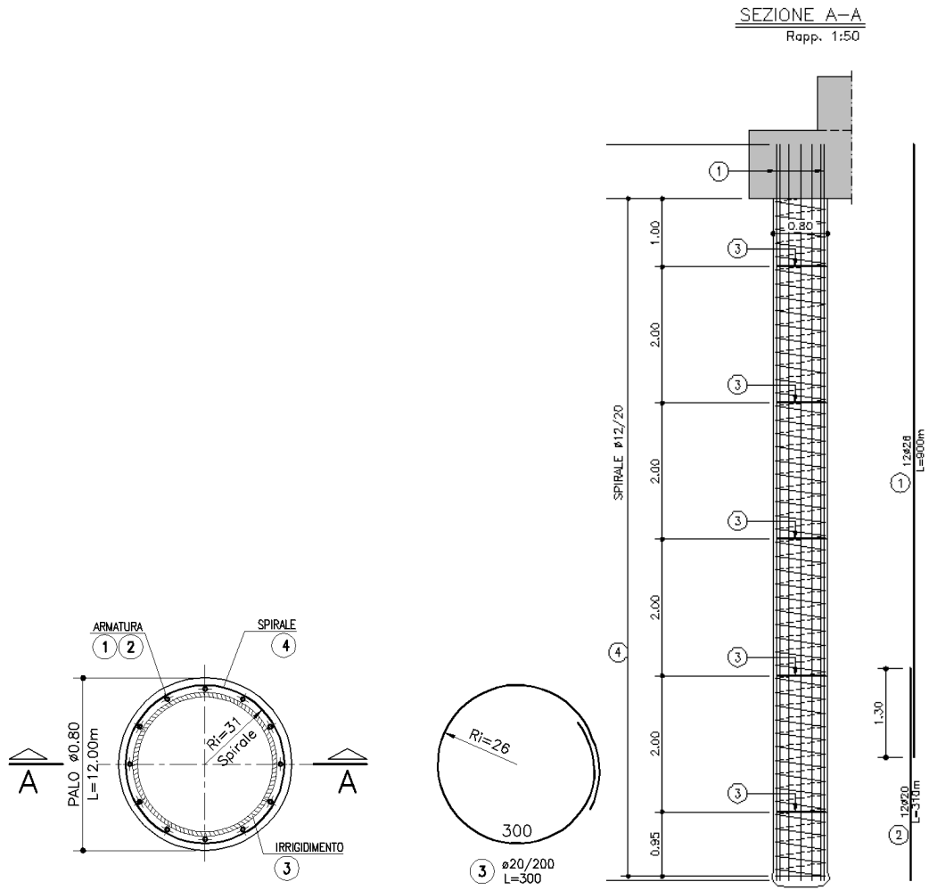
Figura 41: Verifica SLU
