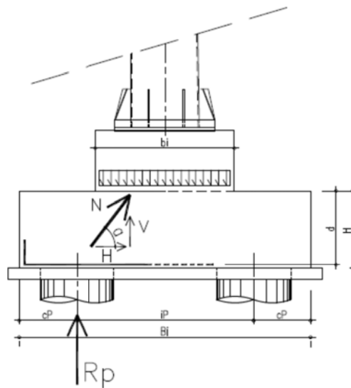
Figura 42: Meccanismo resistente a Tirante-puntone
