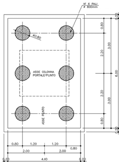
Figura 40: Sezione del plinto di fondazione
