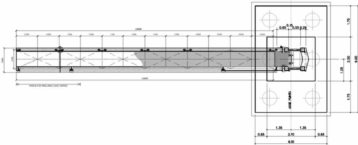
Figura 38: Plinto di fondazione vista in pianta
