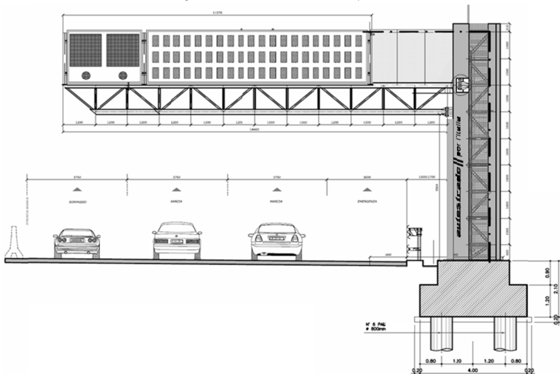
Figura 39: Plinto di fondazione vista prospettica
