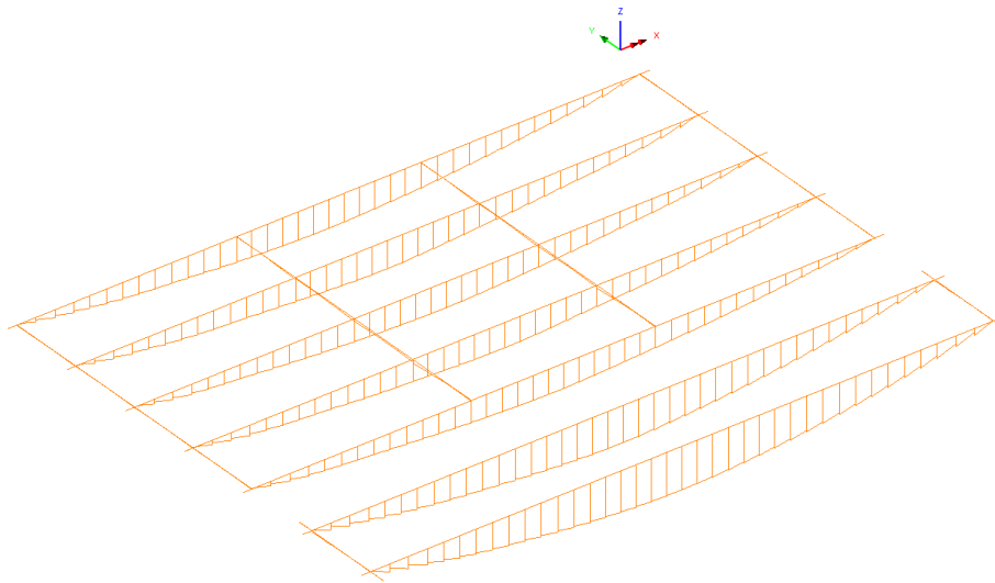
Max/Min Momento flettente - Travi principali e traversi
