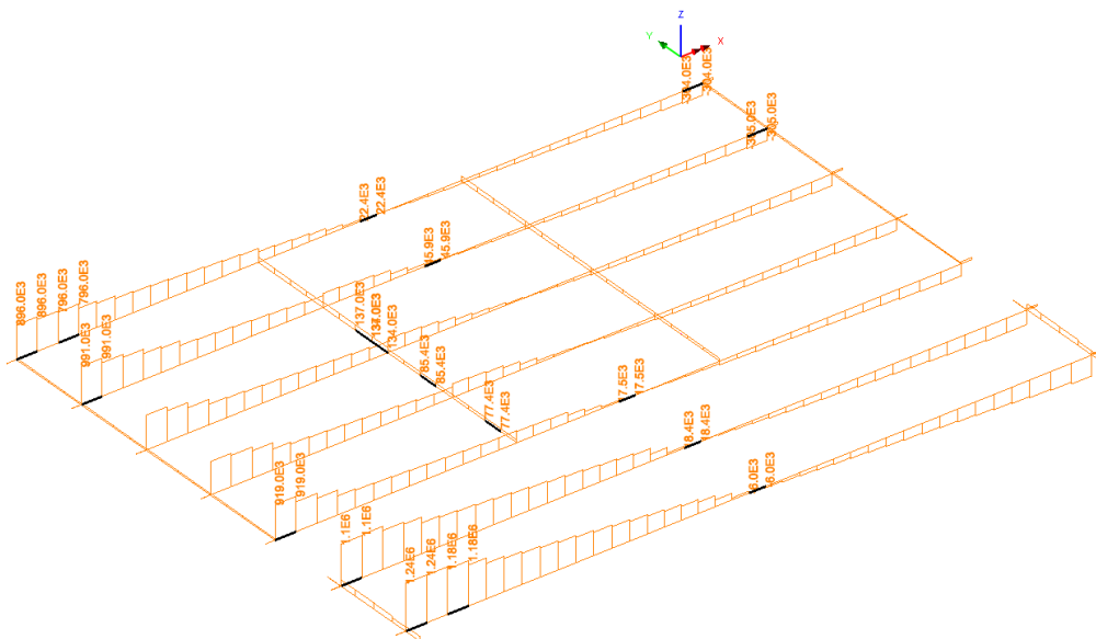
Max Taglio - Travi principali e traversi
