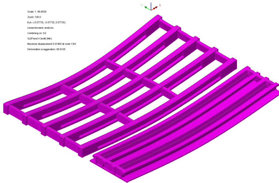
Deformata verticale massima di Fase 3 - Travi principali e trasversi
