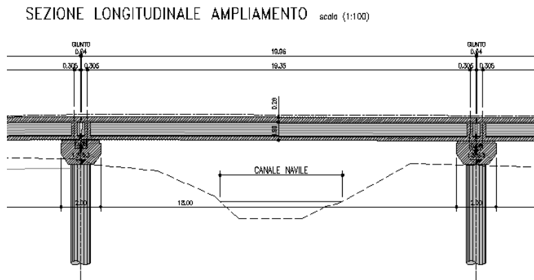
Profilo longitudinale impalcato nuovo
