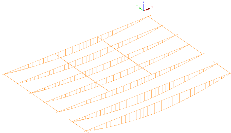
Max/Min Momento flettente - Travi principali e traversi
