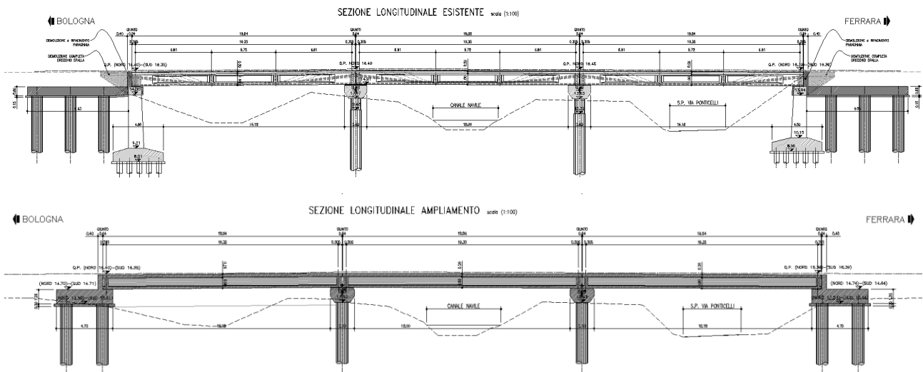
Sezioni longitudinali
