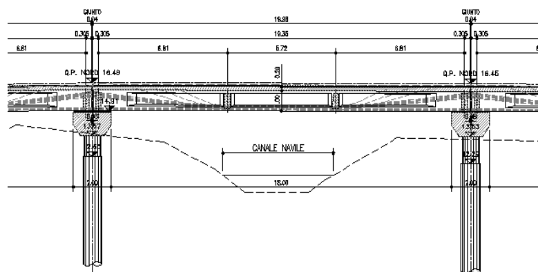
Profilo longitudinale impalcato esistente
