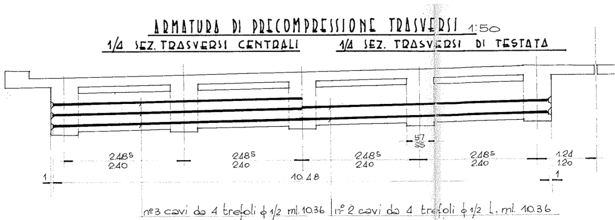
Traversi di campata
