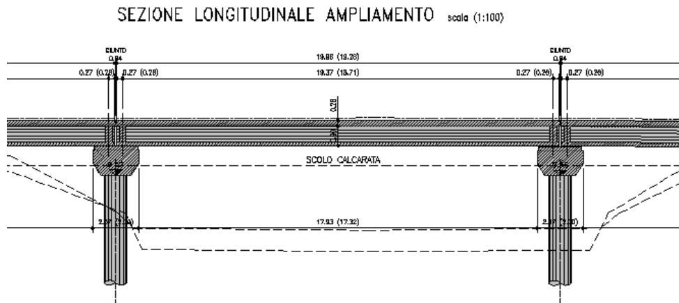
Profilo longitudinale impalcato nuovo
