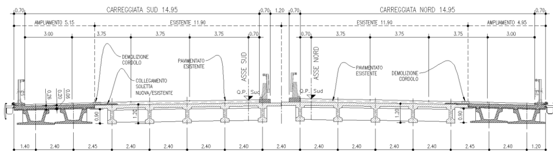
Sezioni trasversali allargate
