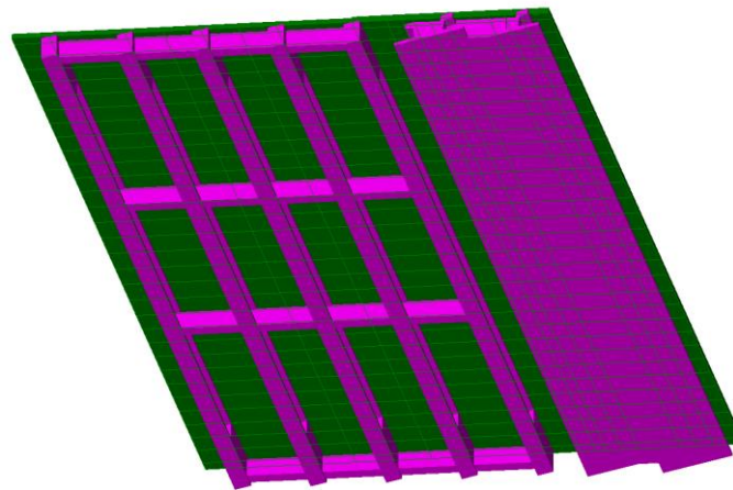
Modello agli E.F. – Campata unica L calc = 19.37 m
