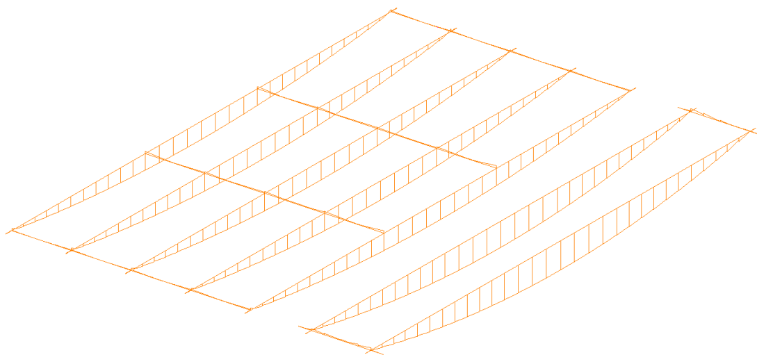
Max/Min Momento flettente - Travi principali e traversi
