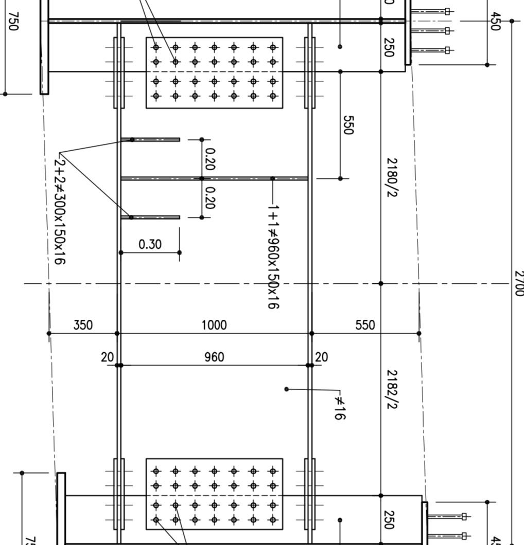
1/2 SEZIONE TRASVERSO DI TESTATA
