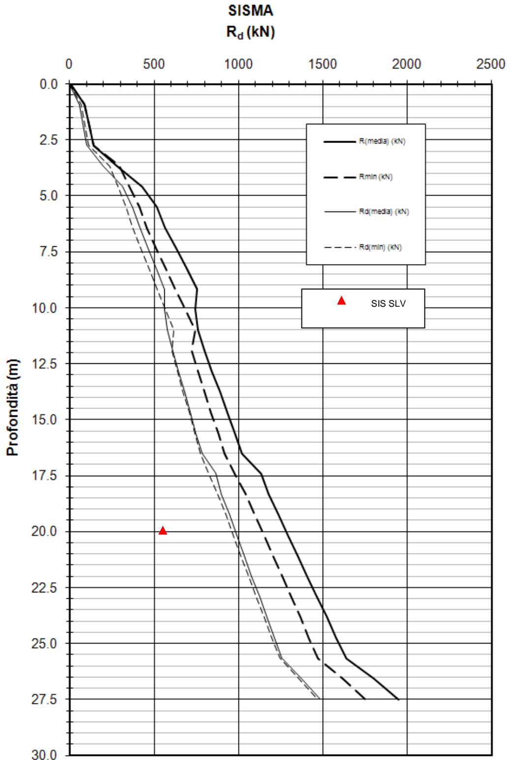
Figura 10-11: Pali esistenti - Azioni assiali massime a confronto con le resistenze di progetto Rd per i pali esistenti soggetti a compressione – combinazione SLV
