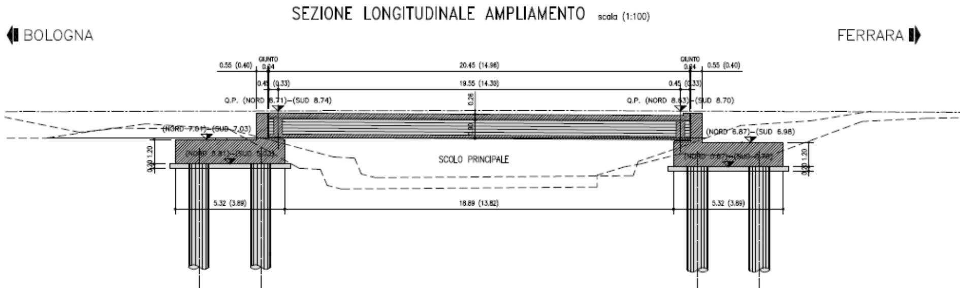
Figura 7-3: Sezione di progetto
