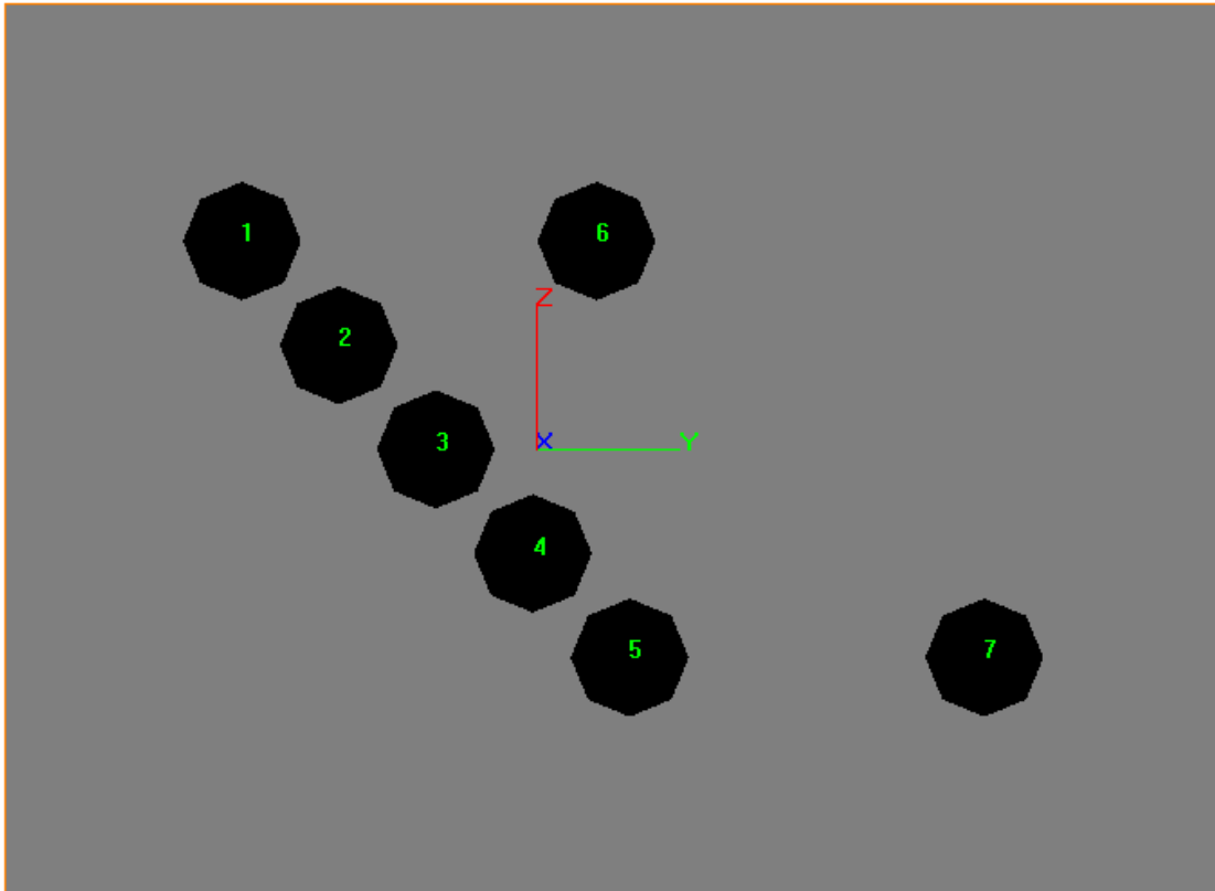
Figura 10-9: Schema Group della palificata - ampliamento fondazione su pali trivellati
