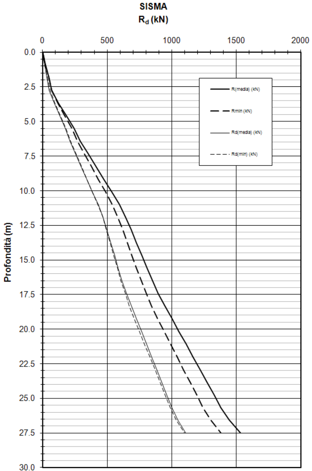
Figura 10-4: Pali esistenti - Resistenza del palo a trazione – combinazione SLV
