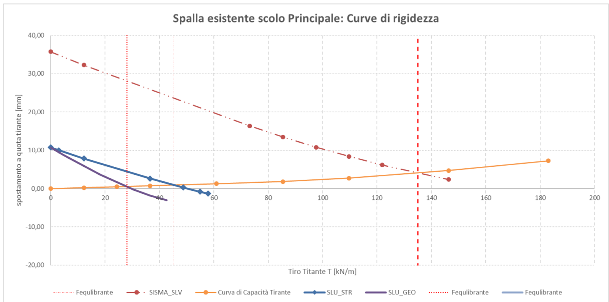
Figura 6-1. Curva di interazione tra spalla e micropali passivi – comportamento fondazione spalla lineare
