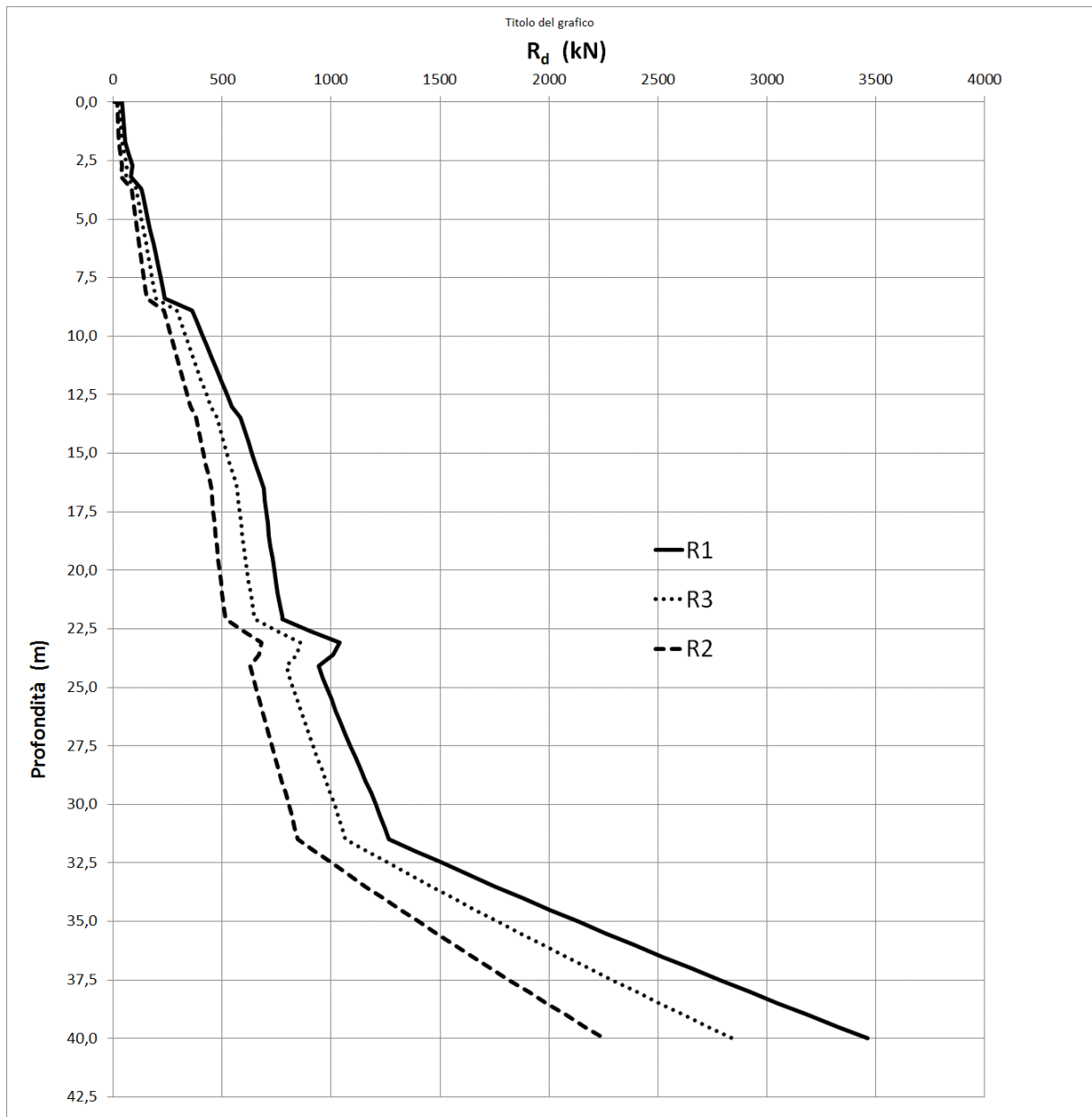
Figura 10-5: Pali trivellati - Resistenza del palo a compressione – combinazione SLU-SLV
