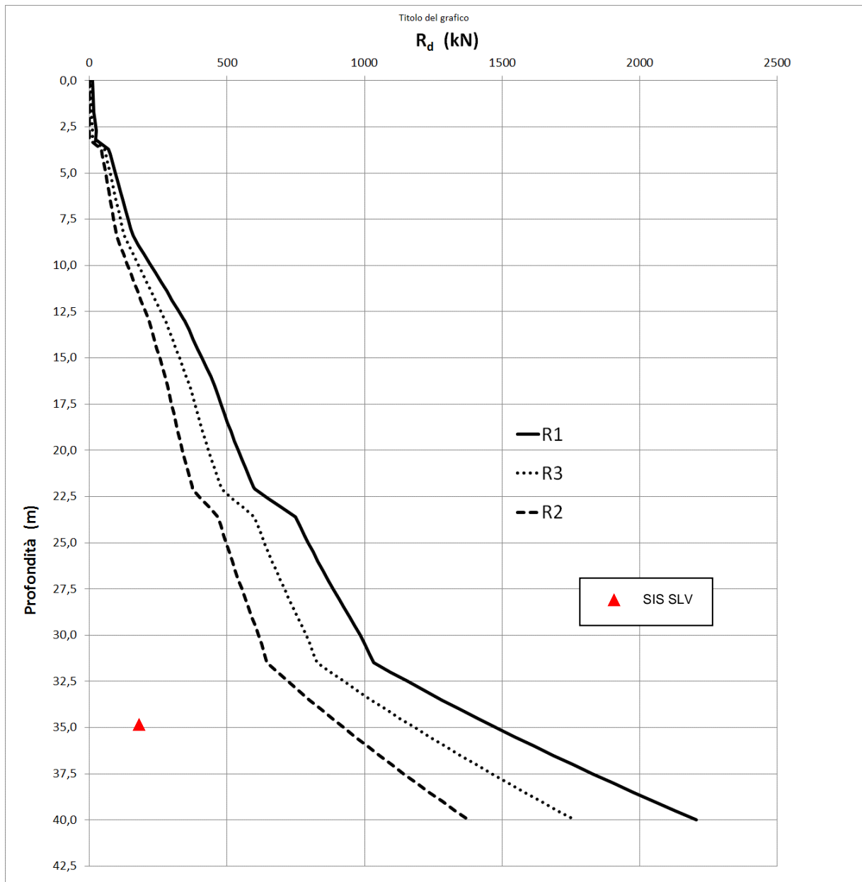
Figura 10-13: Azioni assiali massime a confronto con le resistenze di progetto R_d per i pali trivellati soggetti a trazione – combinazione SLU-SIS
