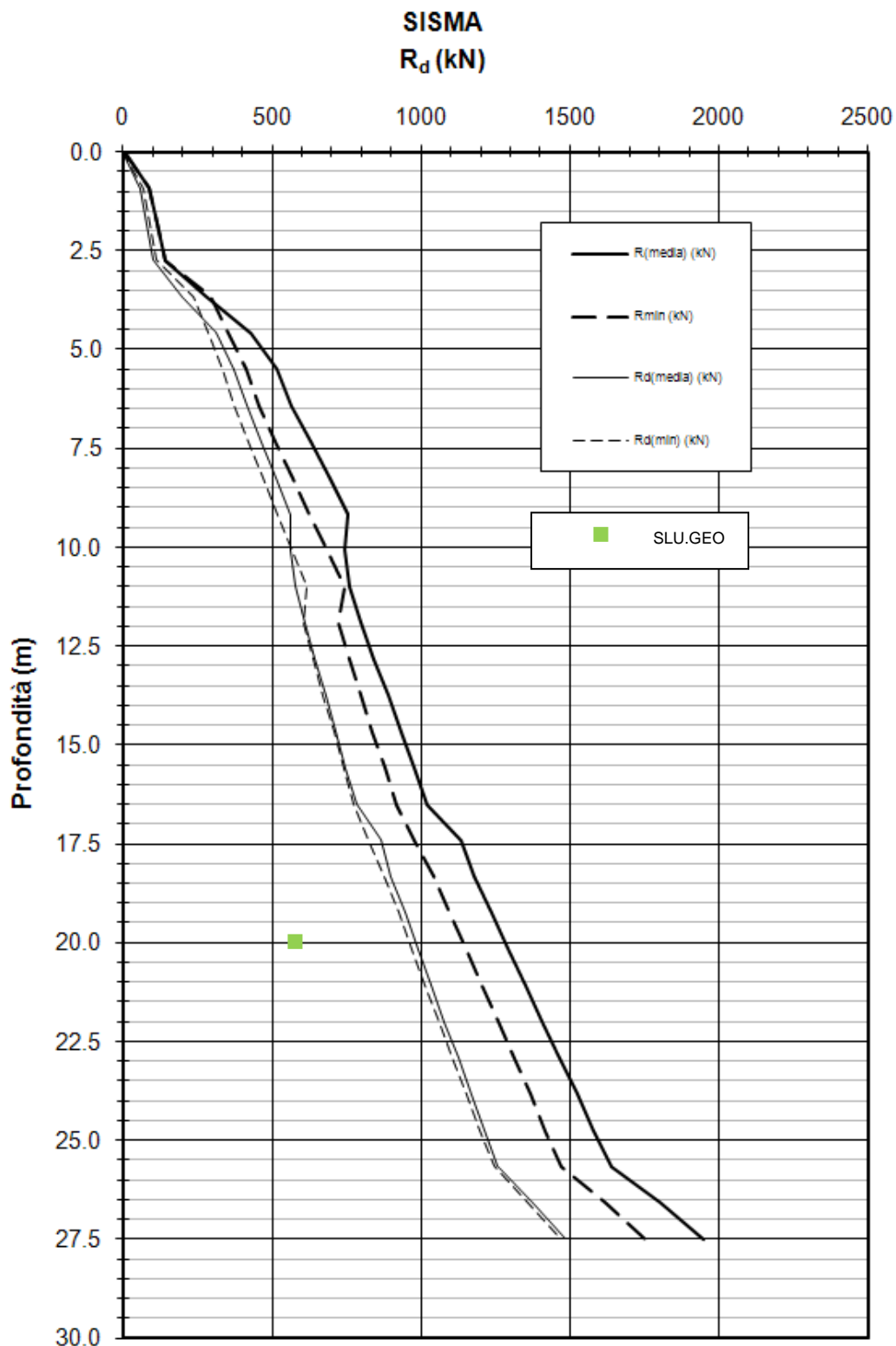
Figura 10-10: Azioni assiali massime a confronto con le resistenze di progetto R d per i pali esistenti soggetti a compressione – combinazione SLU
