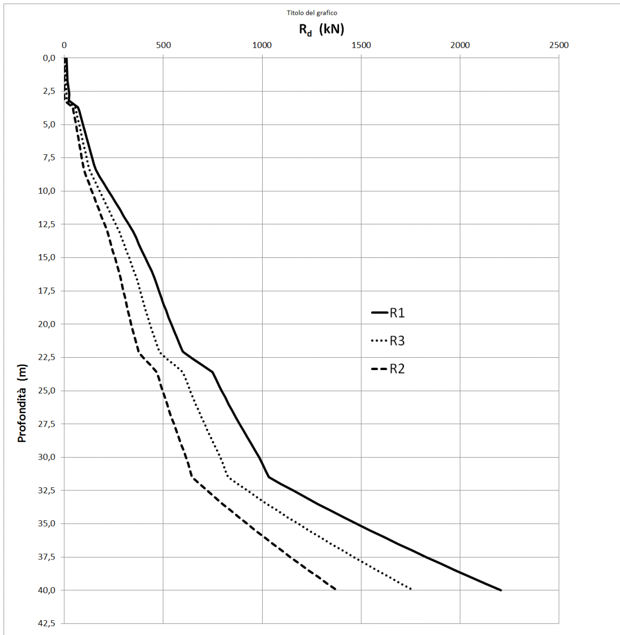
Figura 10-6: Pali trivellati - Resistenza del palo a trazione – combinazione SLU-SLV
