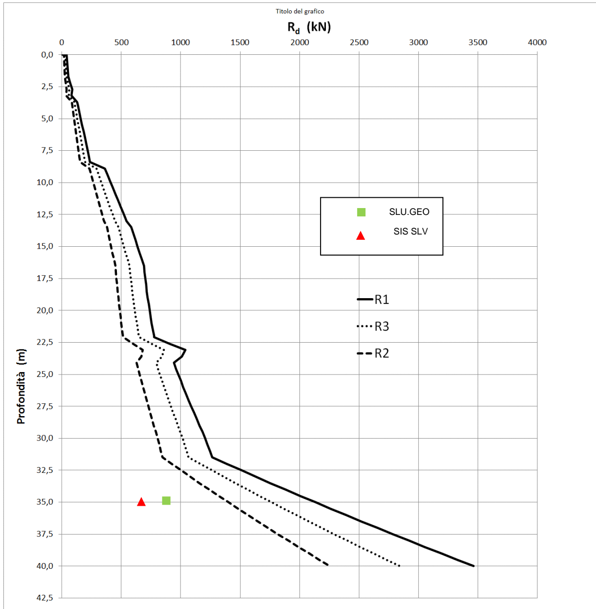
Figura 10-12: Azioni assiali massime a confronto con le resistenze di progetto R_d per i pali trivellati soggetti a compressione – combinazione SLU - SIS
