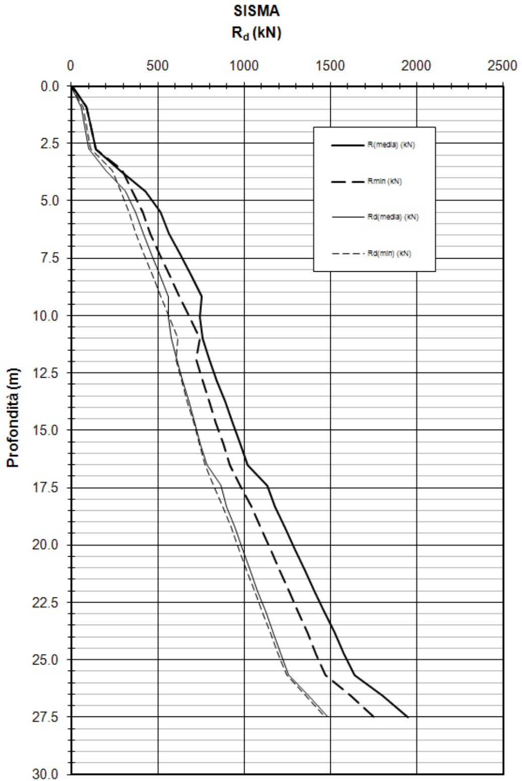
Figura 10-2: Pali esistenti - Resistenza del palo a compressione – combinazione SLV
