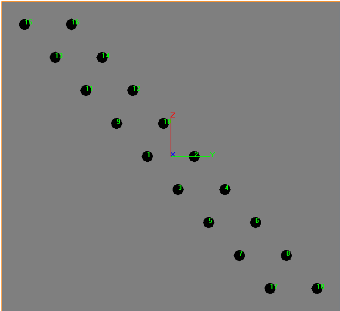
Figura 10-8: Schema Group della palificata - fondazione esistente
